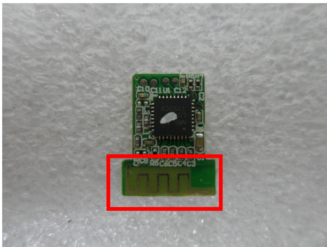
Antenna
