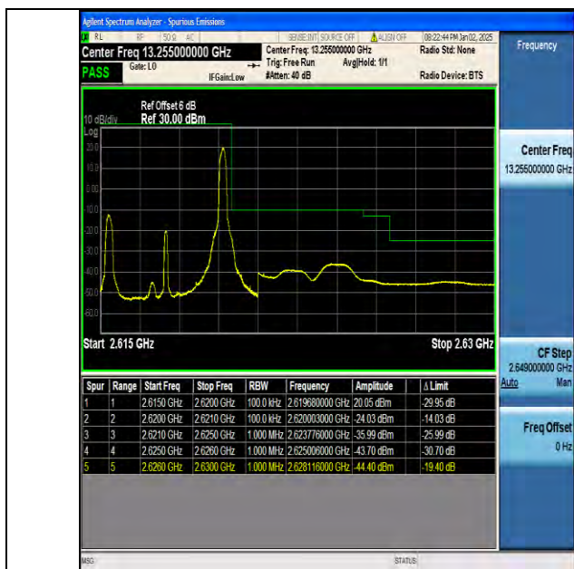
Band38 5MHz QPSK 38225 1RB#24
