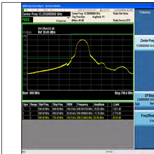
Band12 1.4MHz QPSK 23017 1RB#0
