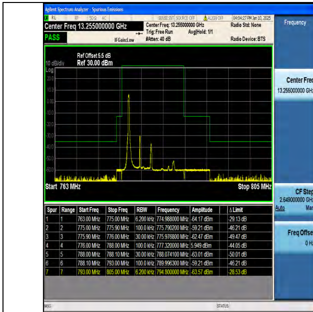
Band13 5MHz QPSK 23205 1RB#0
