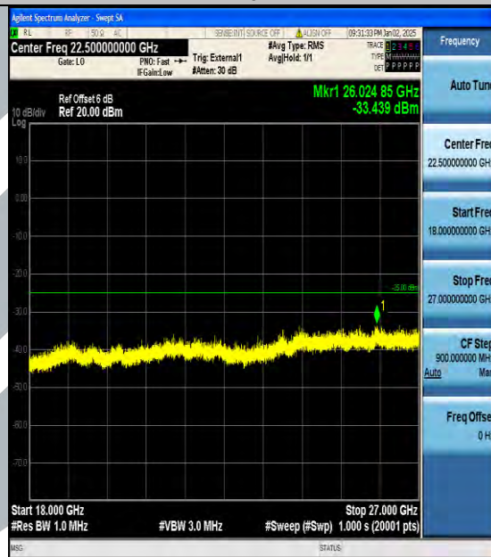
Band38_15MHz_QPSK_38000_1RB#0_18000~27000_18000~27000
