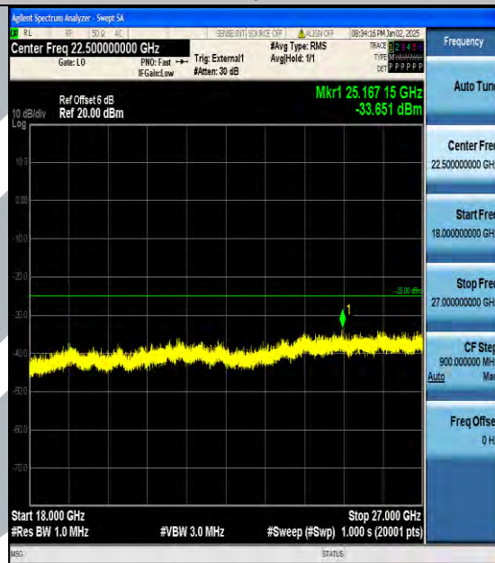
Band38_5MHz_16QAM_38000_1RB#0_18000~27000_18000~27000
