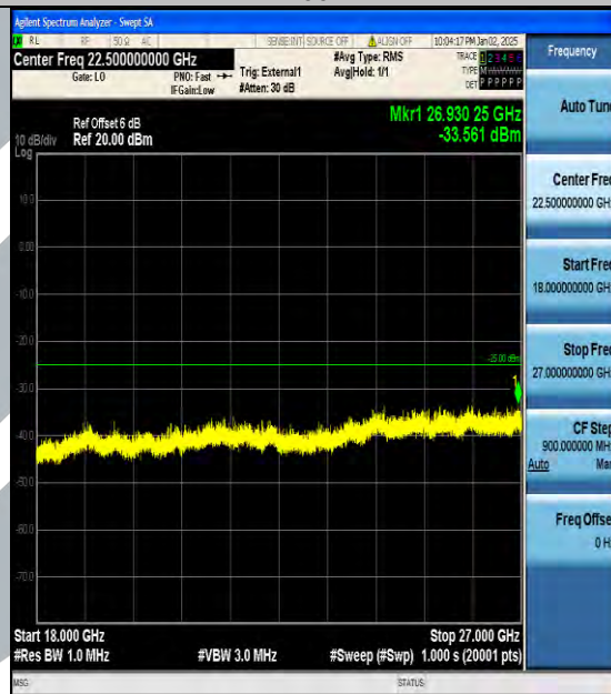
Band38_20MHz_16QAM_38150_1RB#0_18000~27000_18000~27000
