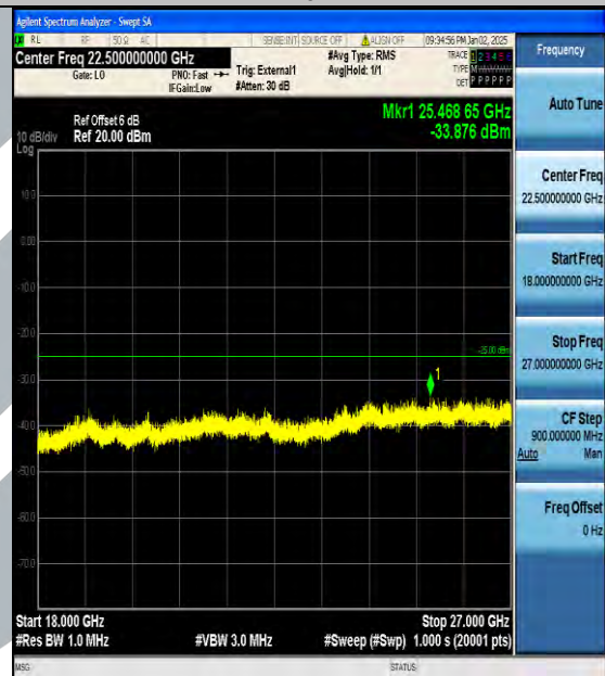
Band38_15MHz_QPSK_38175_1RB#0_18000~27000_18000~27000
