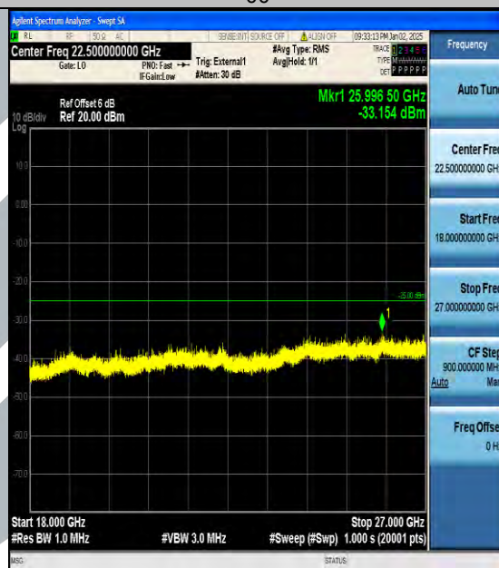
Band38_15MHz_16QAM_38000_1RB#0_18000~27000_18000~27000
