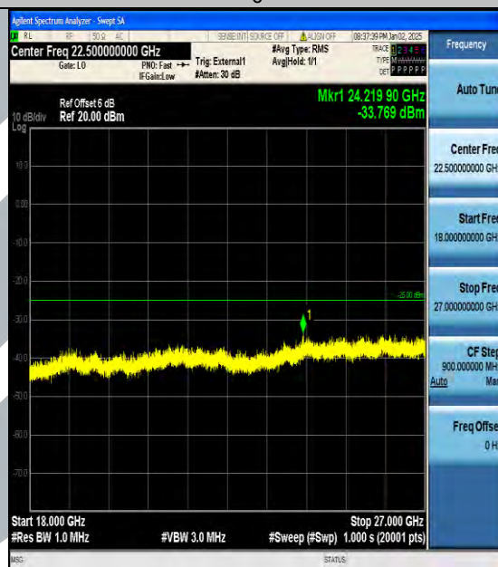
Band38_5MHz_16QAM_38225_1RB#0_18000~27000_18000~27000
