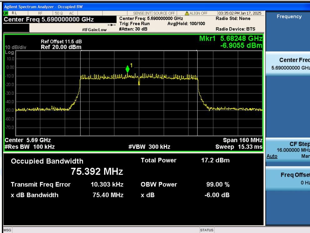
11AC80SISO-Ant1-5690
