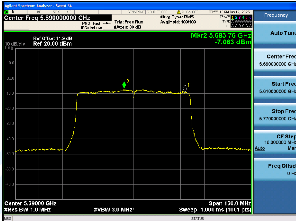
11AC80SISO-Ant1-5690_UNII-2C-PASS
