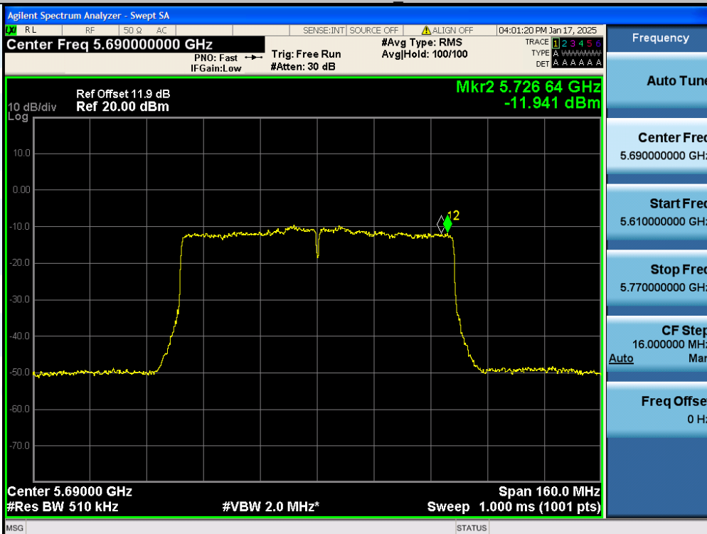
11AC80SISO-Ant1-5690_UNII-3-PASS
