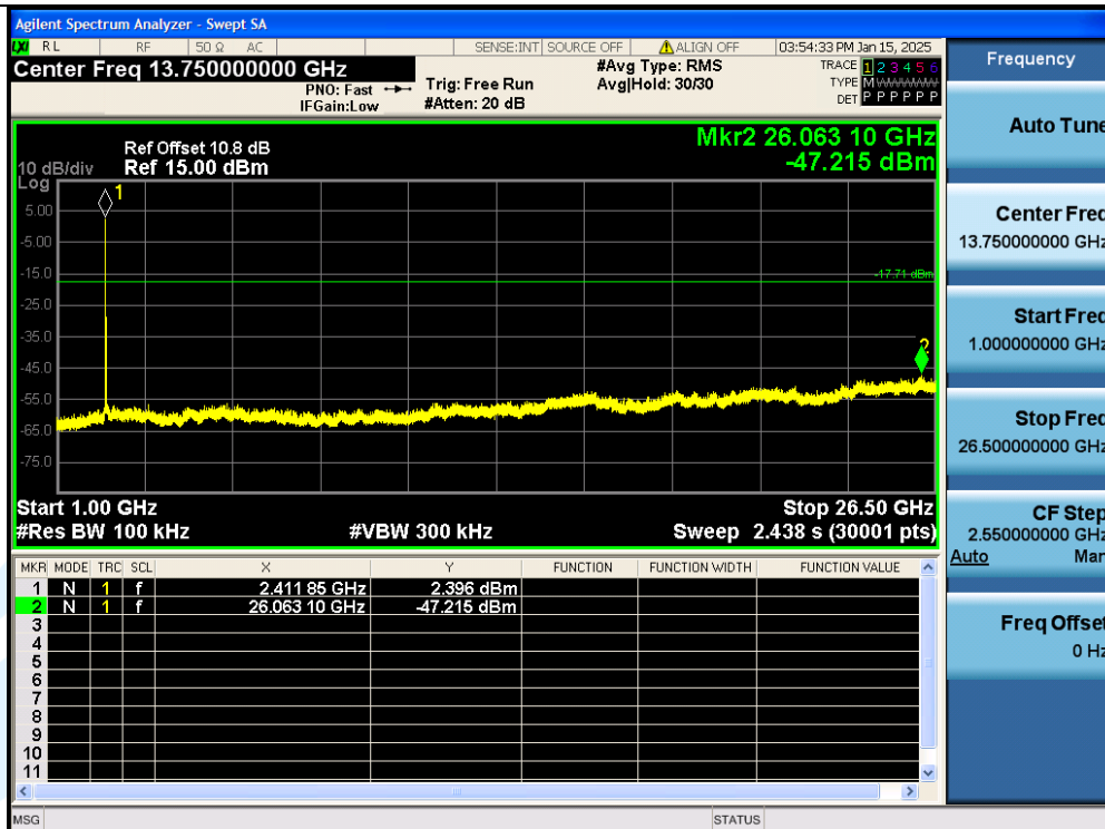
11B-Ant1-2412MHz-1000~26500MHz-PASS
