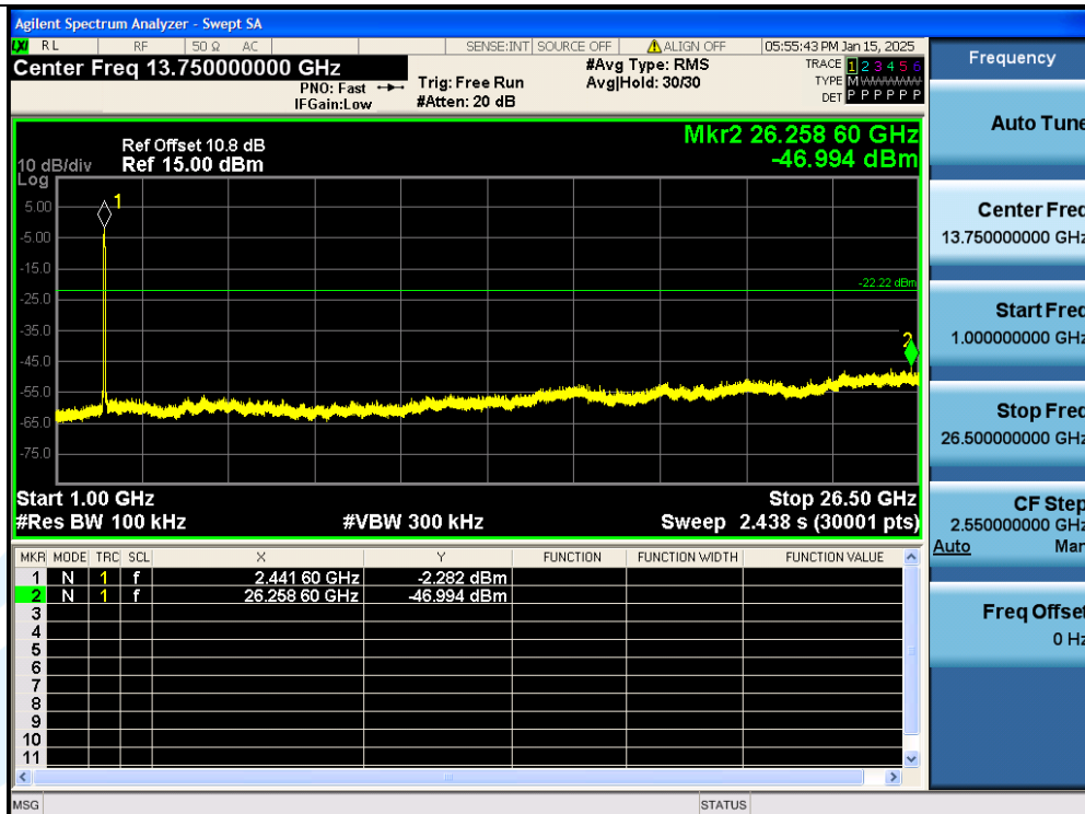
11N40SISO-Ant1-2437MHz-1000~26500MHz-PASS
