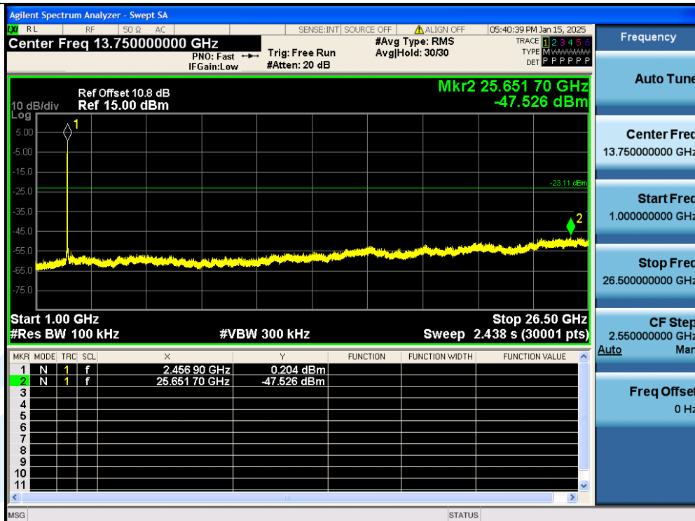
11N20SISO-Ant1-2462MHz-1000~26500MHz-PASS
