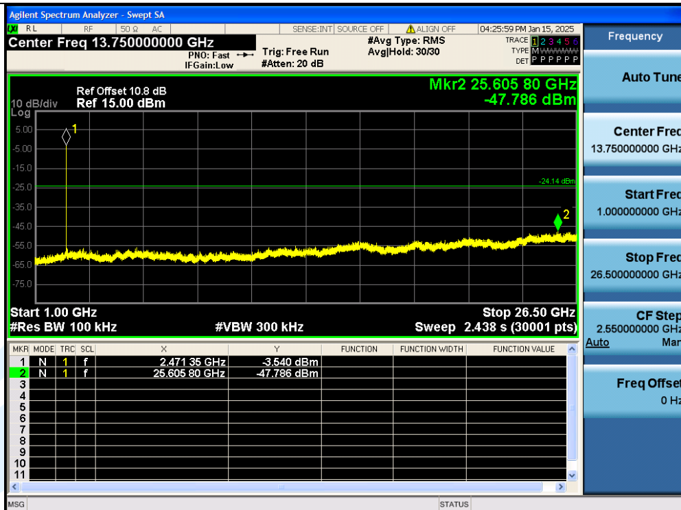
11B-Ant1-2472MHz-1000~26500MHz-PASS
