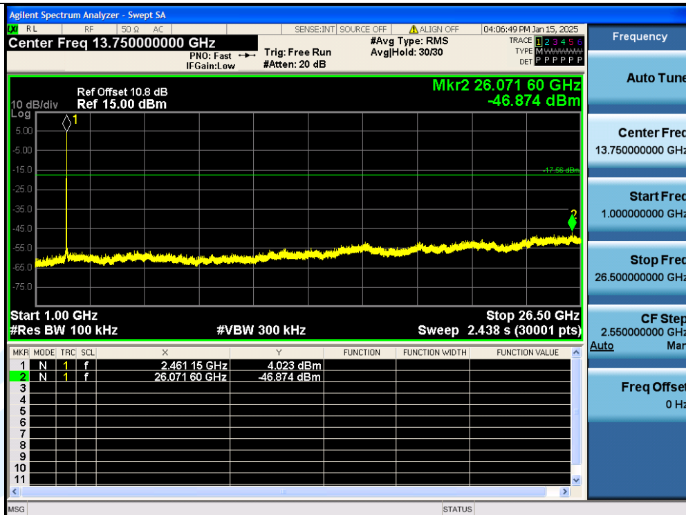
11B-Ant1-2462MHz-1000~26500MHz-PASS
