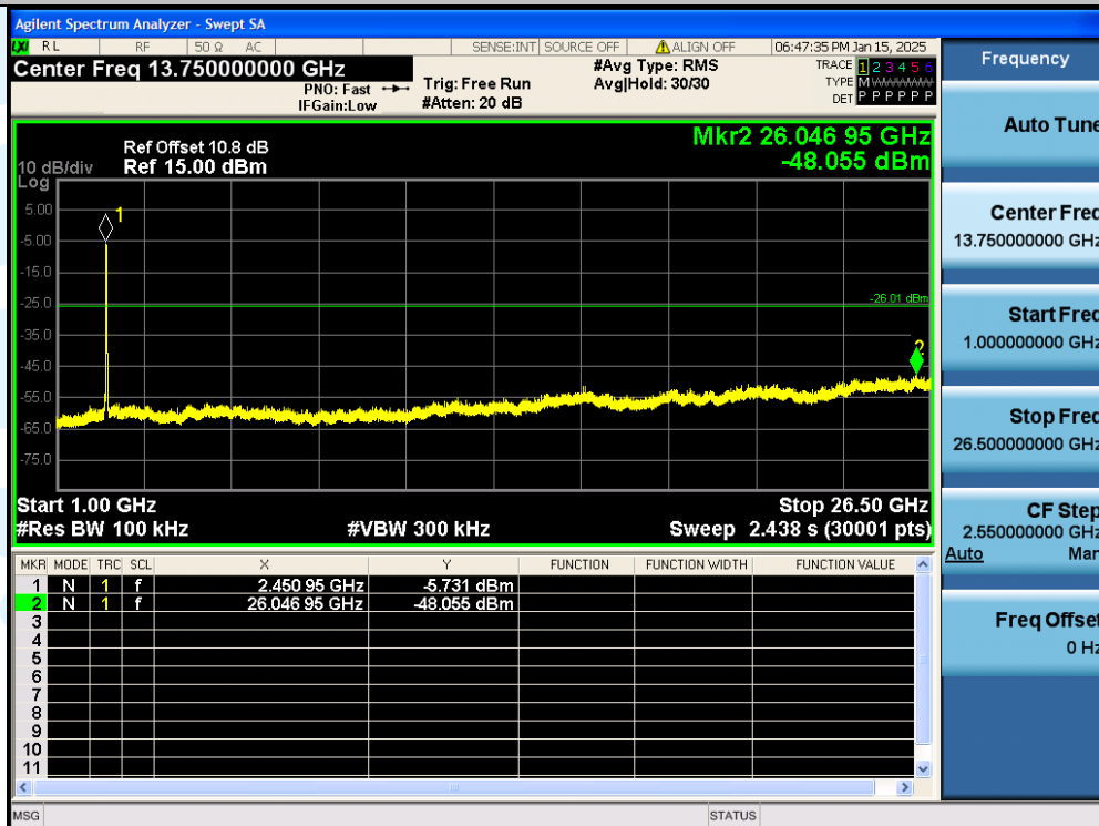
11N40SISO-Ant1-2462MHz-1000~26500MHz-PASS
