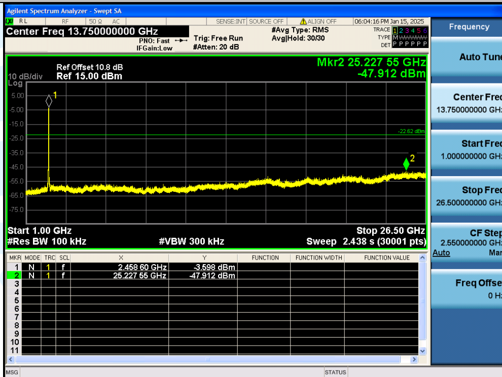
11N40SISO-Ant1-2452MHz-1000~26500MHz-PASS
