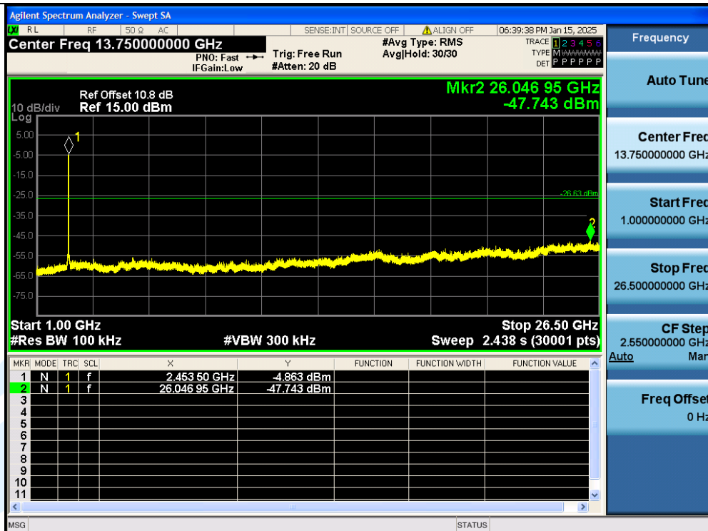
11N40SISO-Ant1-2457MHz-1000~26500MHz-PASS
