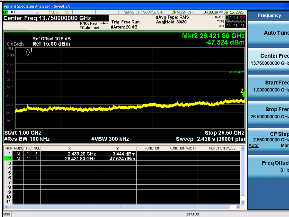
11B-Ant1-2437MHz-1000~26500MHz-PASS
