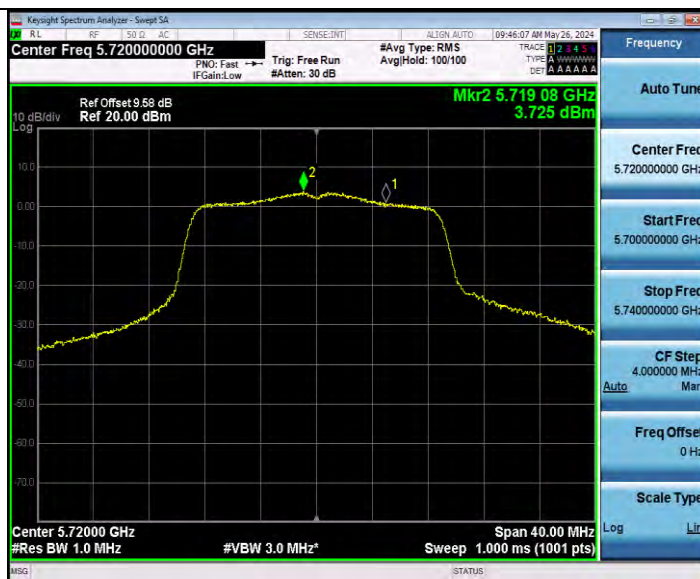
11N20MIMO_Ant9_5720_UNII-2C
