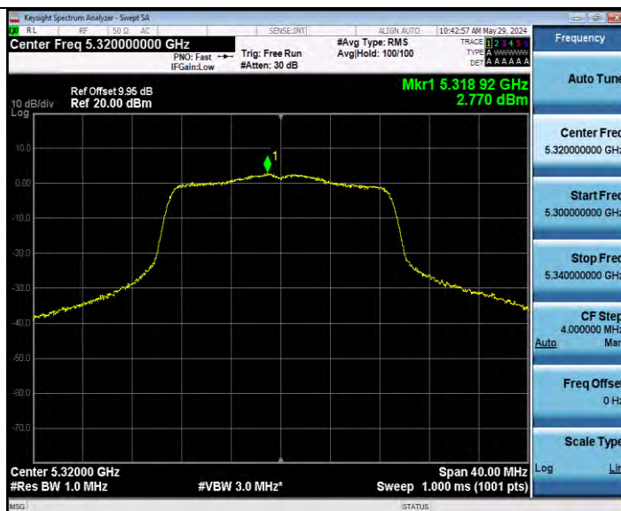
11AC20MIMO_Ant9_5320
