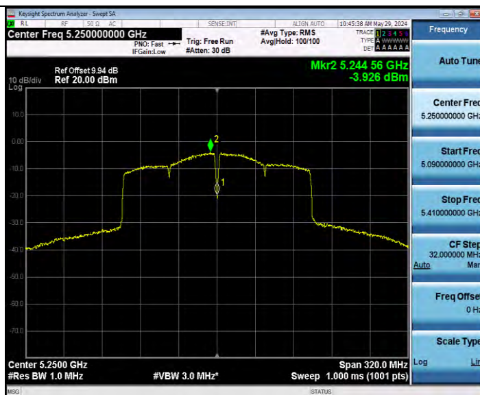
11AC160MIMO_Ant9_5250_UNII-1
