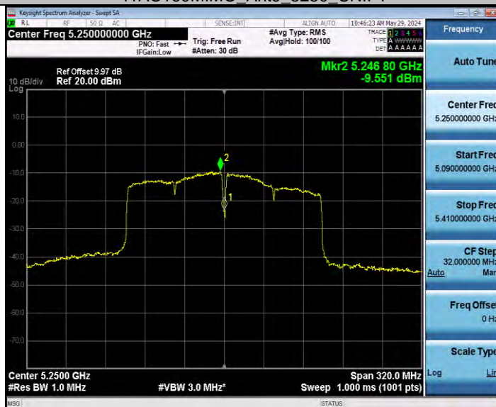
11AC160MIMO_Ant8_5250_UNII-2A
