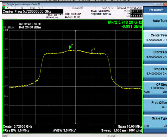
11AX20MIMO_Ant8_5720_UNII-3
