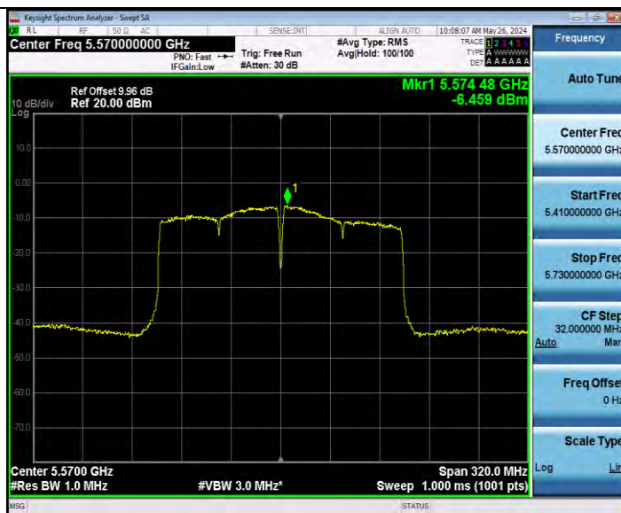
11AC160MIMO_Ant9_5570
