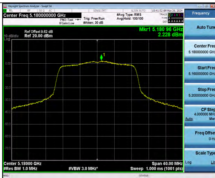
11AC20MIMO_Ant9_5180
