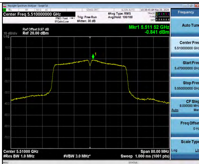
11AC40MIMO_Ant9_5510
