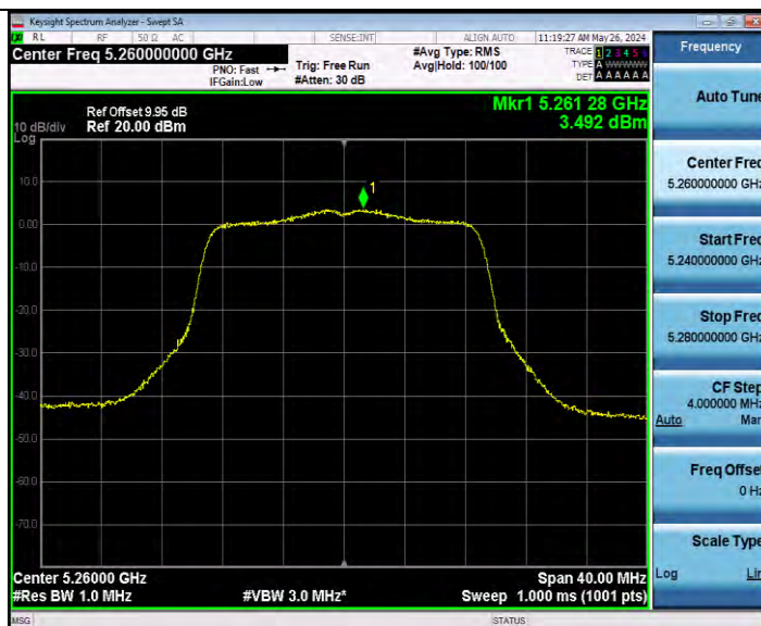
11AC20MIMO_Ant9_5260
