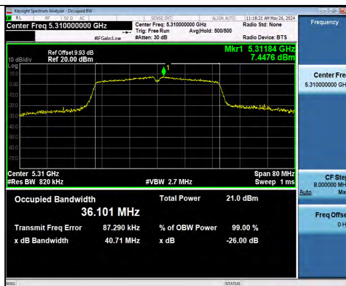
11N40MIMO_Ant9_5310
