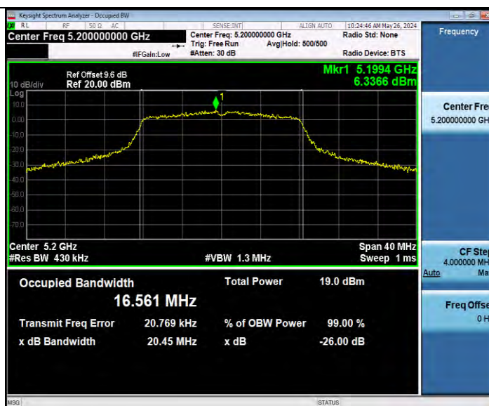
11A-CDD_Ant9_5200
