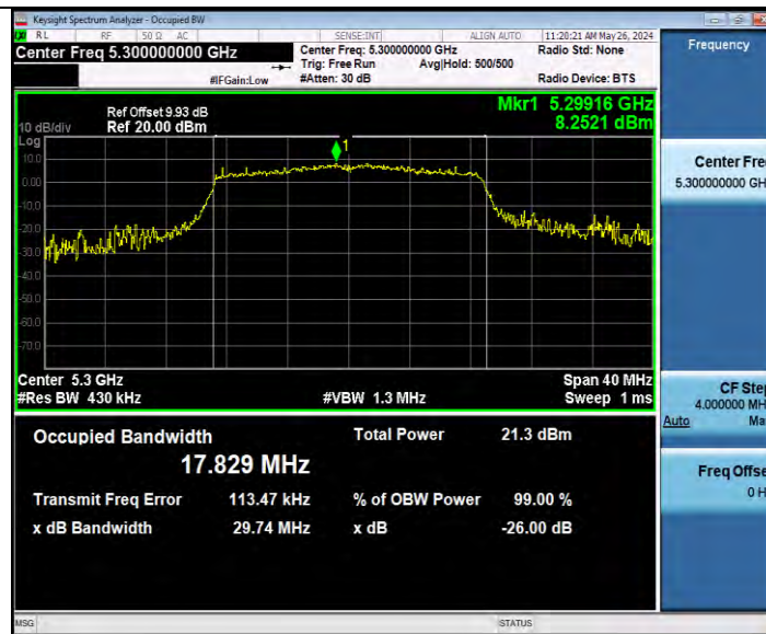
11AC20MIMO_Ant9_5300
