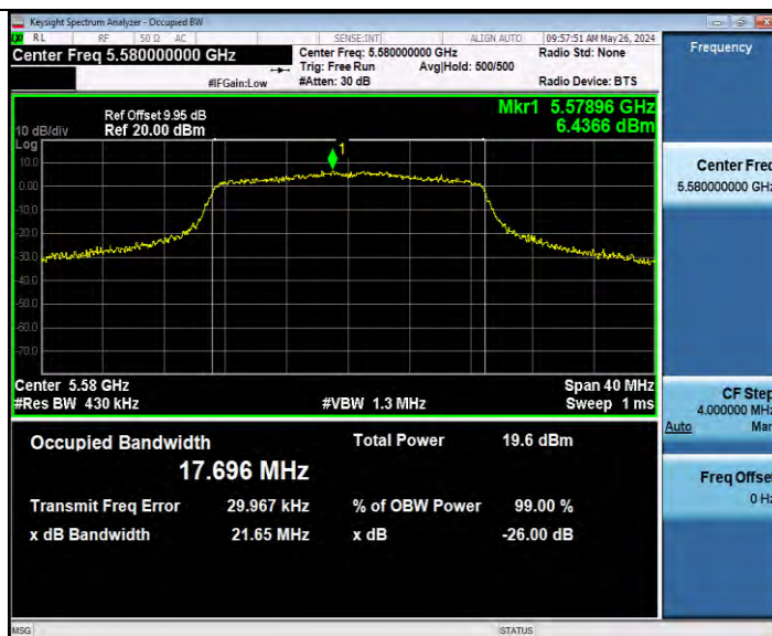
11AC20MIMO_Ant9_5580
