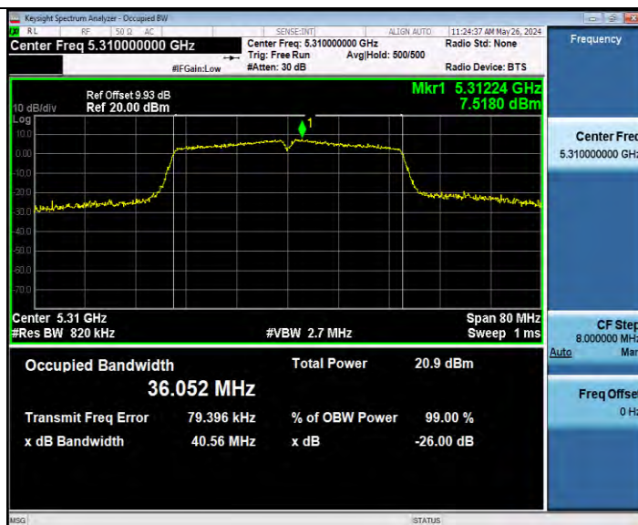
11AC40MIMO_Ant9_5310
