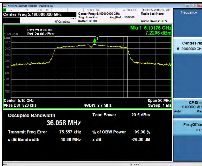
11N40MIMO_Ant9_5190
