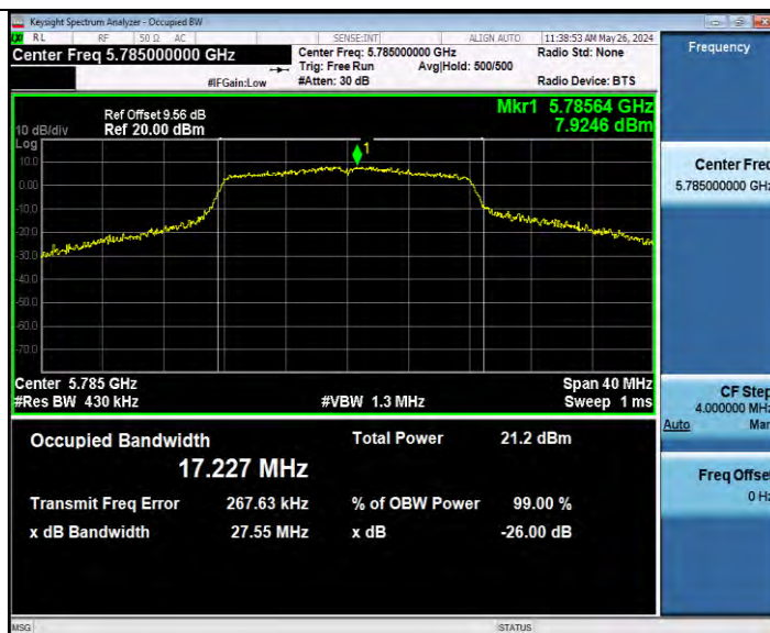
11A-CDD_Ant9_5785
