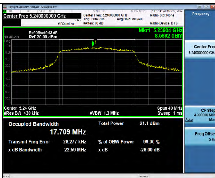
11N20MIMO_Ant9_5240
