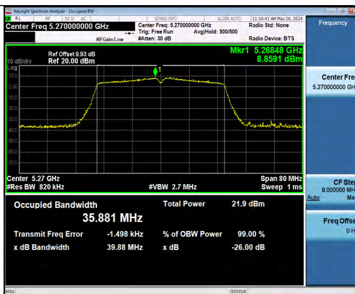
11N40MIMO_Ant9_5270
