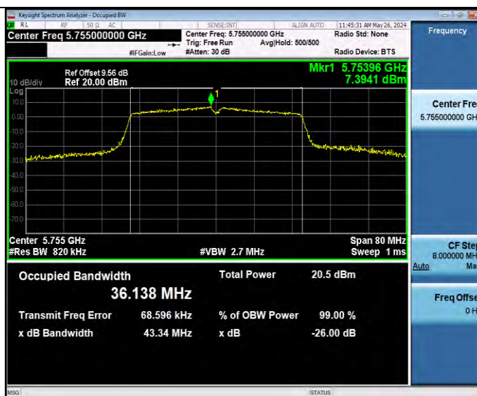
11N40MIMO_Ant9_5755
