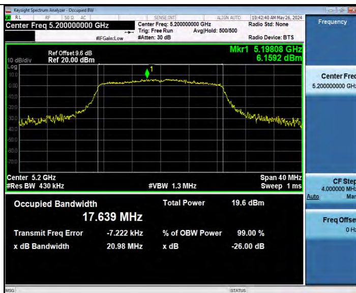
11AC20MIMO_Ant9_5200
