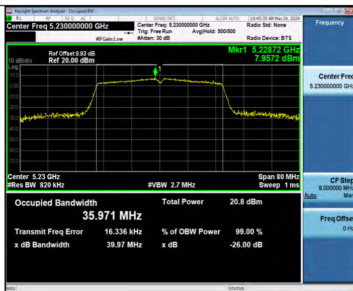
11AC40MIMO_Ant9_5230
