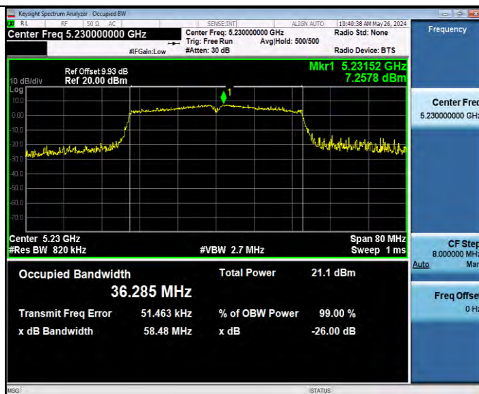
11N40MIMO_Ant9_5230
