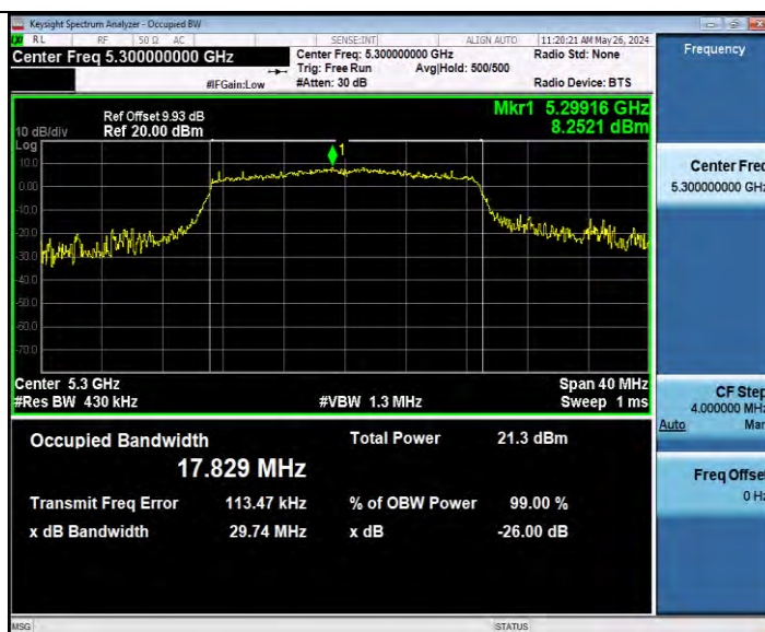
11AC20MIMO_Ant2_5300
