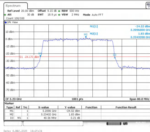
11AX40MIMO-Ant2-5230
