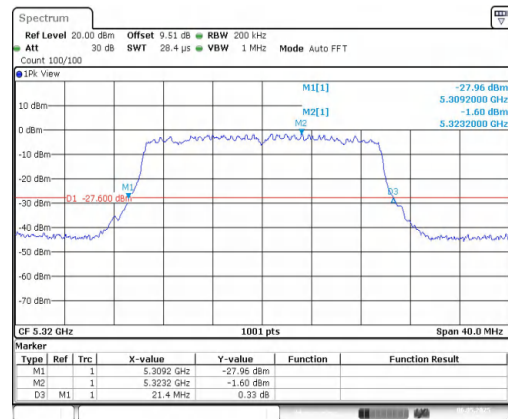
11AX20MIMO-Ant2-5320
