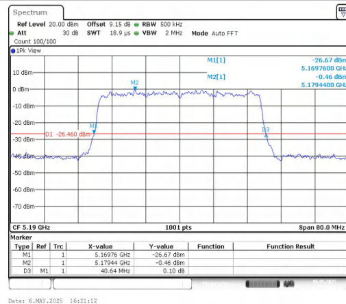
11AX40MIMO-Ant2-5190
