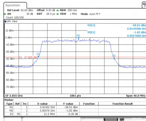
11AX20MIMO-Ant2-5825
