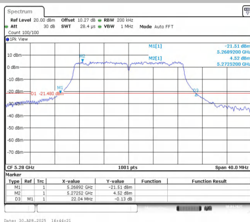
11AC20MIMO-Ant1-5280
