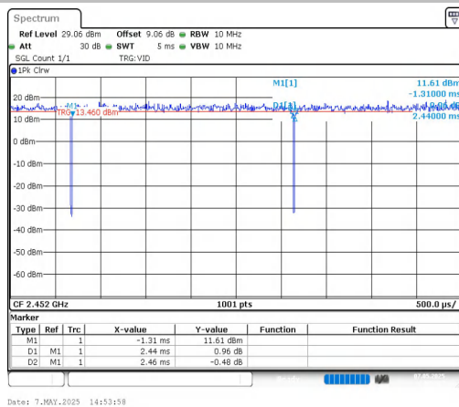
NTNV-11AX40MIMO-Ant1-2452
