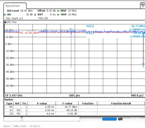
NTNV-11AX20MIMO-Ant2-2437
