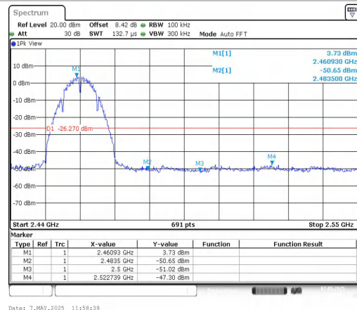
11B-CDD-Ant2-2462-PASS
