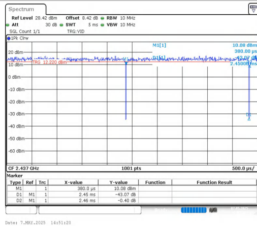
NTNV-11AX40MIMO-Ant2-2437
