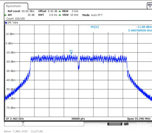
11G-CDD-Ant2-2462-PASS
