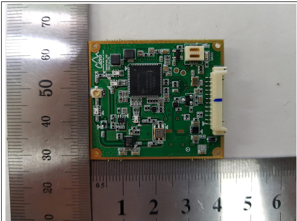
<RFID Module>
