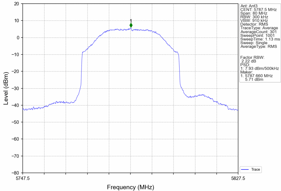
40M_MCH_5787.5MHz_MIMO_NTNV
