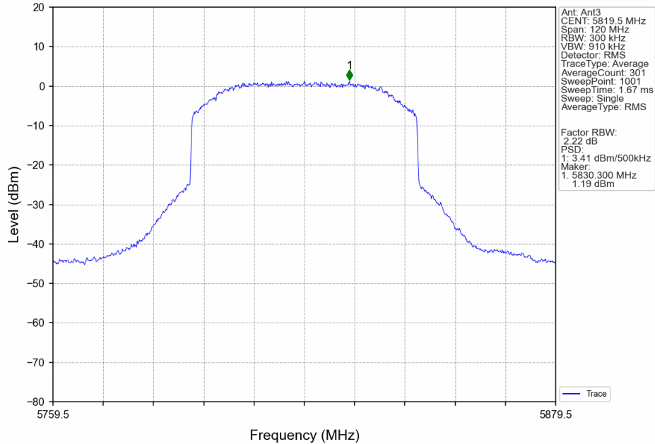
60M_HCH_5819.5MHz_MIMO_NTNV
