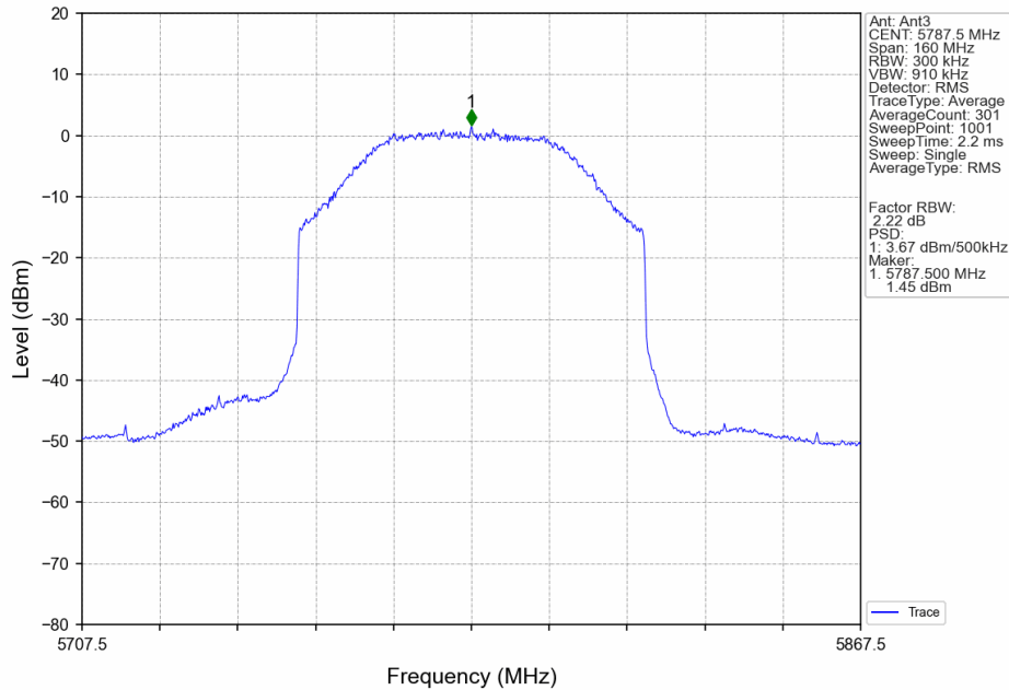
80M_MCH_5787.5MHz_MIMO_NTNV
