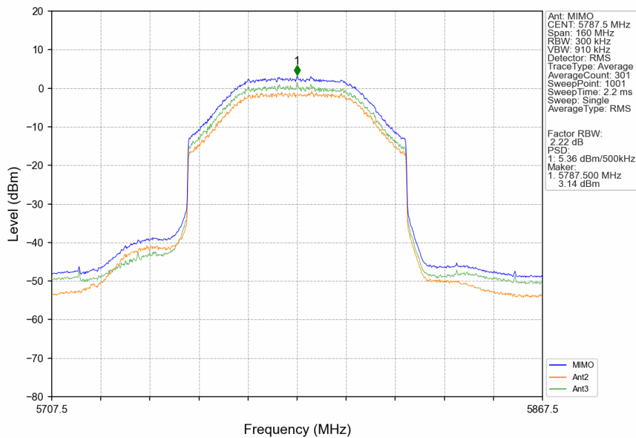
80M_MCH_5787.5MHz_MIMO_NTNV
