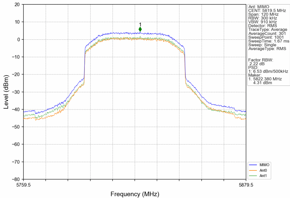
60M_HCH_5819.5MHz_MIMO_NTNV
