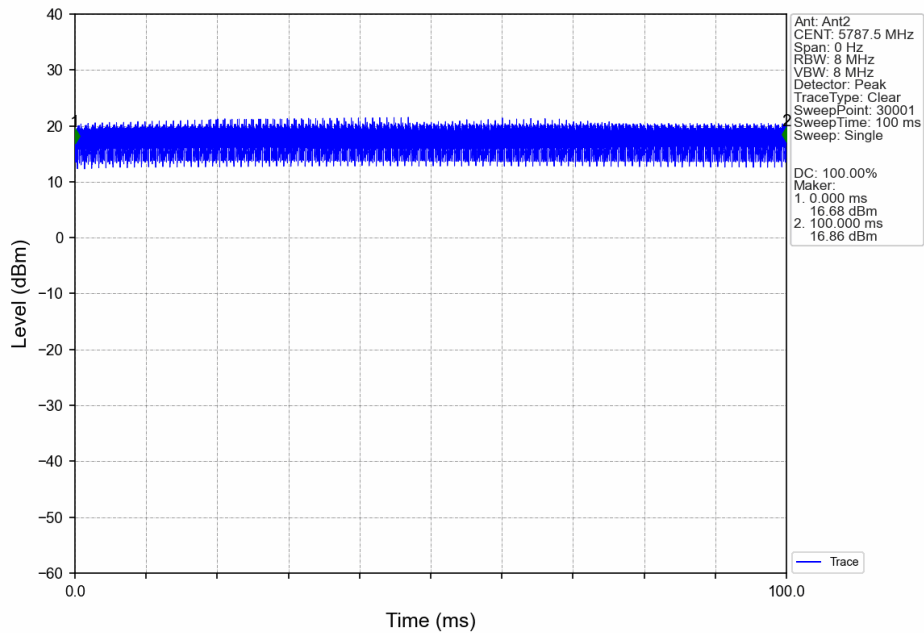
80M_MCH_5787.5MHz_Ant2_NTNV
