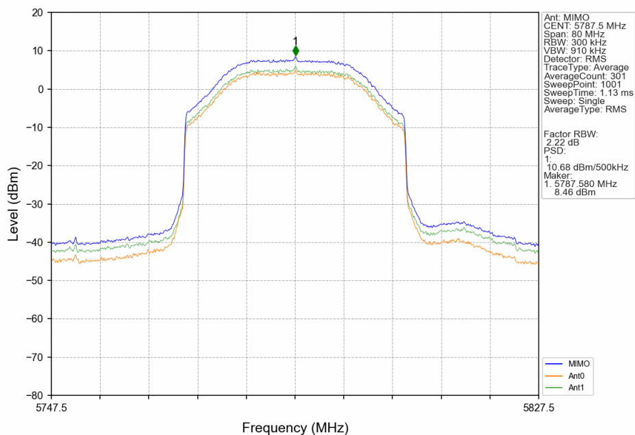
40M_MCH_5787.5MHz_MIMO_NTNV
