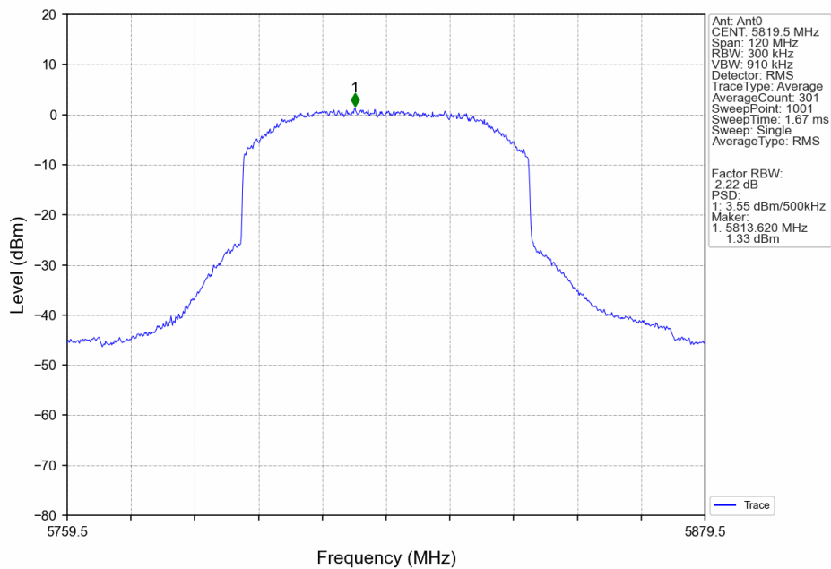
60M_HCH_5819.5MHz_Ant0_NTNV
