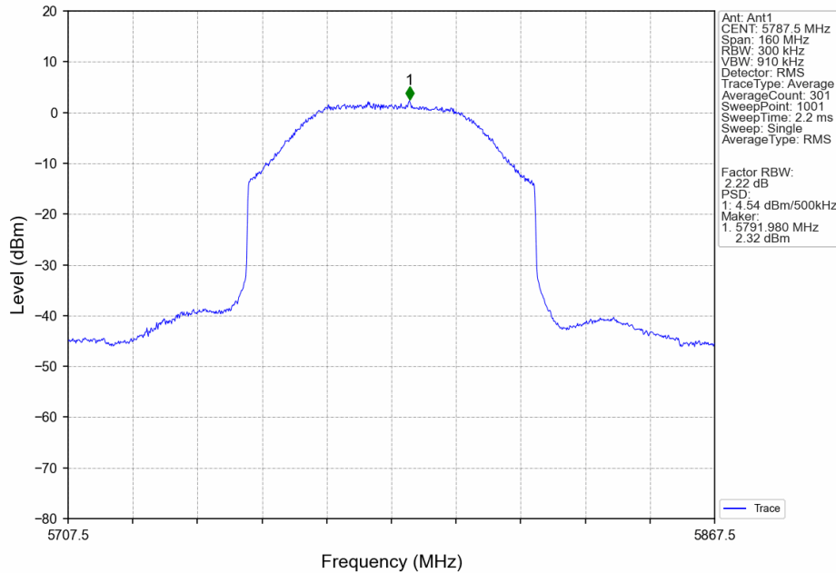
80M_MCH_5787.5MHz_MIMO_NTNV
