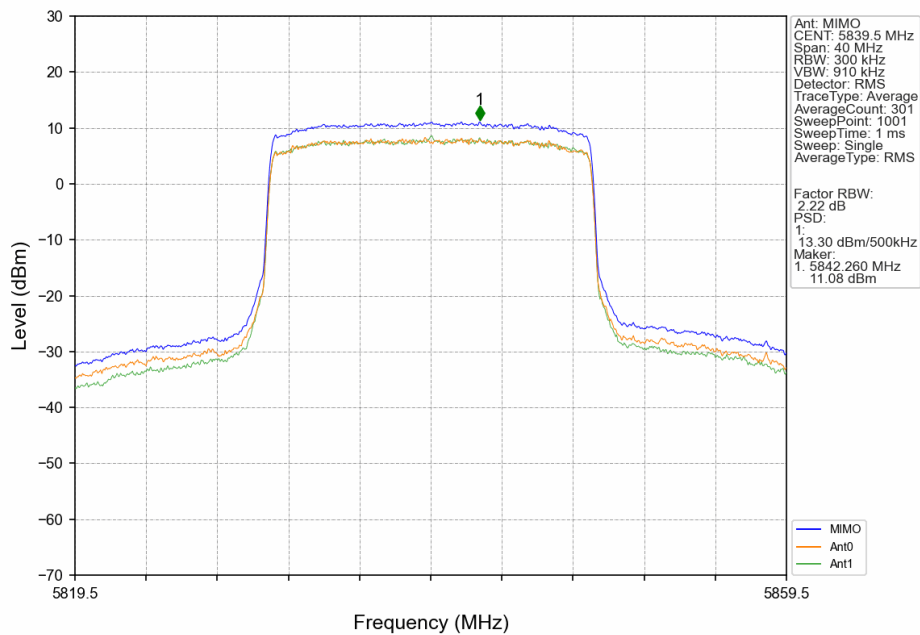
20M_HCH_5839.5MHz_MIMO_NTNV
