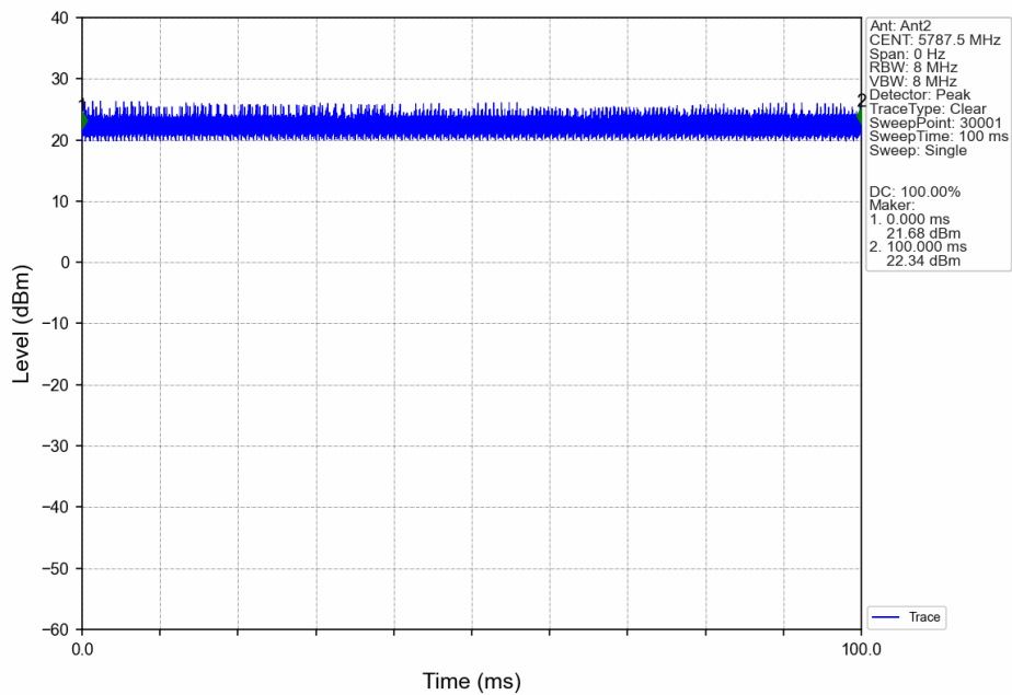
40M_MCH_5787.5MHz_Ant2_NTNV
