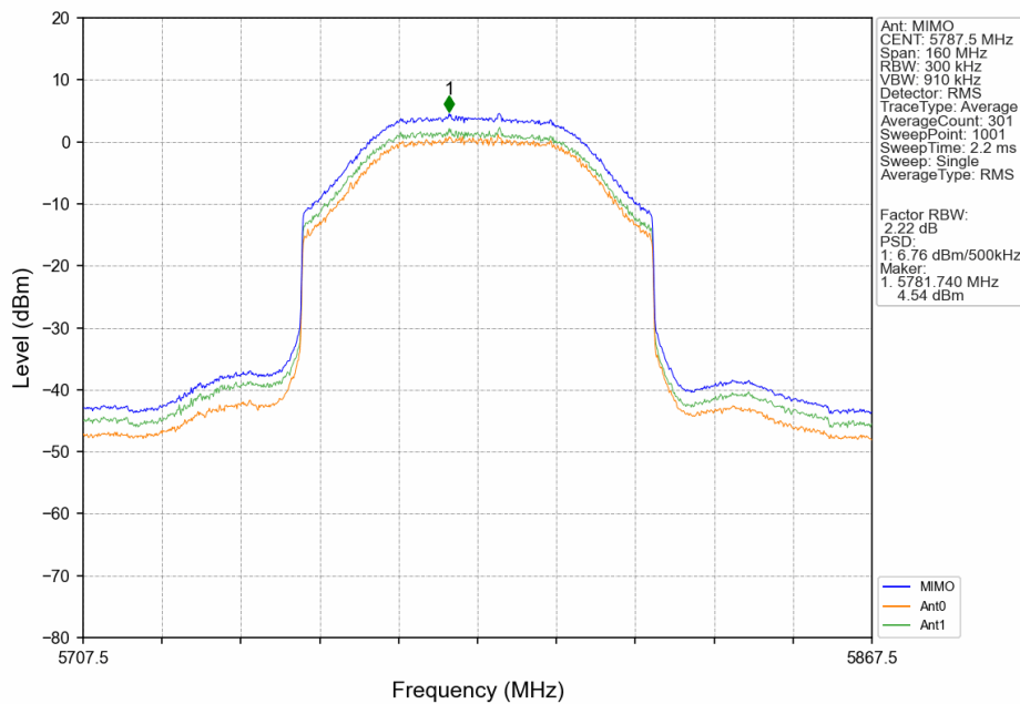
80M_MCH_5787.5MHz_MIMO_NTNV
