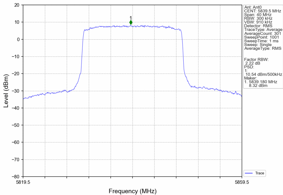
20M_HCH_5839.5MHz_Ant0_NTNV
