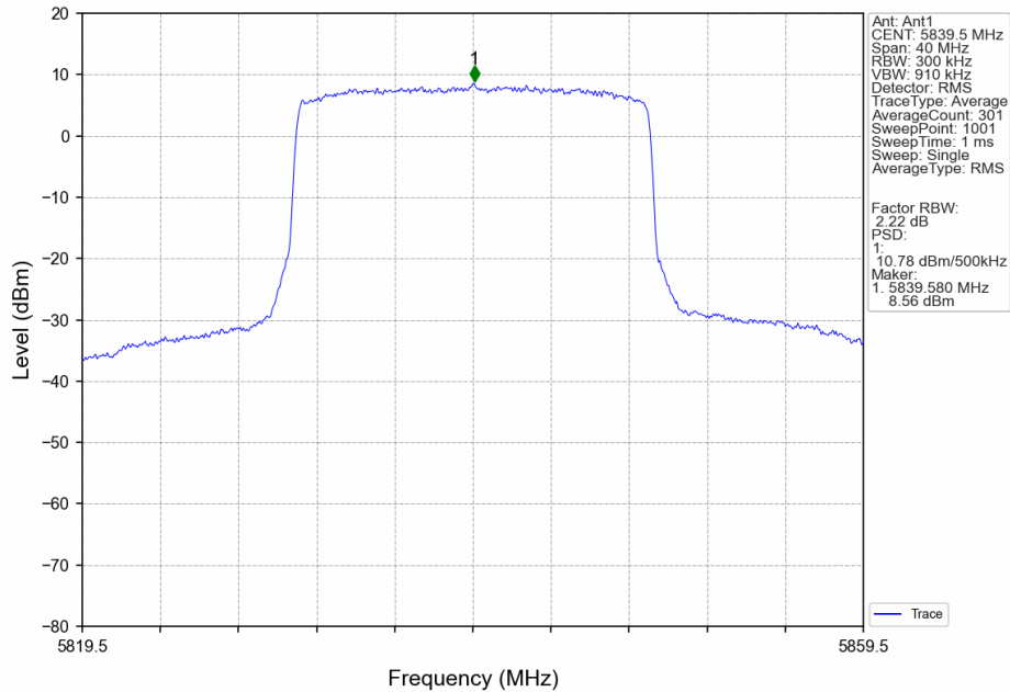
20M_HCH_5839.5MHz_MIMO_NTNV
