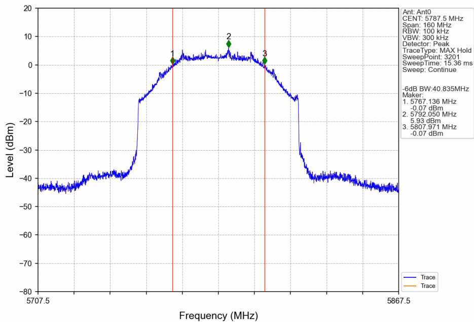
80M_MCH_5787.5MHz_Ant0_NTNV
