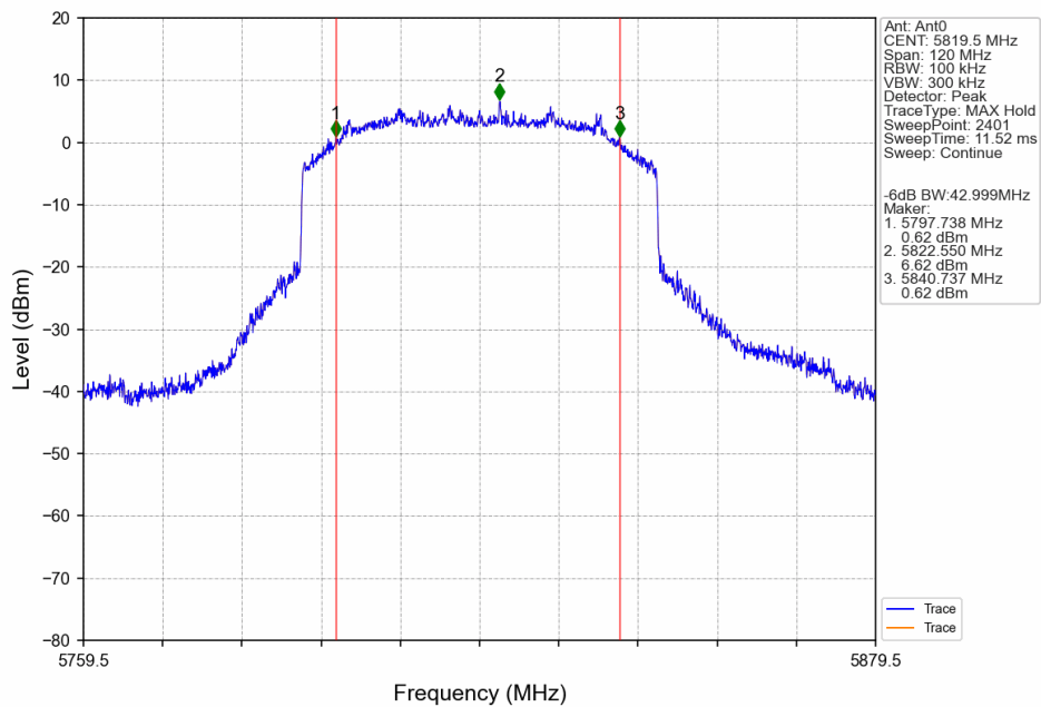
60M_HCH_5819.5MHz_Ant0_NTNV
