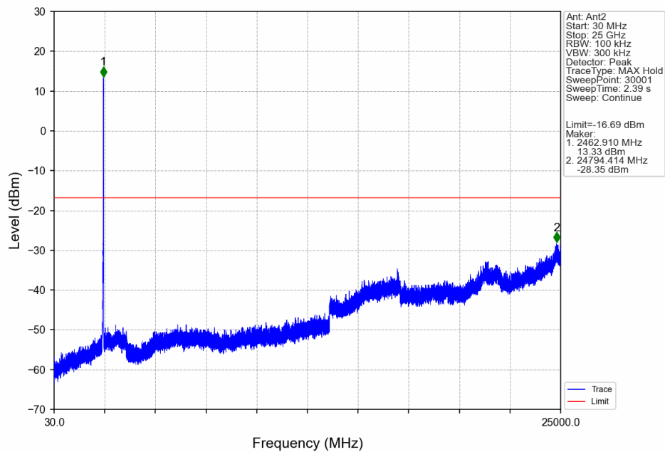
20M_HCH_2462.5MHz_Ant2_NTNV
