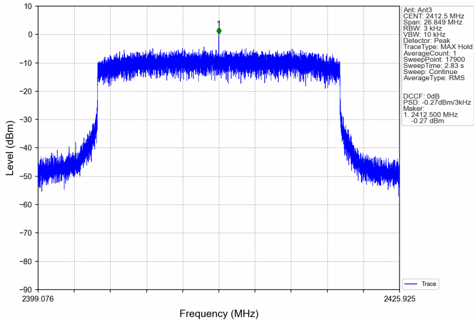
20M_LCH_2412.5MHz_MIMO_NTNV
