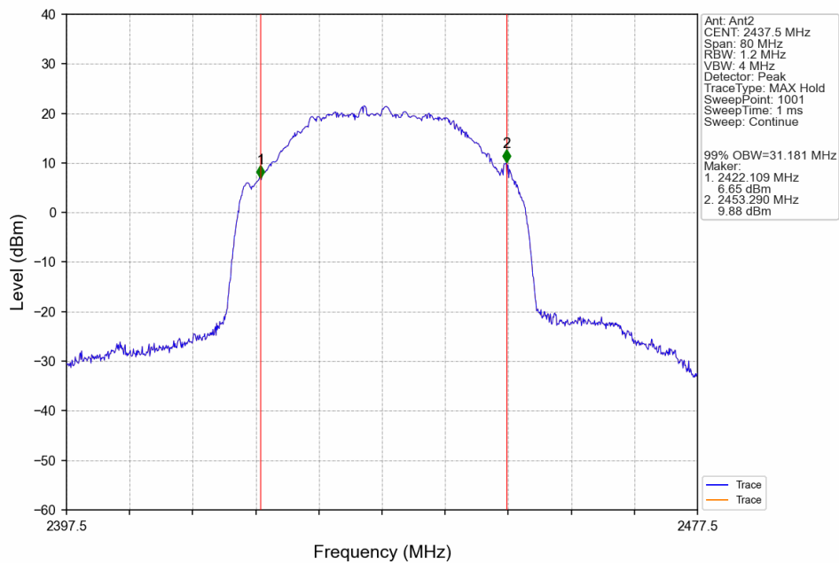
40M_MCH_2437.5MHz_Ant2_NTNV
