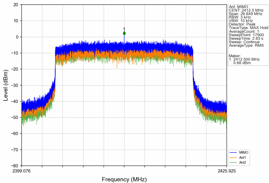
20M_LCH_2412.5MHz_MIMO_NTNV
