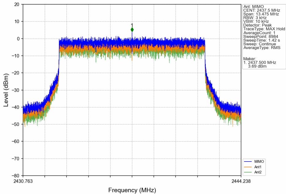
10M_MCH_2437.5MHz_MIMO_NTNV
