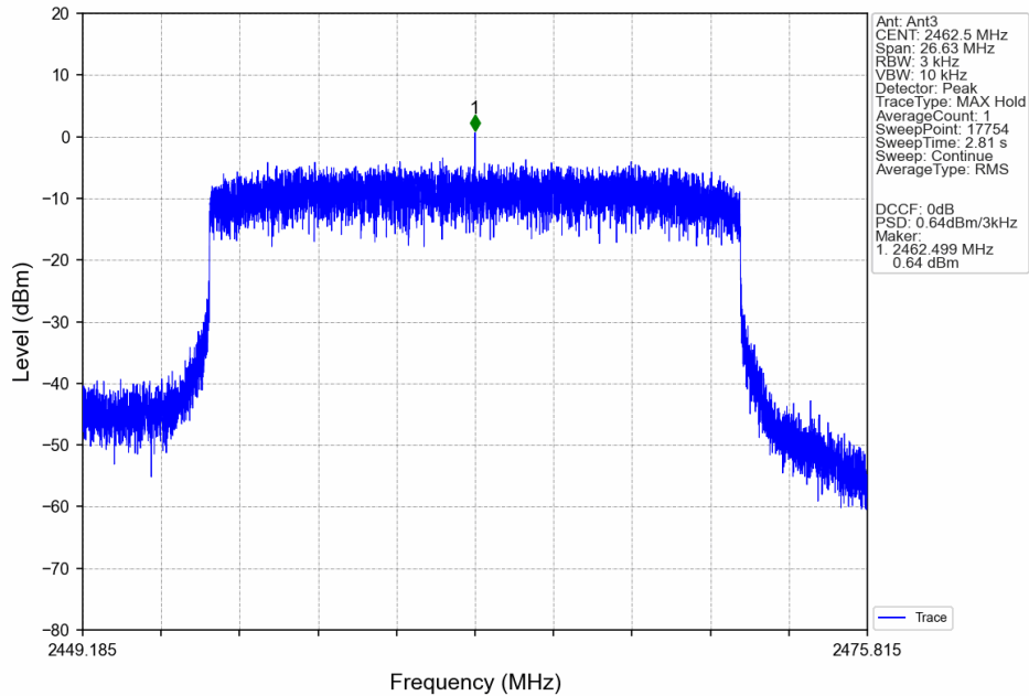
20M_HCH_2462.5MHz_MIMO_NTNV
