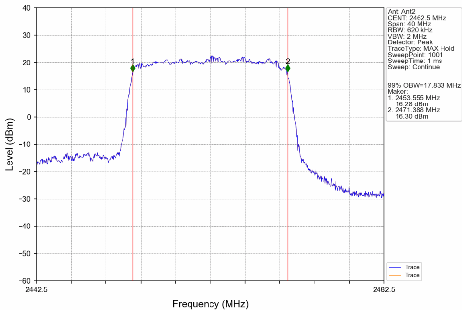
20M_HCH_2462.5MHz_Ant2_NTNV
