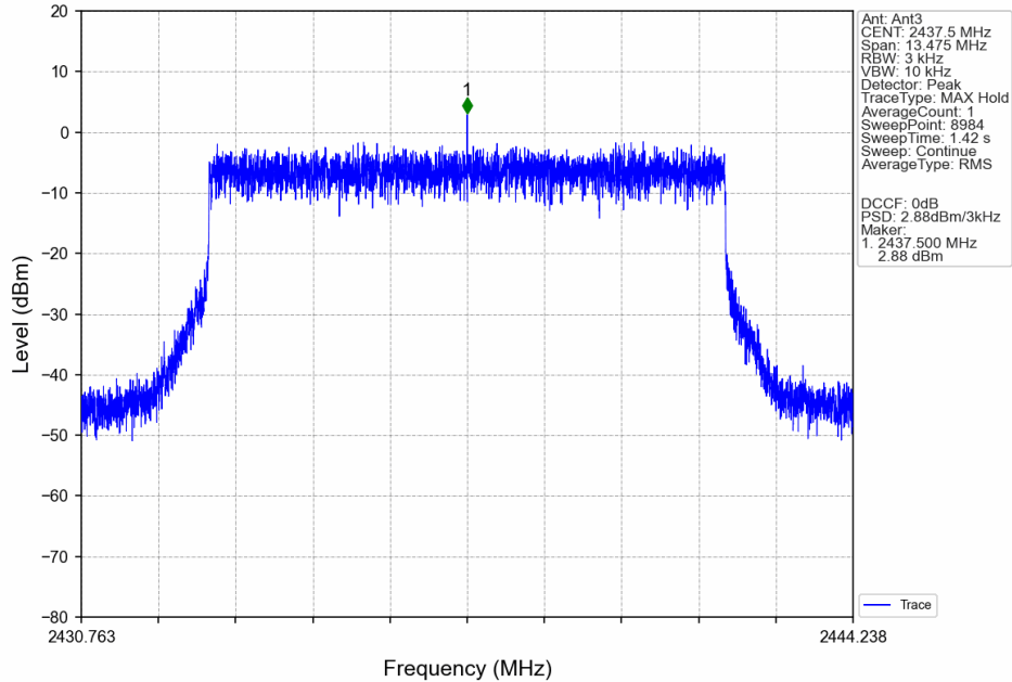
10M_MCH_2437.5MHz_MIMO_NTNV
