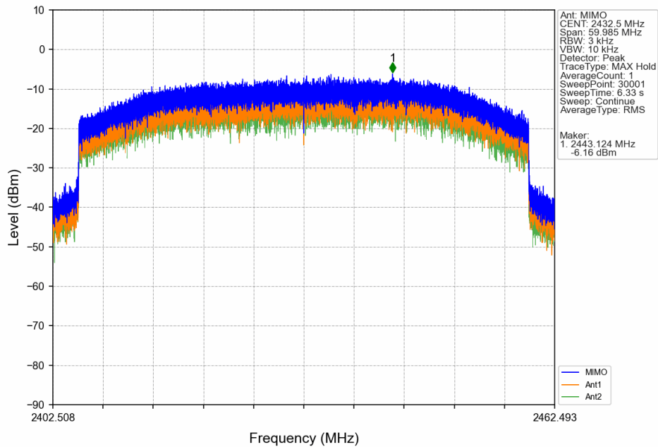
60M_LCH_2432.5MHz_MIMO_NTNV
