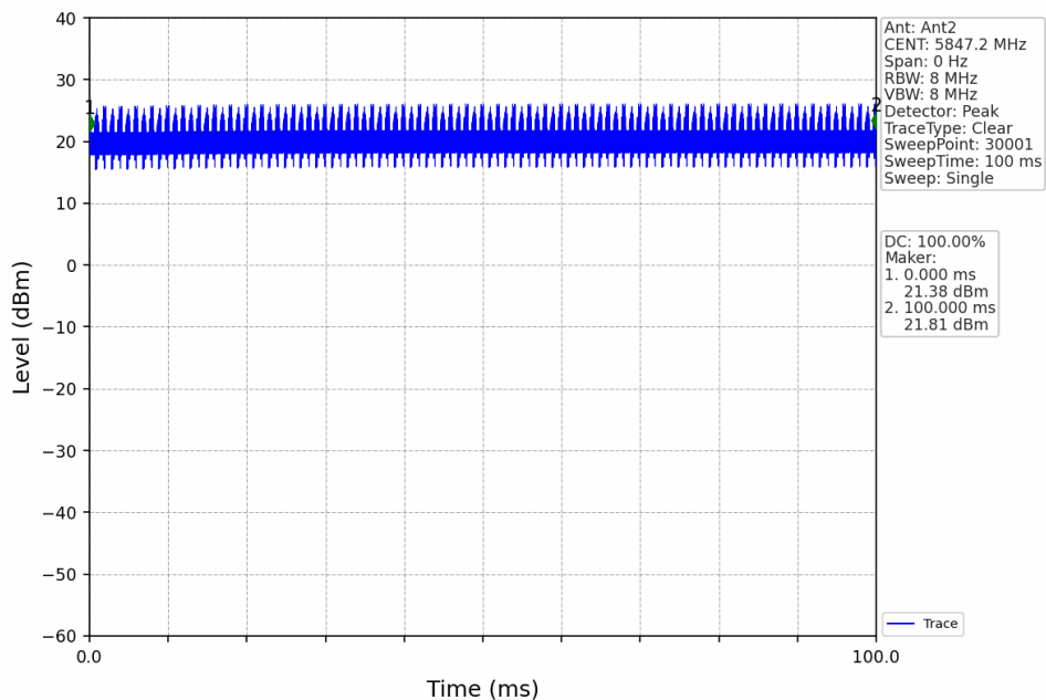
3M_HCH_5847.2MHz_Ant2_NTNV
