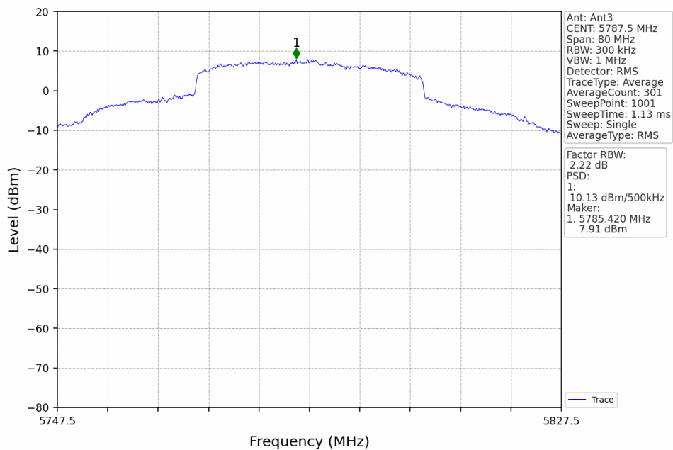
40M_MCH_5787.5MHz_Ant3_NTNV
