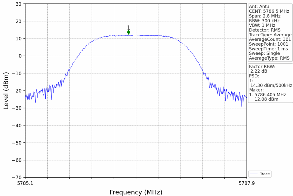
1.4M_MCH_5786.5MHz_MIMO_NTNV
