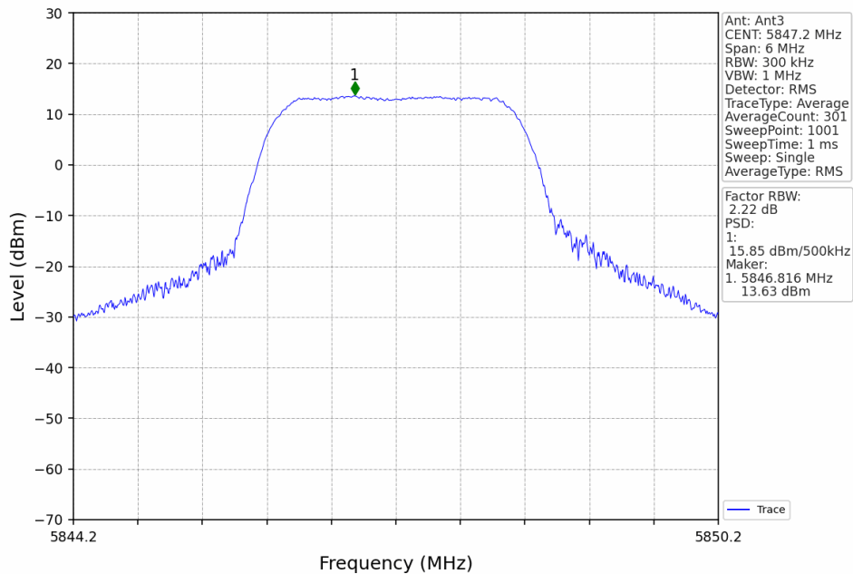
3M_HCH_5847.2MHz_Ant3_NTNV
