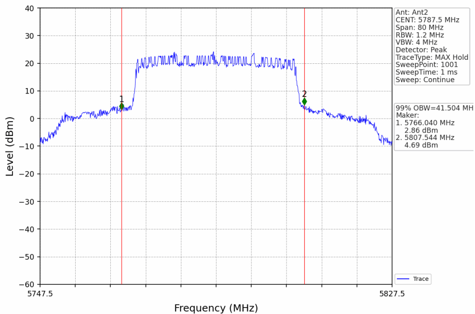
40M_MCH_5787.5MHz_Ant2_NTNV
