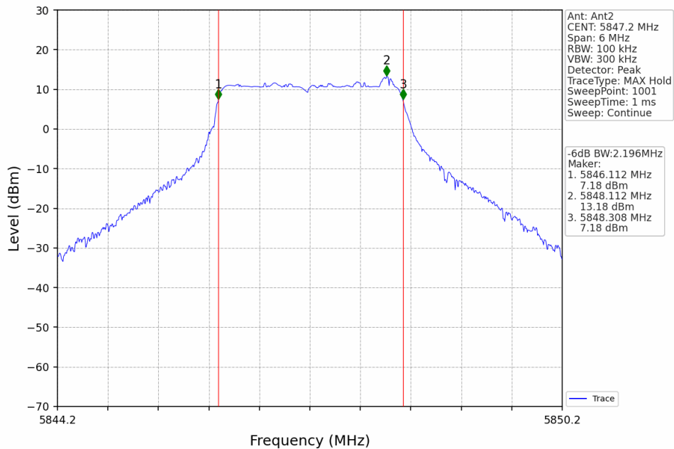
3M_HCH_5847.2MHz_Ant2_NTNV
