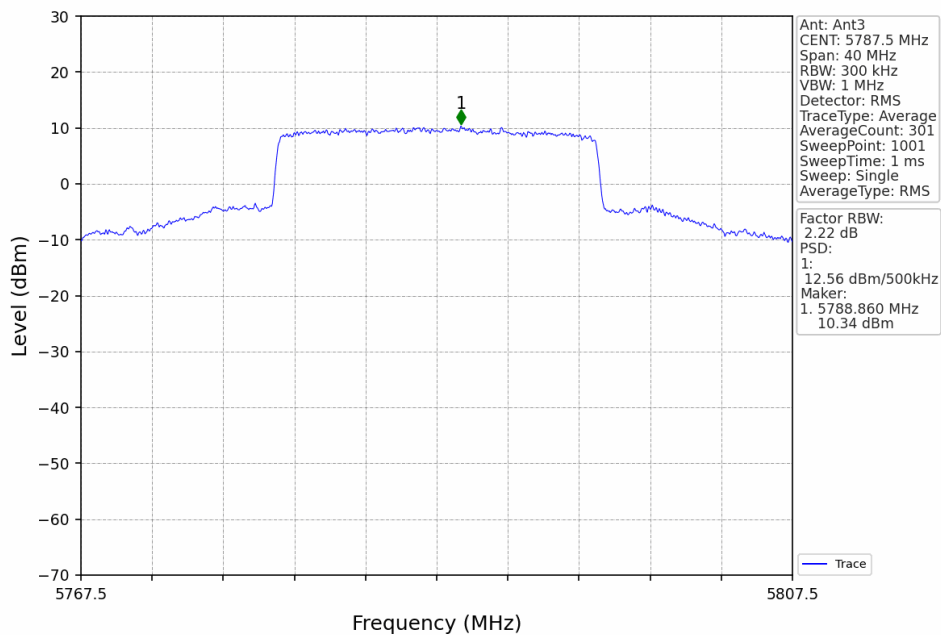
20M_MCH_5787.5MHz_Ant3_NTNV
