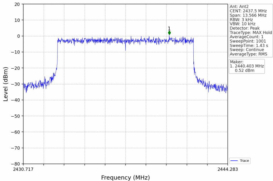
10M_MCH_2437.5MHz_Ant2_NTNV
