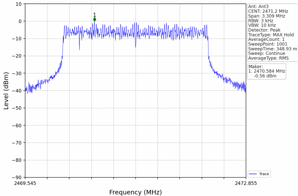
3M_HCH_2471.2MHz_MIMO_NTNV
