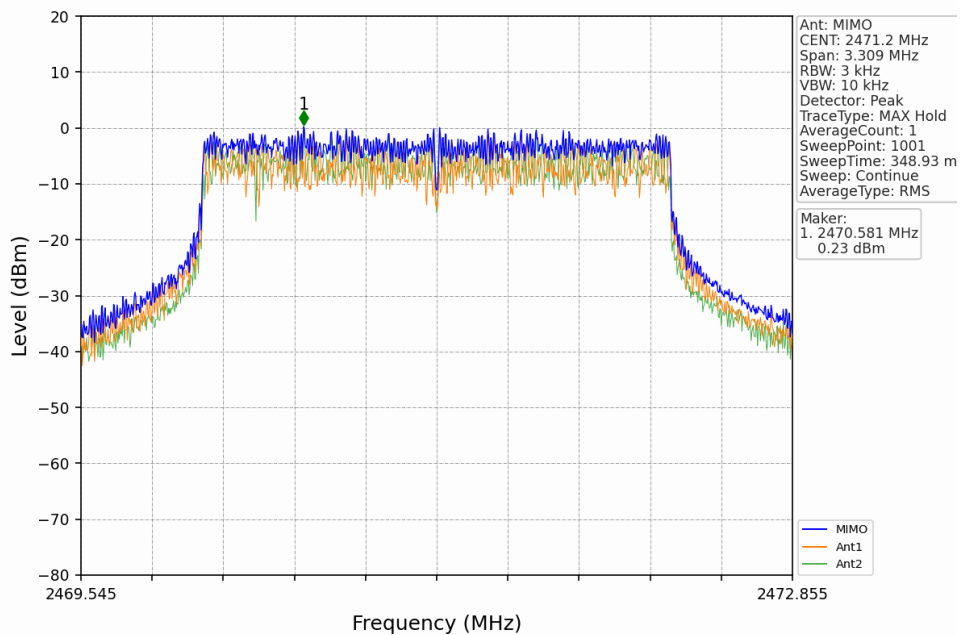
3M_HCH_2471.2MHz_MIMO_NTNV
