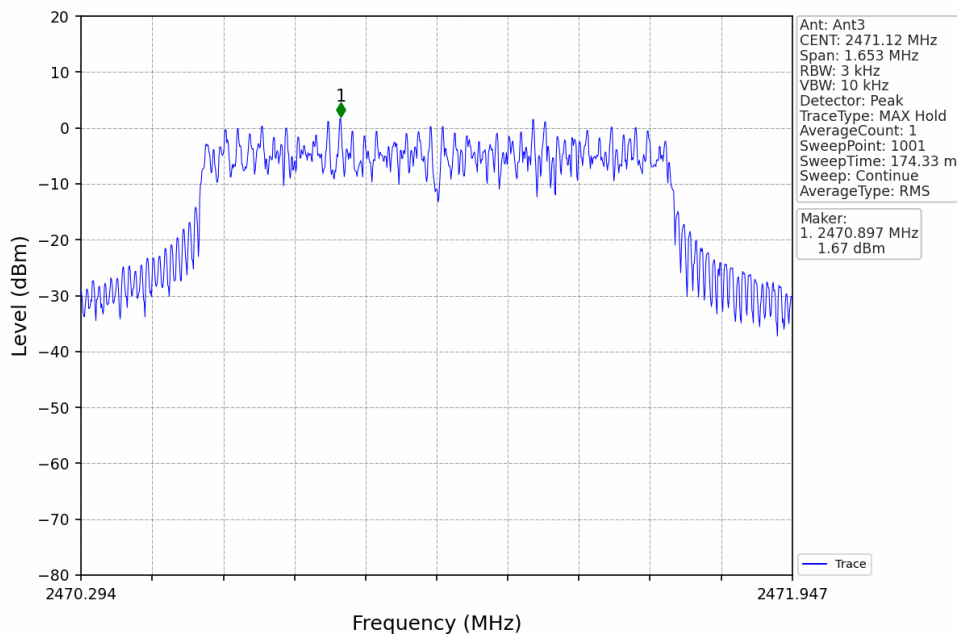
1.4M_HCH_2471.12MHz_Ant3_NTNV
