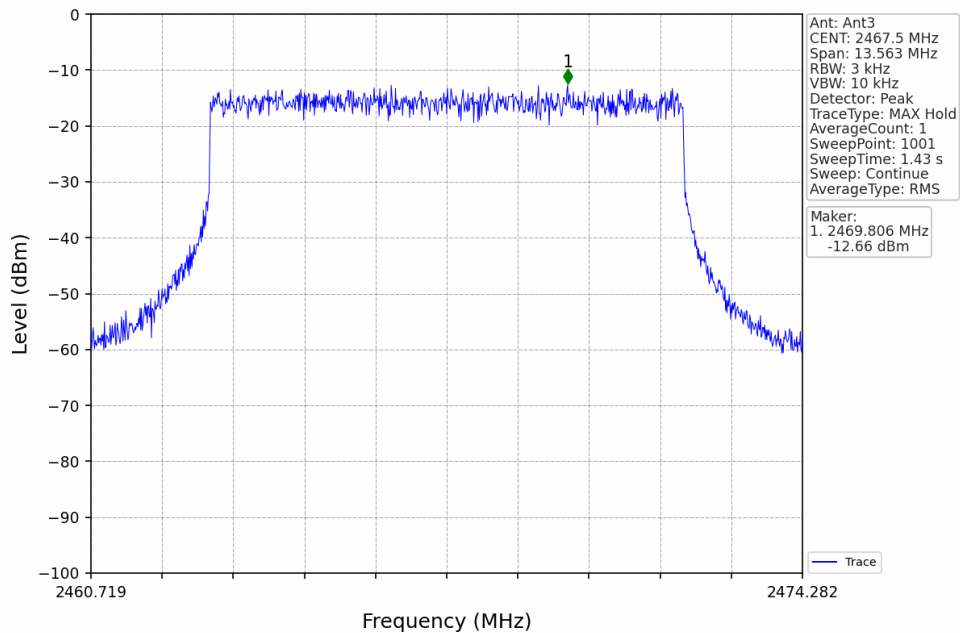
10M_HCH_2467.5MHz_Ant3_NTNV
