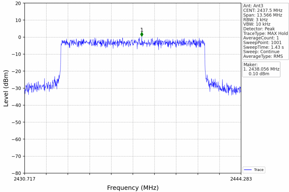
10M_MCH_2437.5MHz_MIMO_NTNV
