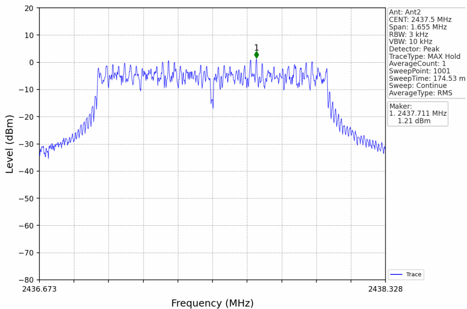
1.4M_MCH_2437.5MHz_Ant2_NTNV
