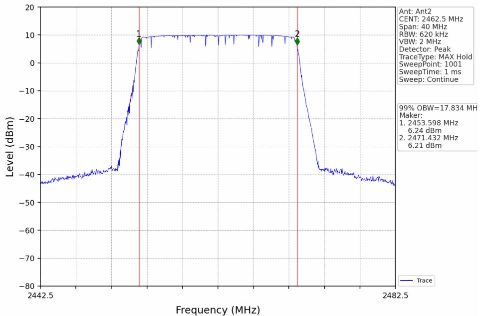
20M_HCH_2462.5MHz_Ant2_NTNV
