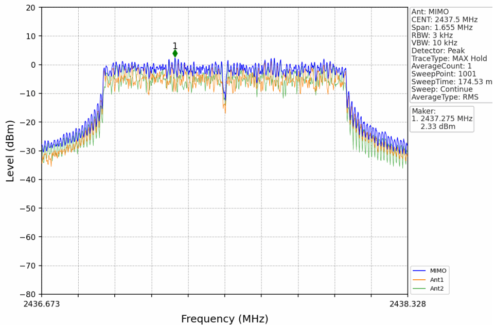
1.4M_MCH_2437.5MHz_MIMO_NTNV
