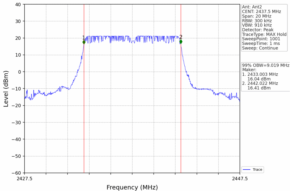
10M_MCH_2437.5MHz_Ant2_NTNV
