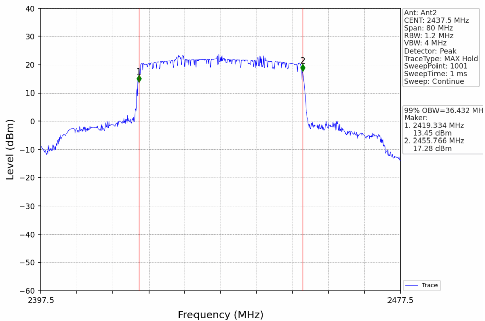
40M_MCH_2437.5MHz_Ant2_NTNV
