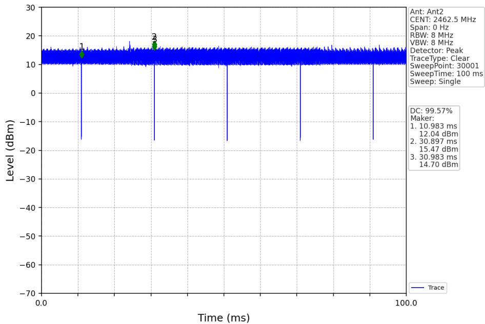
20M_HCH_2462.5MHz_Ant2_NTNV
