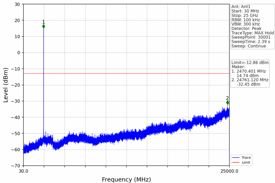
1.4M_HCH_2471.12MHz_Ant1_NTNV
