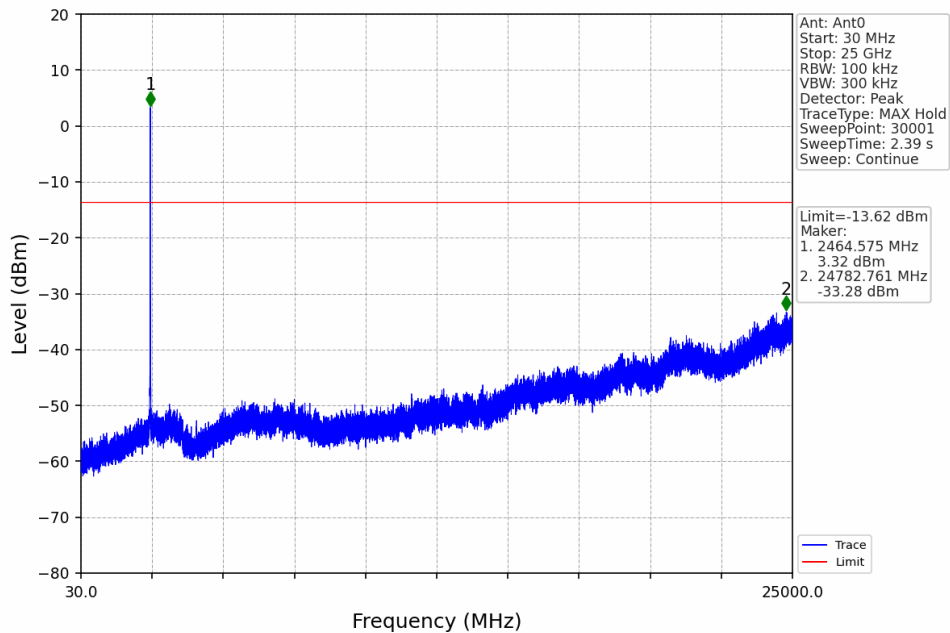
20M_HCH_2462.5MHz_Ant0_NTNV
