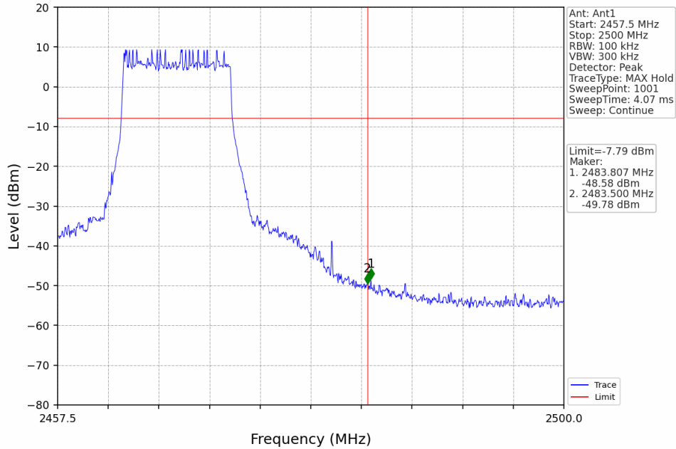
10M_HCH_2467.5MHz_Ant1_NTNV
