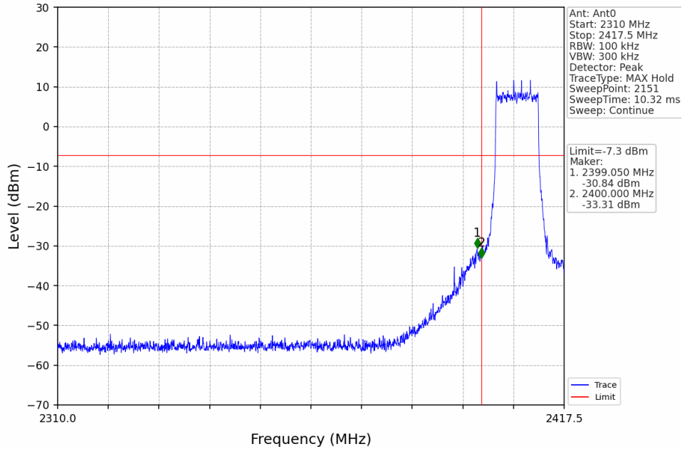
10M_LCH_2407.5MHz_Ant0_NTNV
