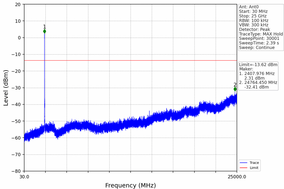
20M_LCH_2412.5MHz_Ant0_NTNV
