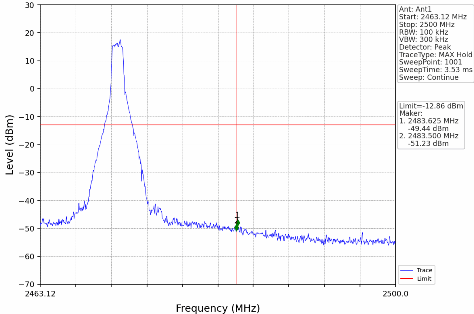
1.4M_HCH_2471.12MHz_Ant1_NTNV
