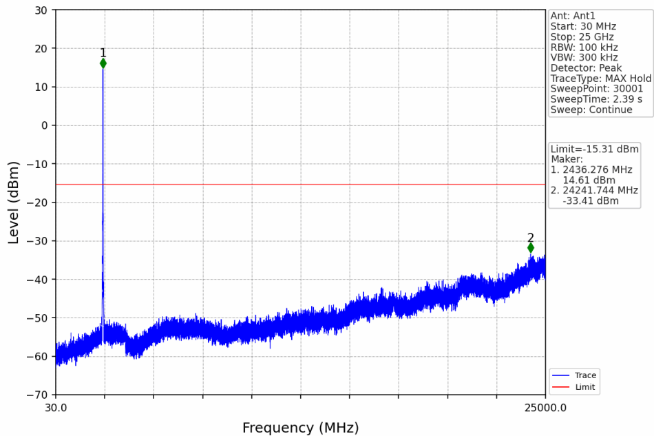
20M_MCH_2437.5MHz_Ant1_NTNV
