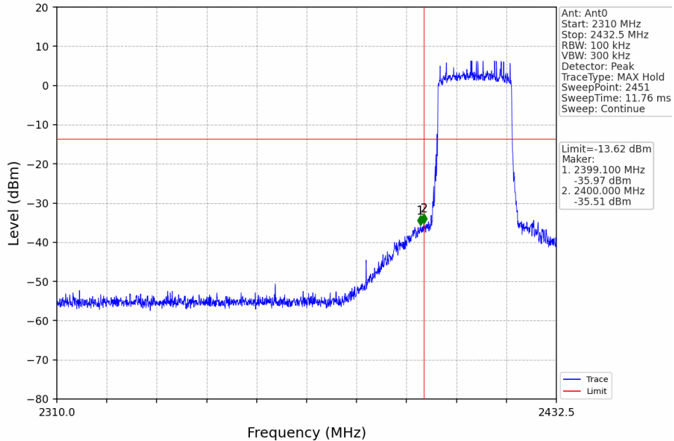
20M_LCH_2412.5MHz_Ant0_NTNV
