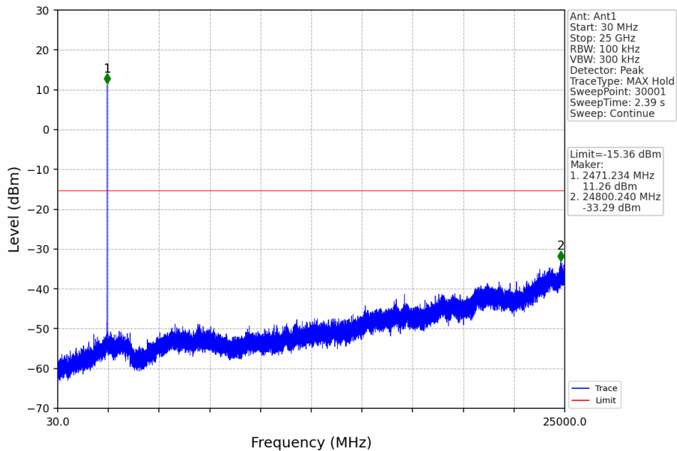
3M_HCH_2471.2MHz_Ant1_NTNV
