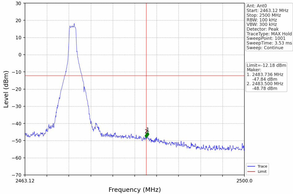
1.4M_HCH_2471.12MHz_Ant0_NTNV
