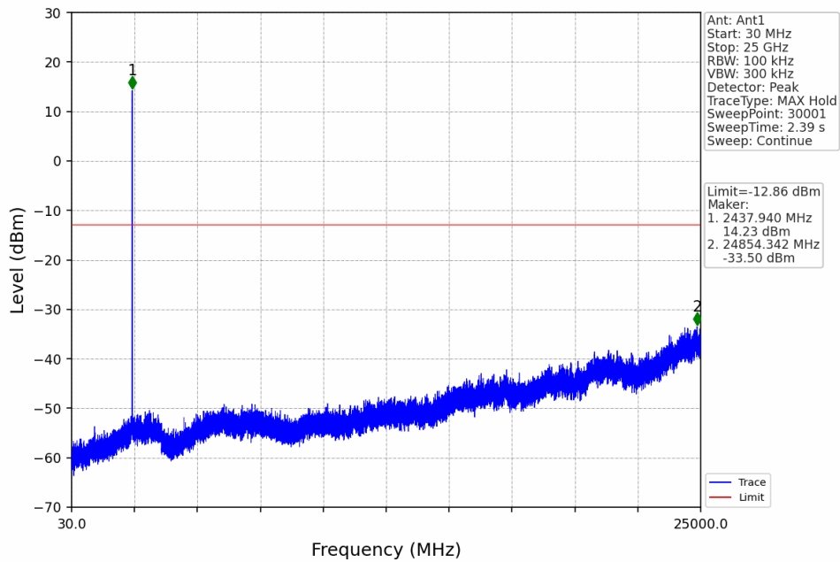
1.4M_MCH_2437.5MHz_Ant1_NTNV
