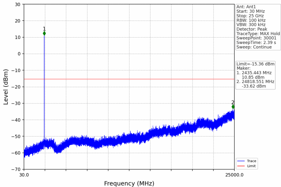
3M_MCH_2435.5MHz_Ant1_NTNV
