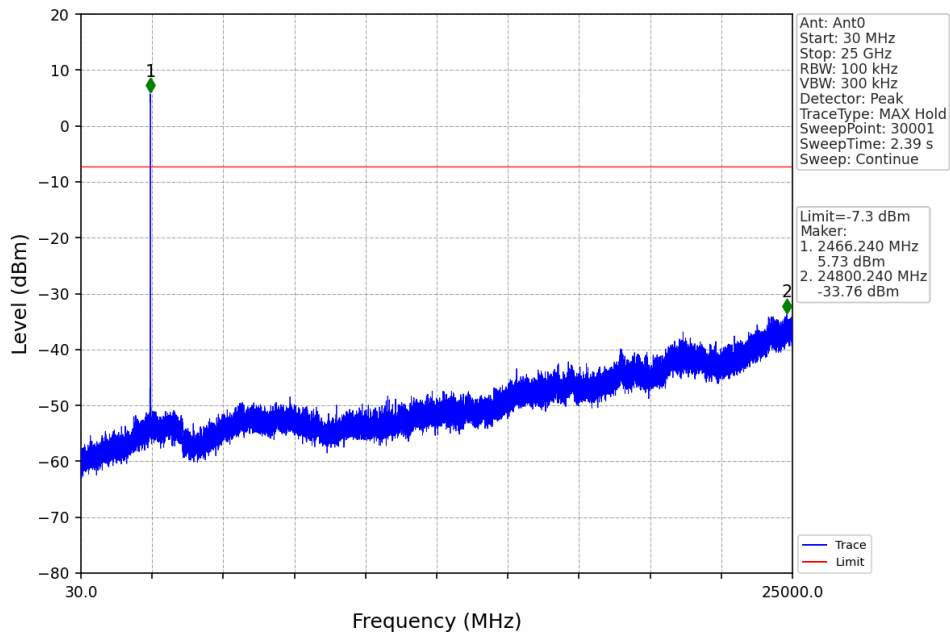
10M_HCH_2467.5MHz_Ant0_NTNV
