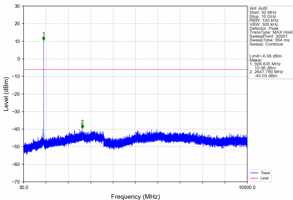
1.4M_HCH_927.2MHz_Ant0_NTNV
