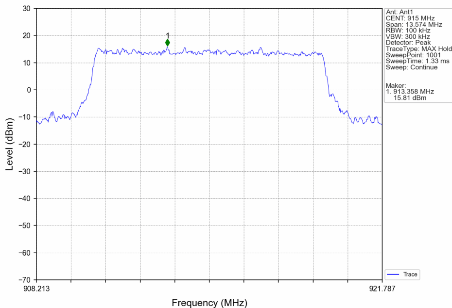
10M_MCH_915MHz_Ant1_NTNV
