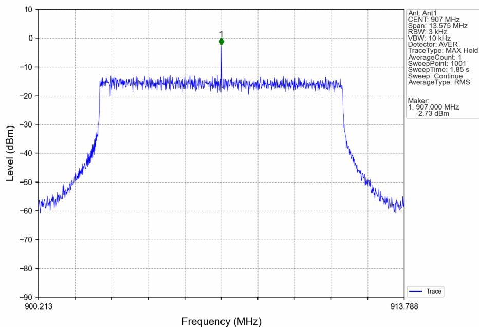
10M_LCH_907MHz_MIMO_NTNV
