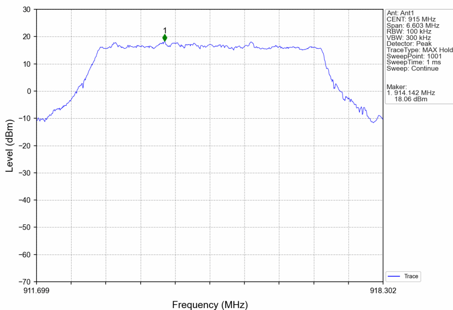
5M_MCH_915MHz_Ant1_NTNV
