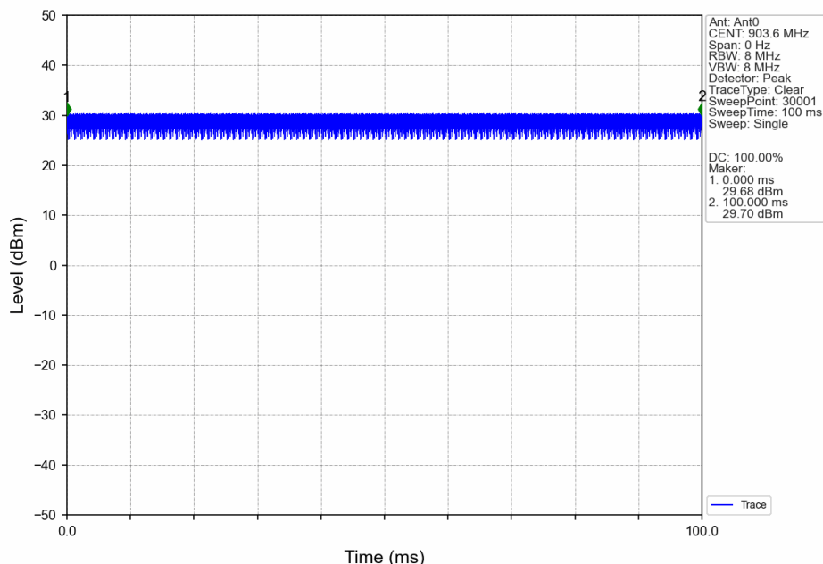
3M_LCH_903.6MHz_Ant0_NTNV
