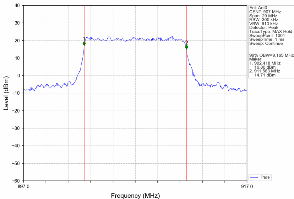
10M_LCH_907MHz_Ant0_NTNV
