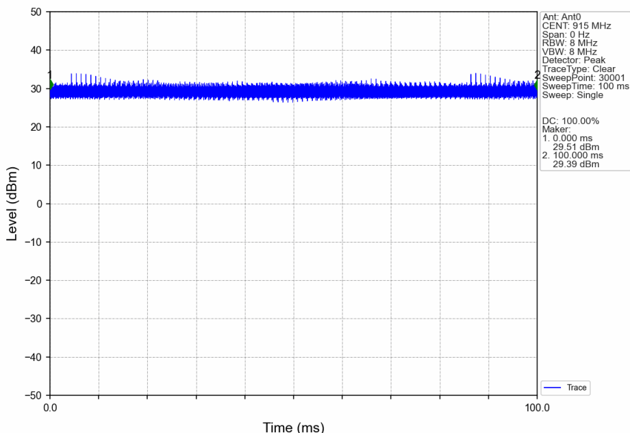
20M_MCH_915MHz_Ant0_NTNV
