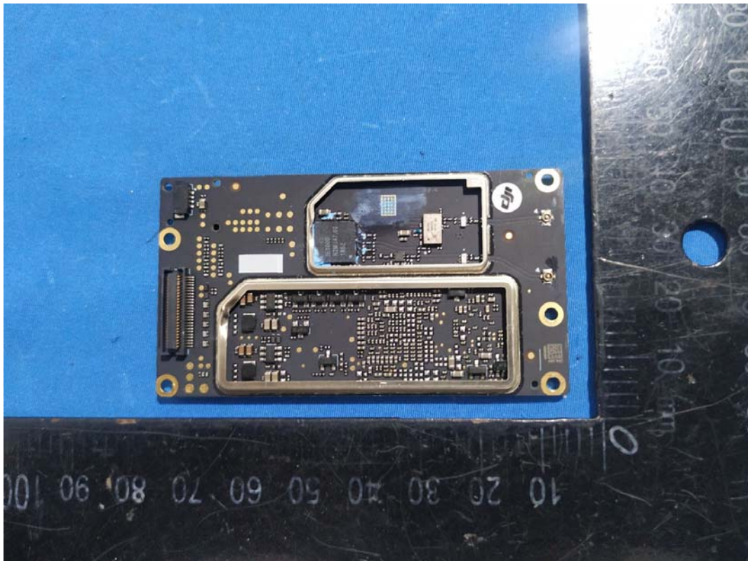
SDR Module
