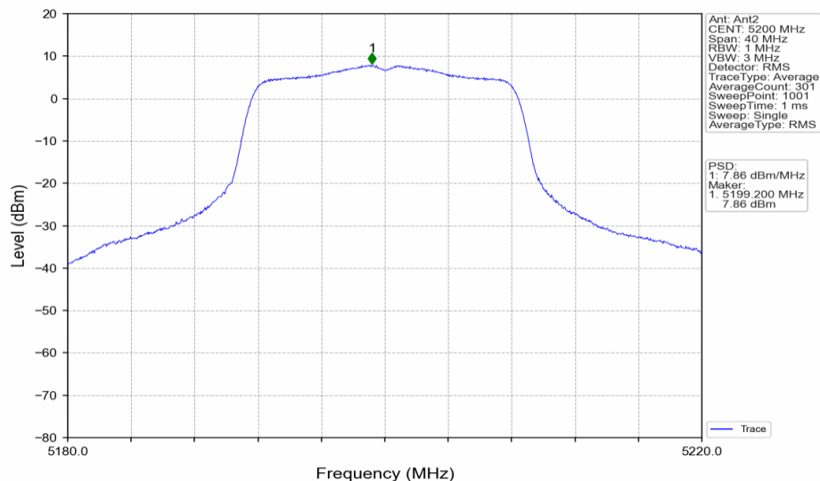
802.11a_MCH_5200MHz_Ant2_NTNV
