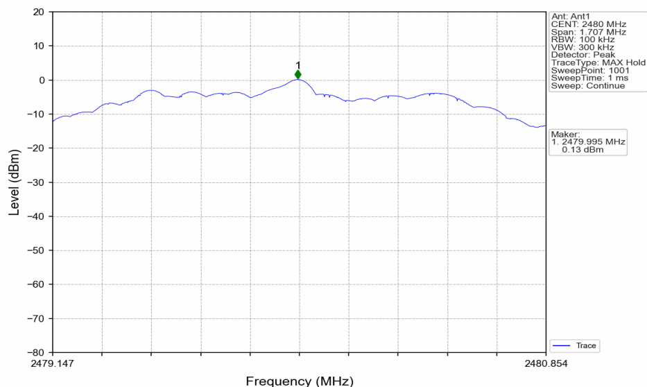
2M_HCH_2480MHz_Ant1_NTNV
