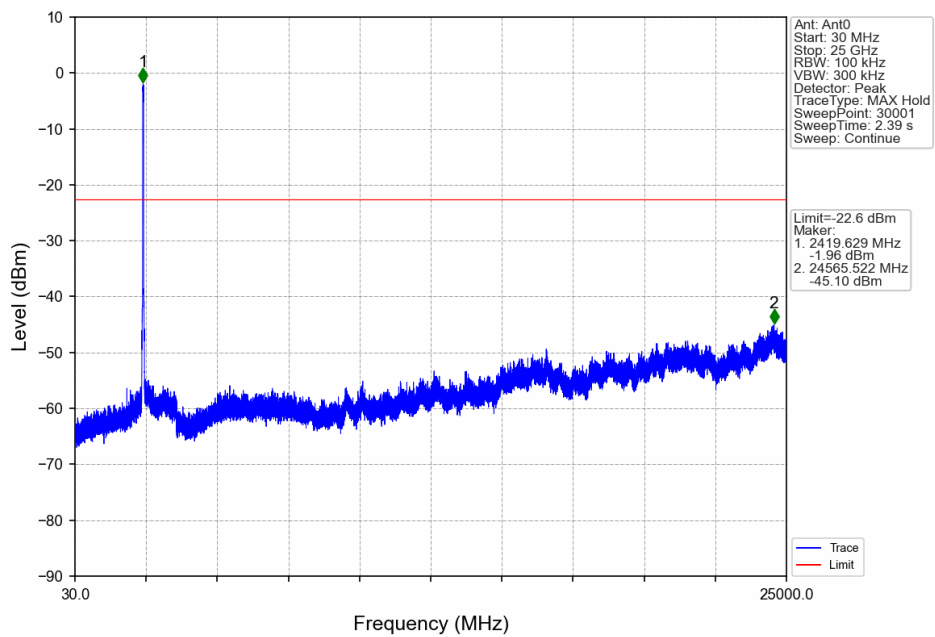
40MHz_LCH_2422.5MHz_Ant0_NTNV
