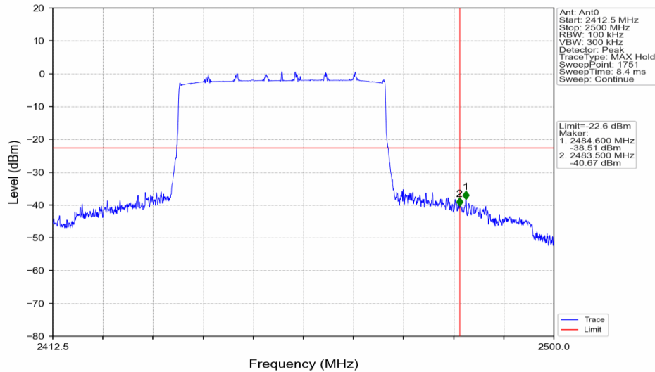
40MHz_HCH_2452.5MHz_Ant0_NTNV
