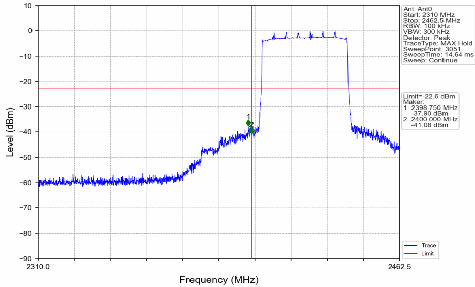
40MHz_LCH_2422.5MHz_Ant0_NTNV
