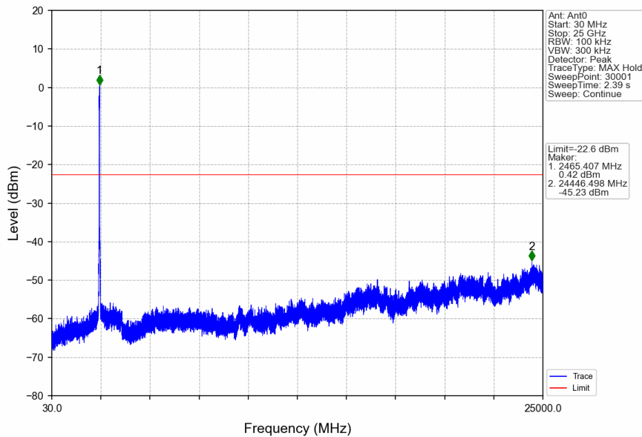
40MHz_HCH_2452.5MHz_Ant0_NTNV
