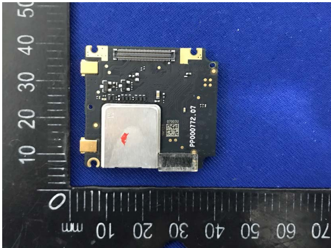
RF Module bottom
