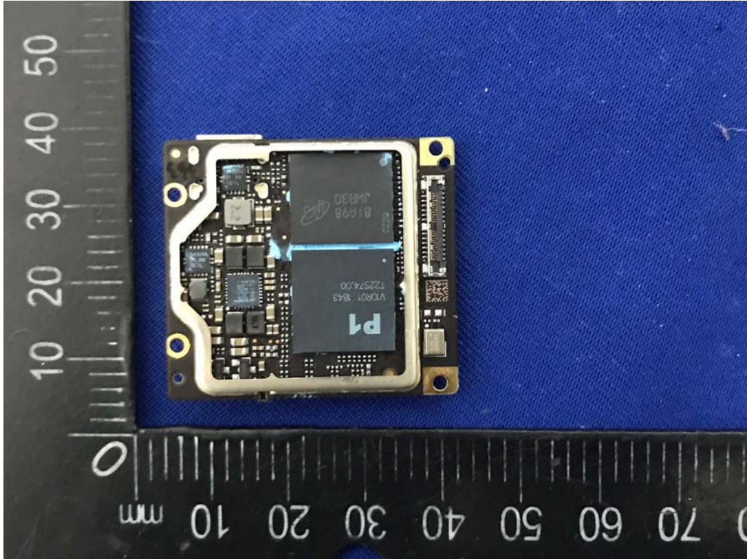
RF Module top
