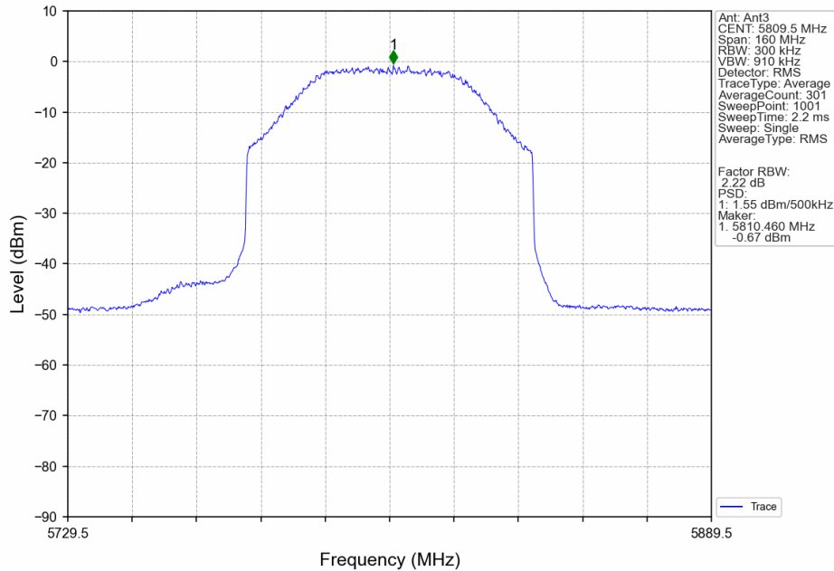
80M_HCH_5809.5MHz_MIMO_NTNV
