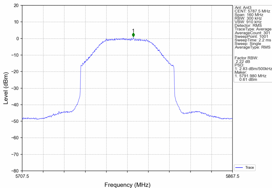
80M_MCH_5787.5MHz_Ant3_NTNV
