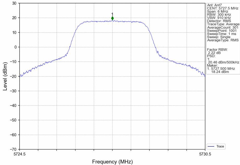
3M_LCH_5727.5MHz_MIMO_NTNV
