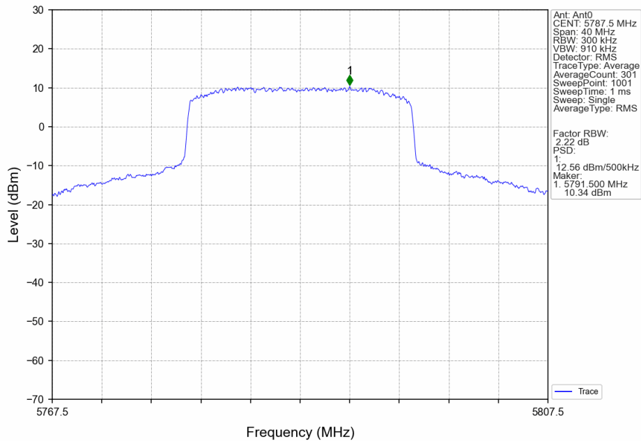
20M_MCH_5787.5MHz_Ant0_NTNV
