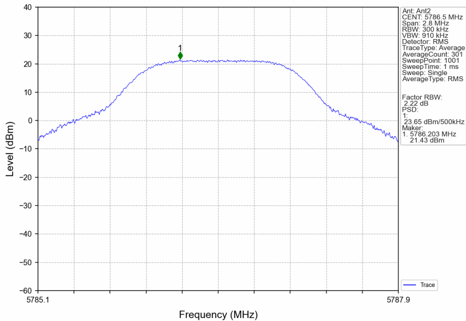
1.4M_MCH_5786.5MHz_Ant2_NTNV
