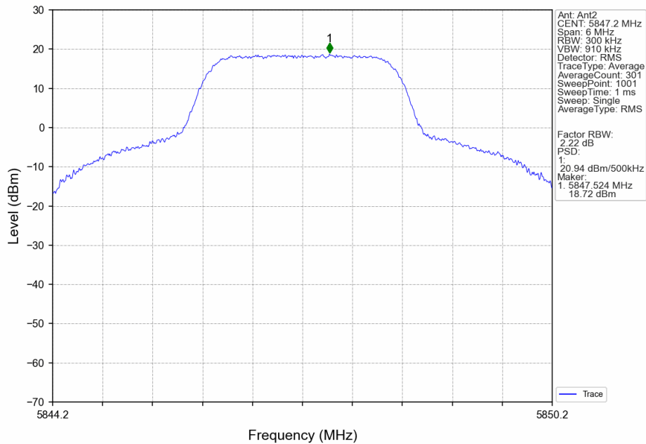
3M_HCH_5847.2MHz_Ant2_NTNV
