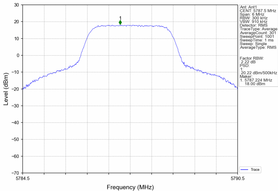
3M_MCH_5787.5MHz_Ant1_NTNV
