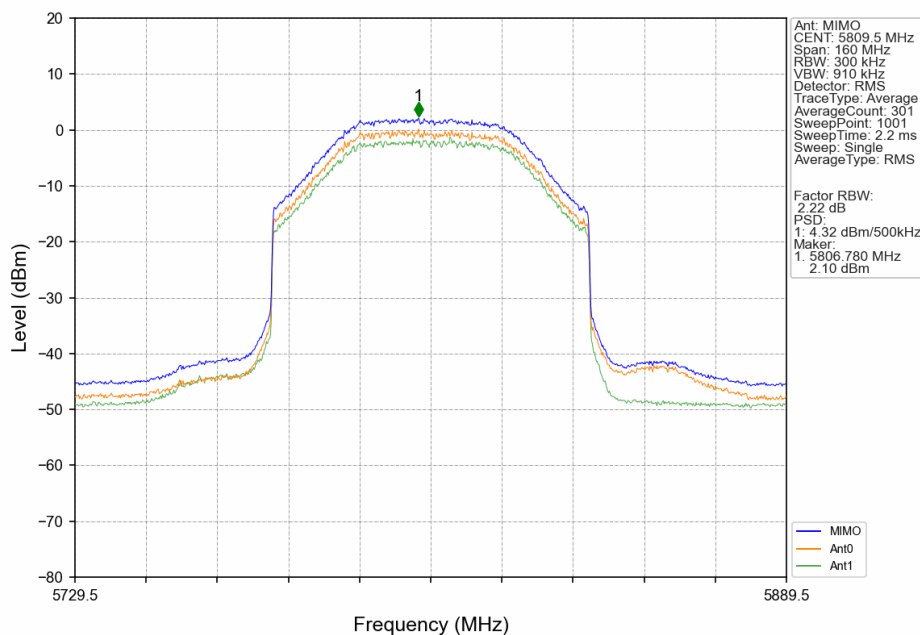
80M_HCH_5809.5MHz_MIMO_NTNV
