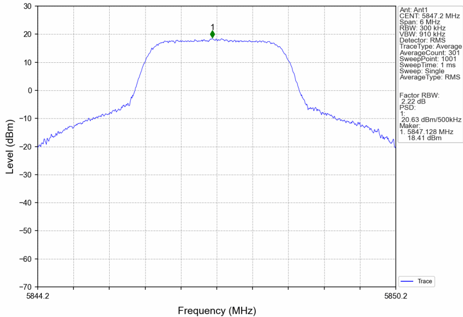
3M_HCH_5847.2MHz_MIMO_NTNV
