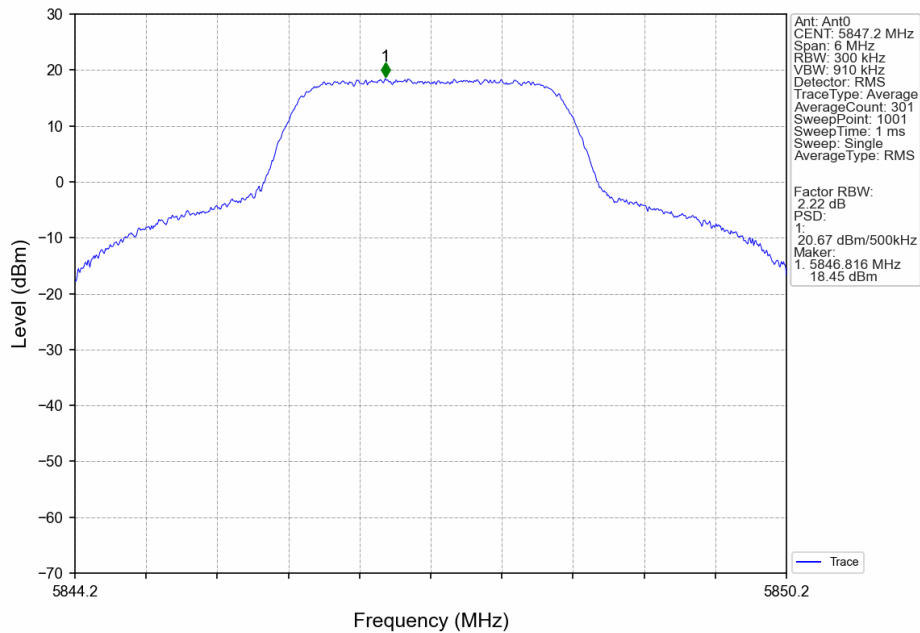
3M_HCH_5847.2MHz_Ant0_NTNV
