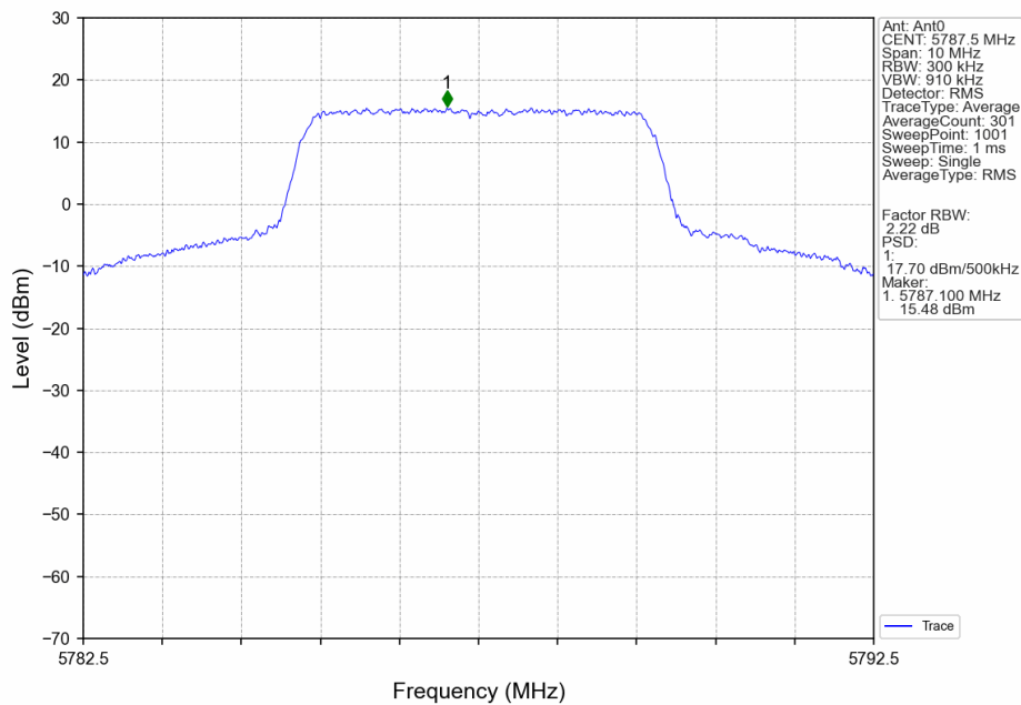
5M_MCH_5787.5MHz_Ant0_NTNV
