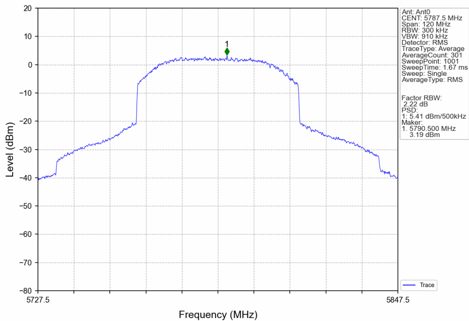
60M_MCH_5787.5MHz_Ant0_NTNV
