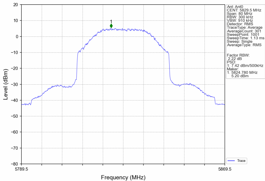
40M_HCH_5829.5MHz_Ant0_NTNV
