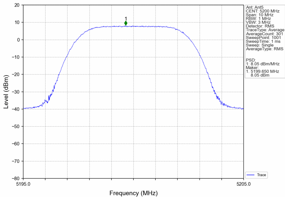
5M_MCH_5200MHz_Ant5_NTNV
