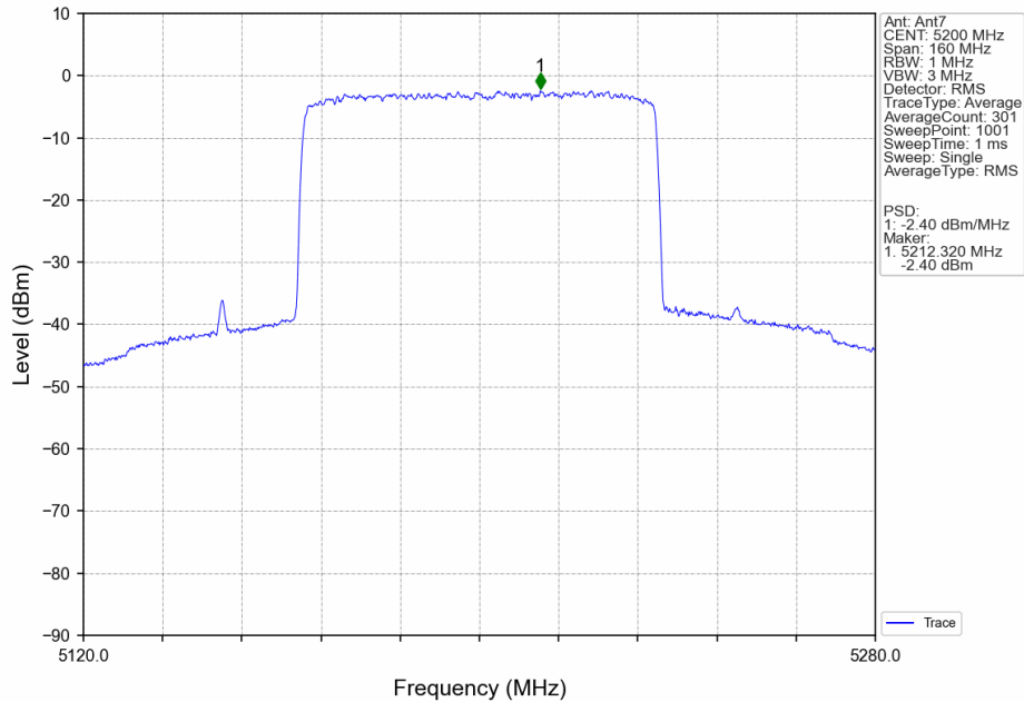
80M_MCH_5200MHz_MIMO_NTNV
