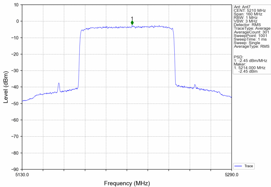
80M_HCH_5210MHz_Ant7_NTNV
