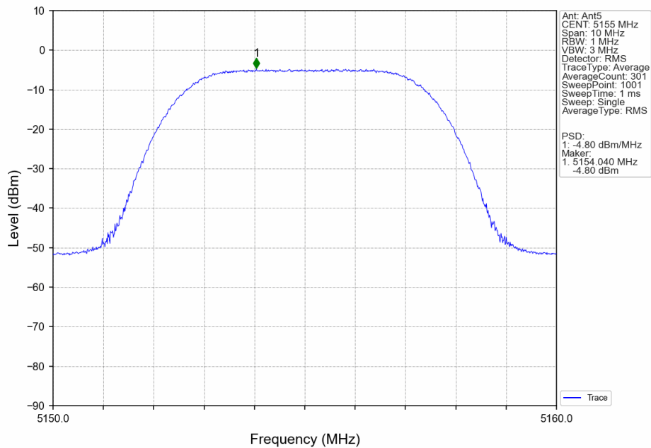
5M_LCH_5155MHz_MIMO_NTNV
