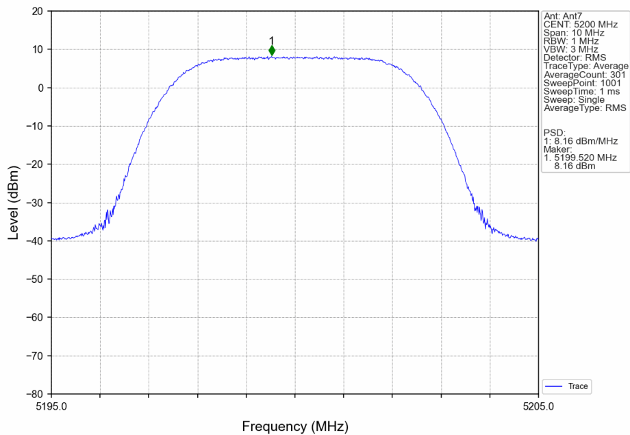
5M_MCH_5200MHz_Ant7_NTNV
