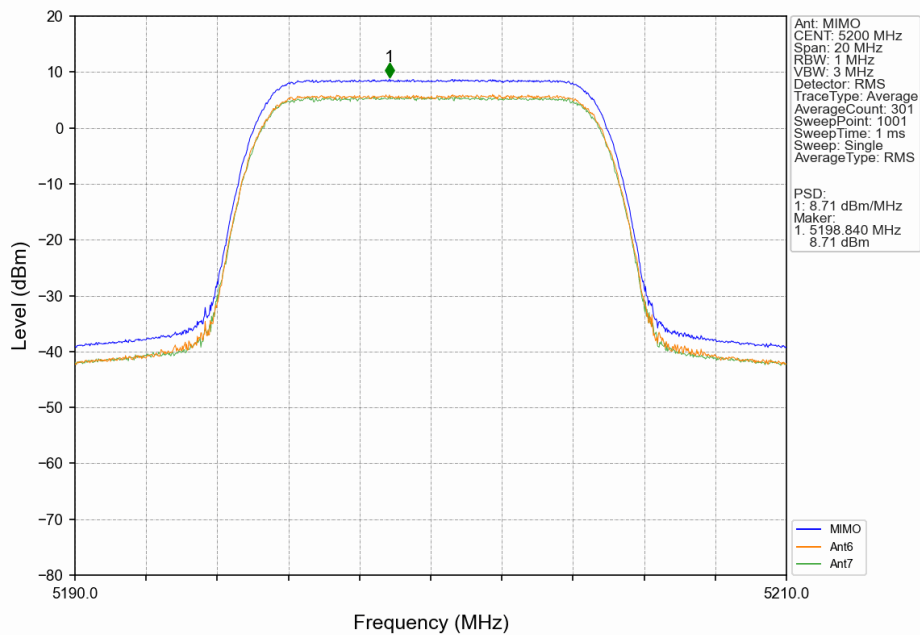
10M_MCH_5200MHz_MIMO_NTNV
