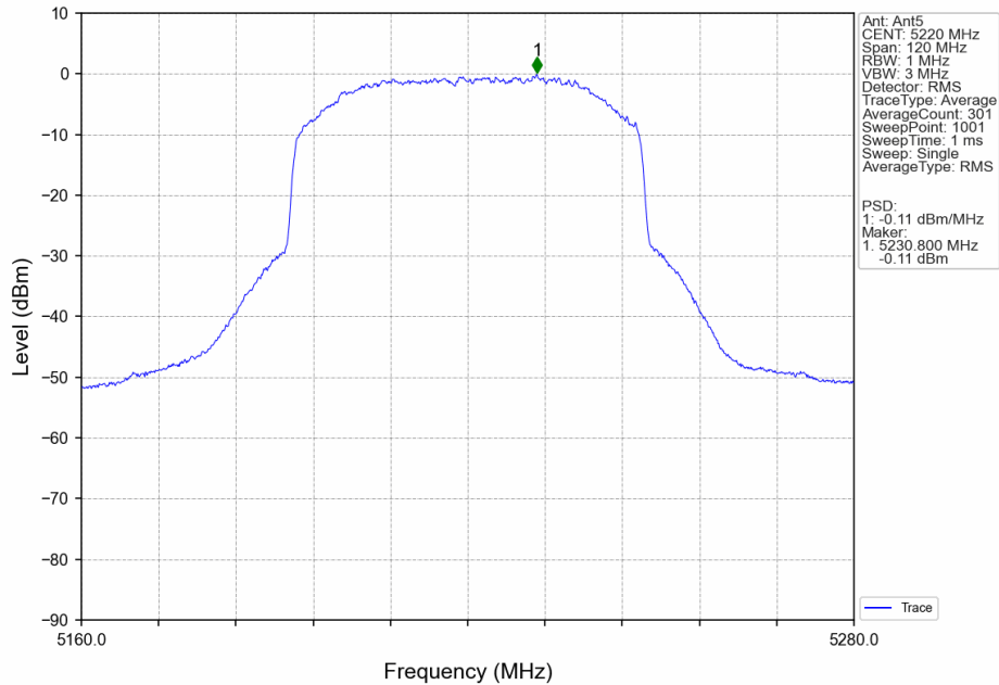
60M_HCH_5220MHz_MIMO_NTNV
