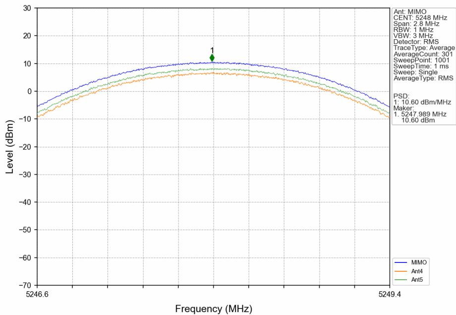
1.4M_HCH_5248MHz_MIMO_NTNV
