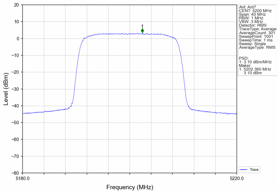
20M_MCH_5200MHz_Ant7_NTNV
