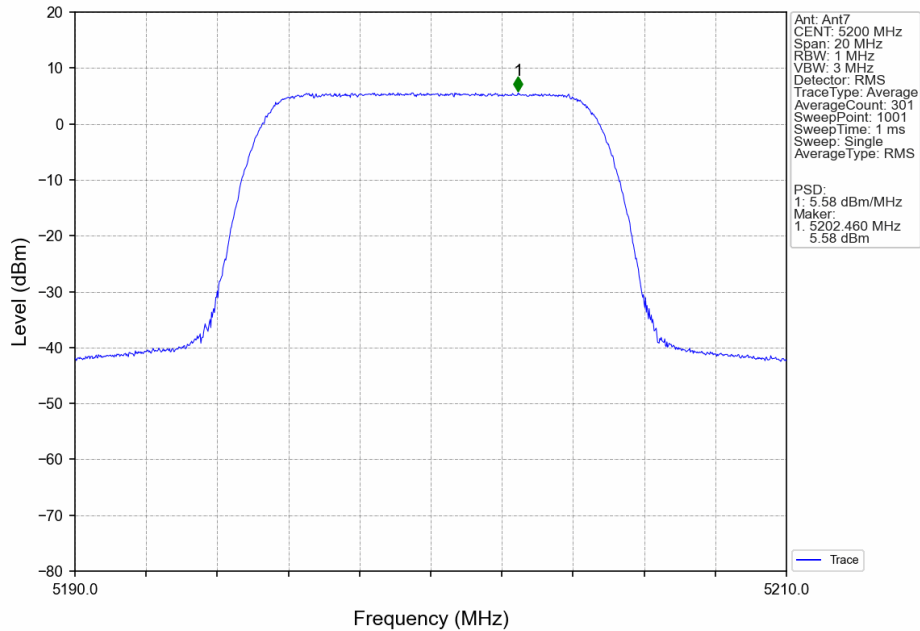
10M_MCH_5200MHz_MIMO_NTNV
