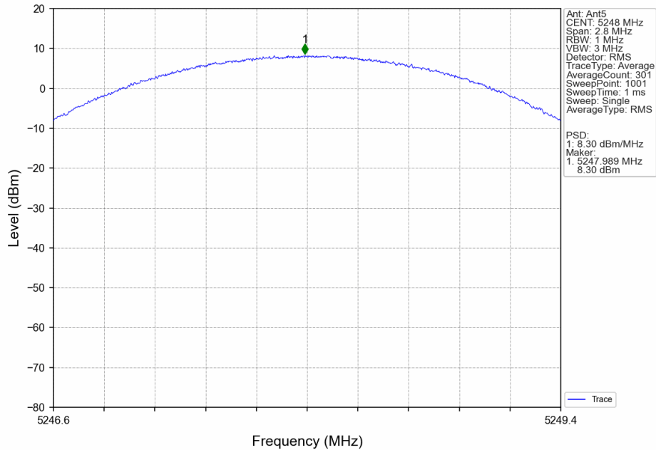
1.4M_HCH_5248MHz_MIMO_NTNV
