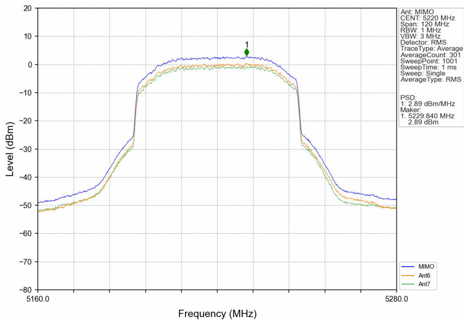
60M_HCH_5220MHz_MIMO_NTNV
