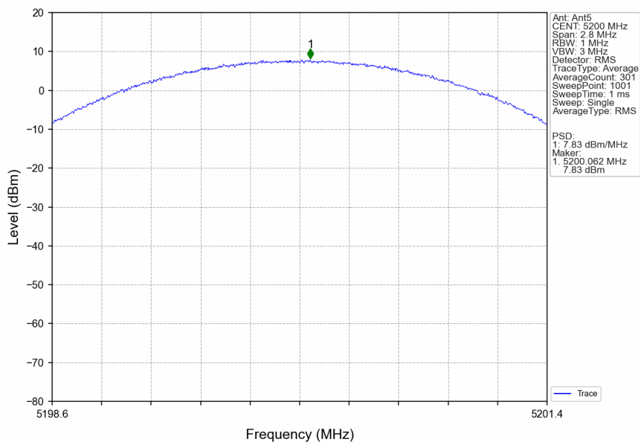
1.4M_MCH_5200MHz_Ant5_NTNV
