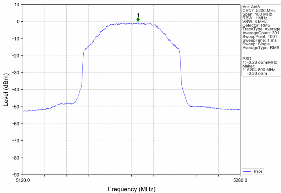
80M_MCH_5200MHz_MIMO_NTNV
