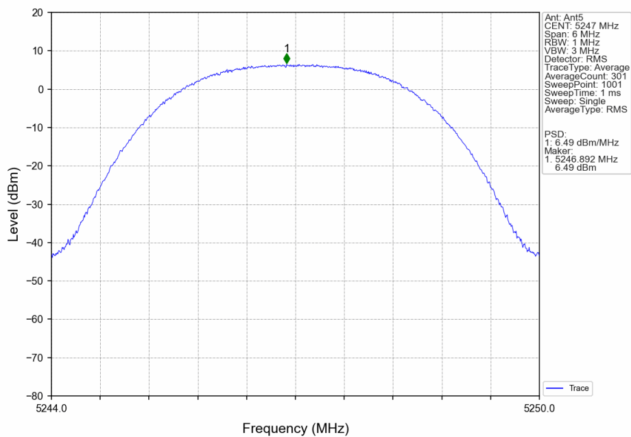
3M_HCH_5247MHz_Ant5_NTNV
