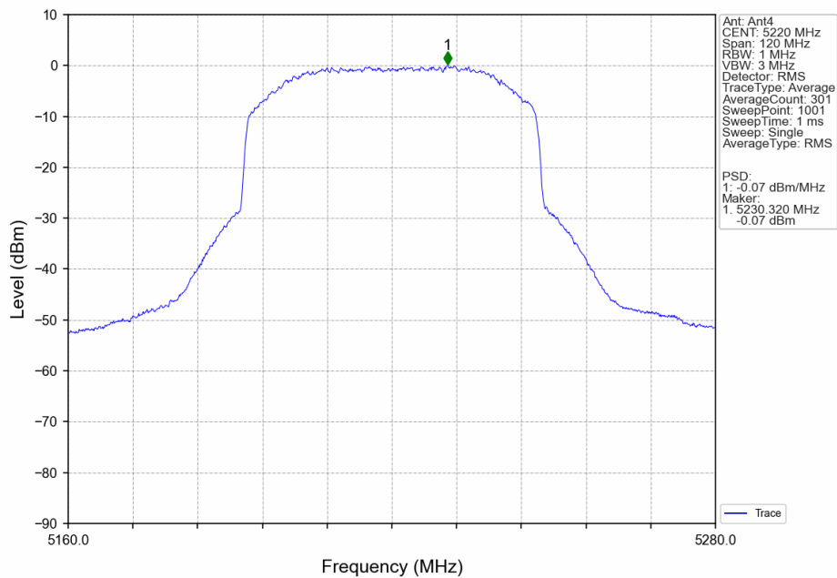
60M_HCH_5220MHz_Ant4_NTNV
