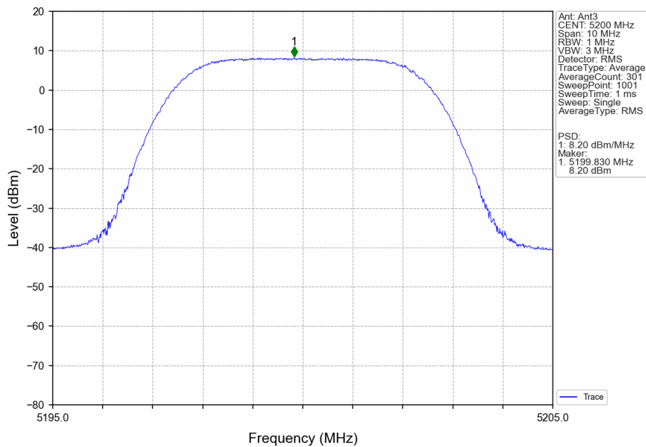
5M_MCH_5200MHz_Ant3_NTNV
