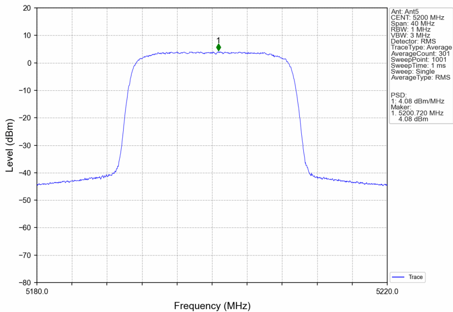
20M_MCH_5200MHz_Ant5_NTNV
