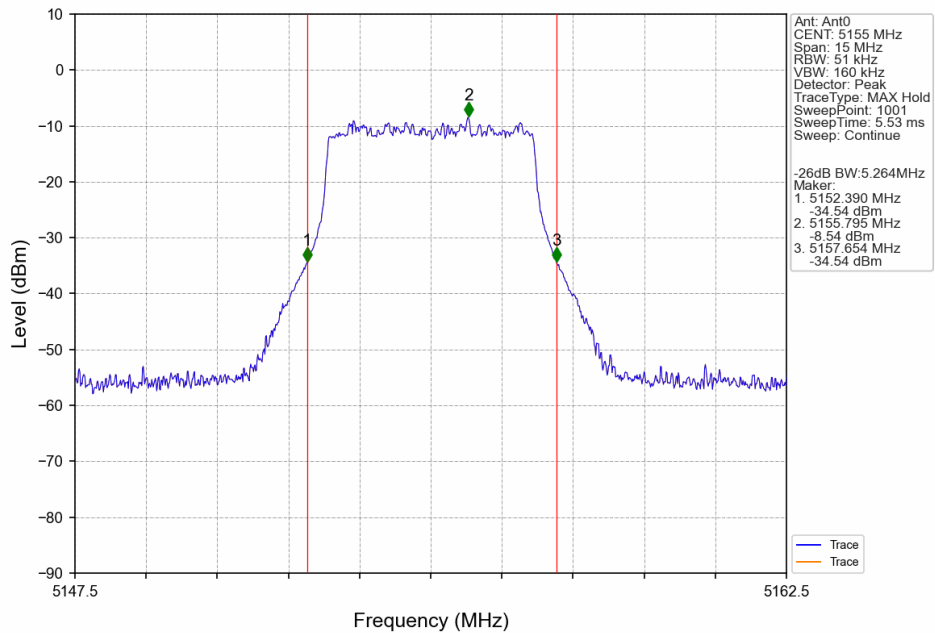
5M_LCH_5155MHz_Ant0_NTNV
