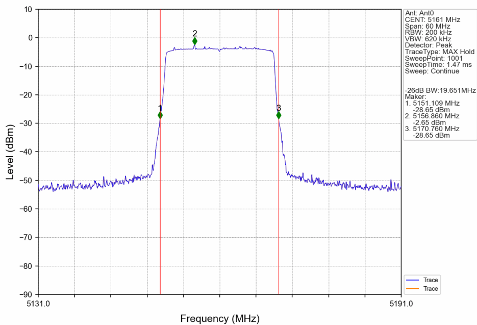
20M_LCH_5161MHz_Ant0_NTNV
