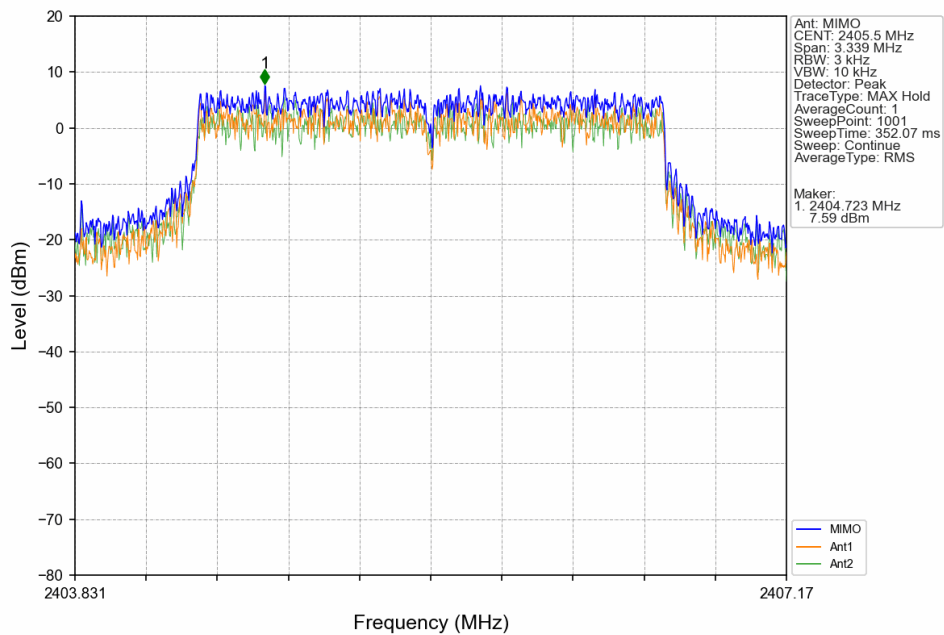
3M_LCH_2405.5MHz_MIMO_NTNV
