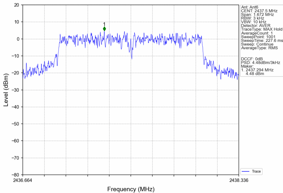
1.4M_MCH_2437.5MHz_Ant6_NTNV
