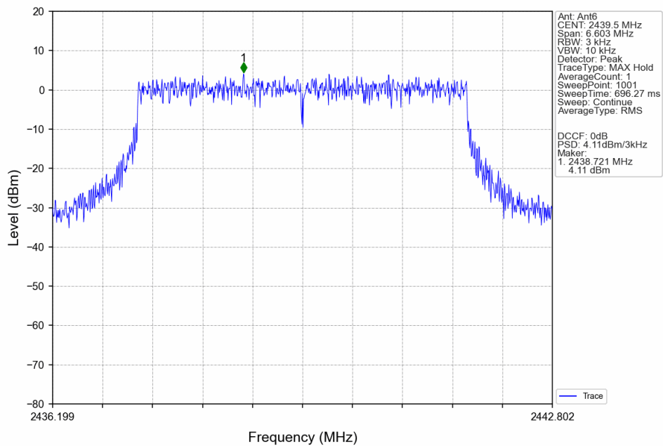
5M_MCH_2439.5MHz_Ant6_NTNV
