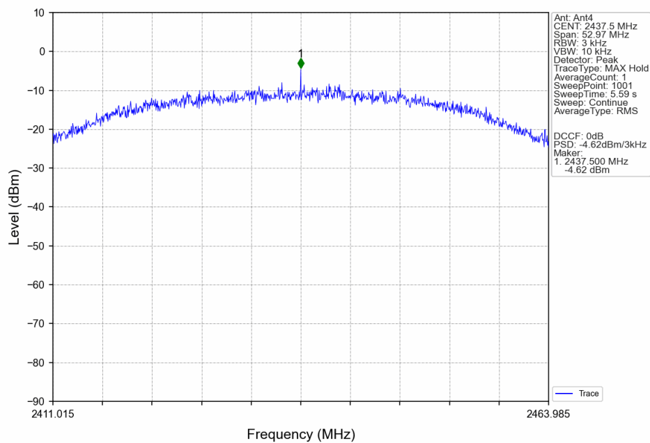
60M_MCH_2437.5MHz_Ant4_NTNV
