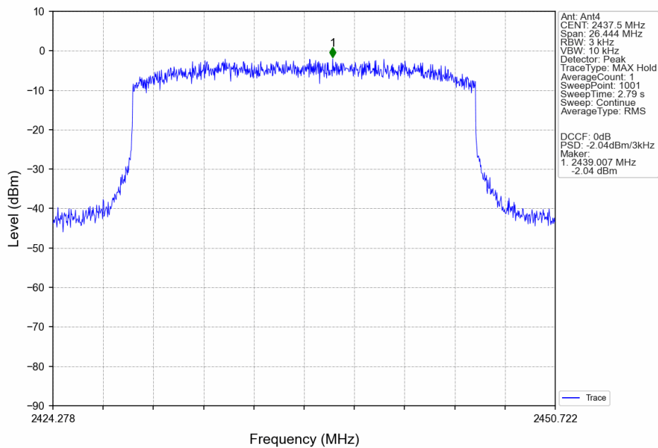
20M_MCH_2437.5MHz_Ant4_NTNV
