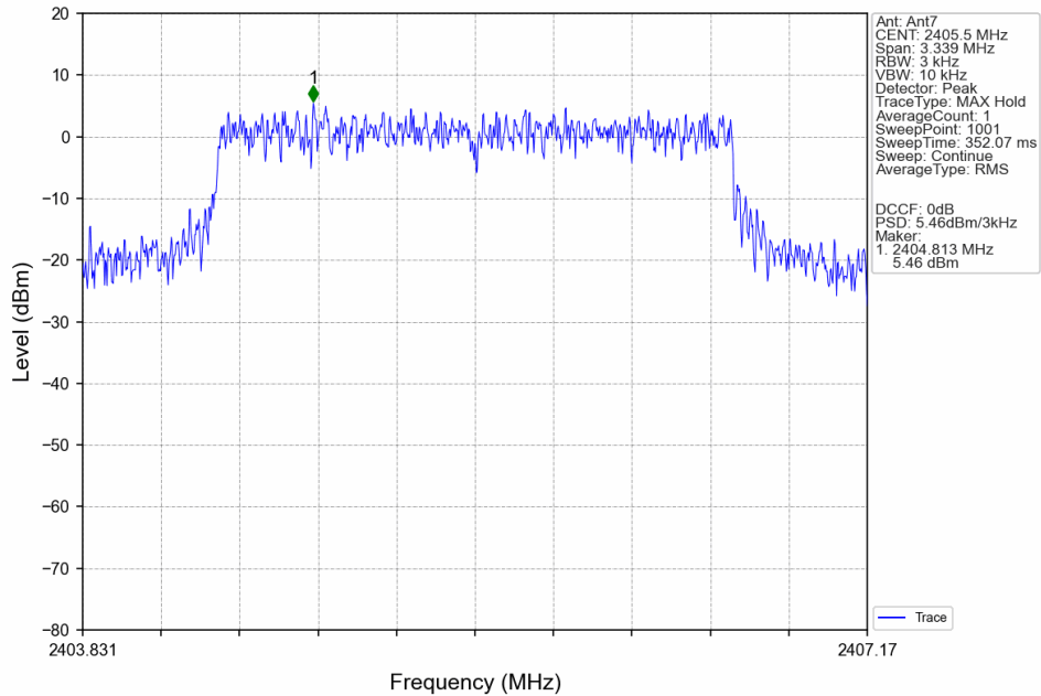
3M_LCH_2405.5MHz_MIMO_NTNV
