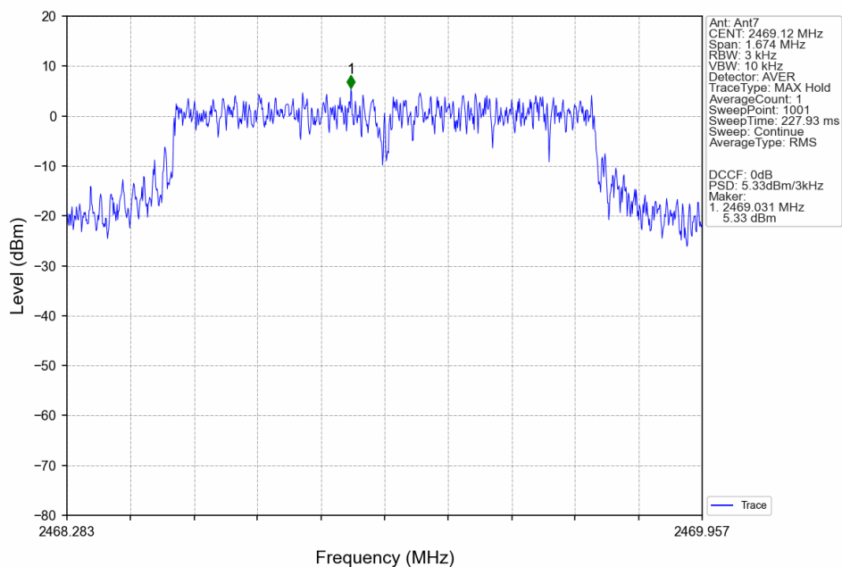
1.4M_HCH_2469.12MHz_Ant7_NTNV
