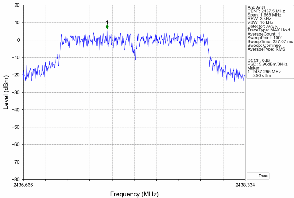
1.4M_MCH_2437.5MHz_Ant4_NTNV
