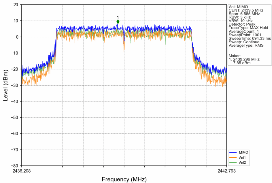
5M_MCH_2439.5MHz_MIMO_NTNV
