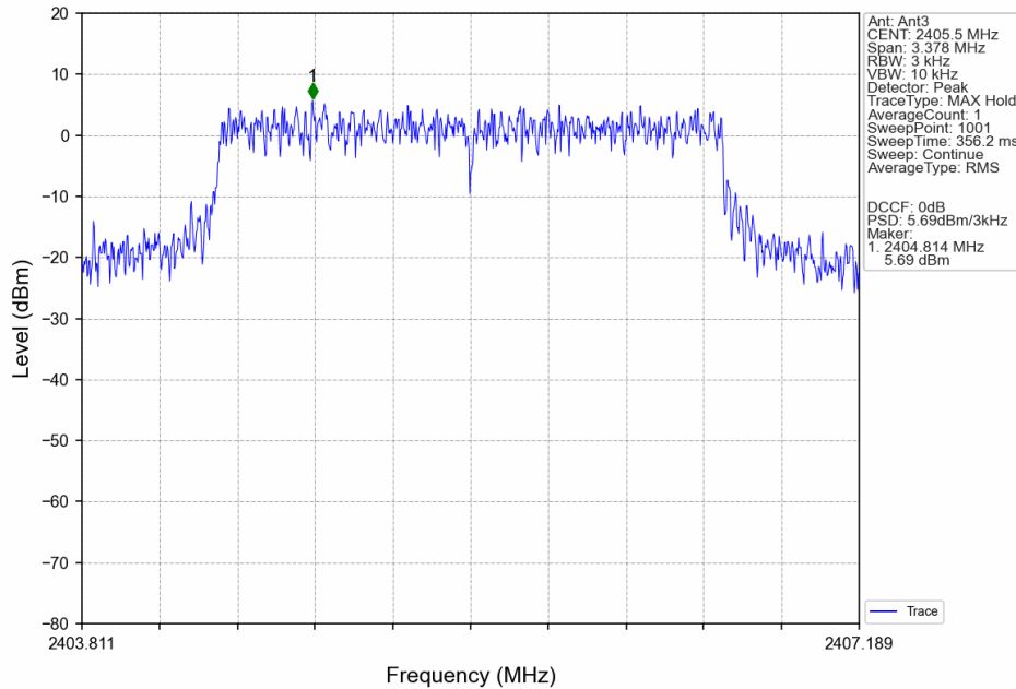
3M_LCH_2405.5MHz_MIMO_NTNV
