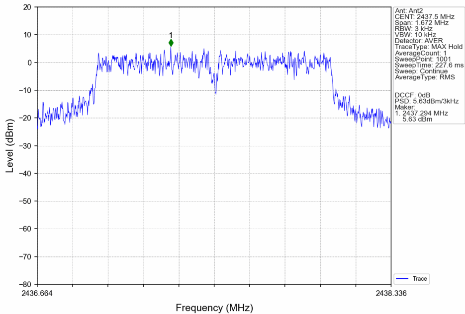
1.4M_MCH_2437.5MHz_Ant2_NTNV
