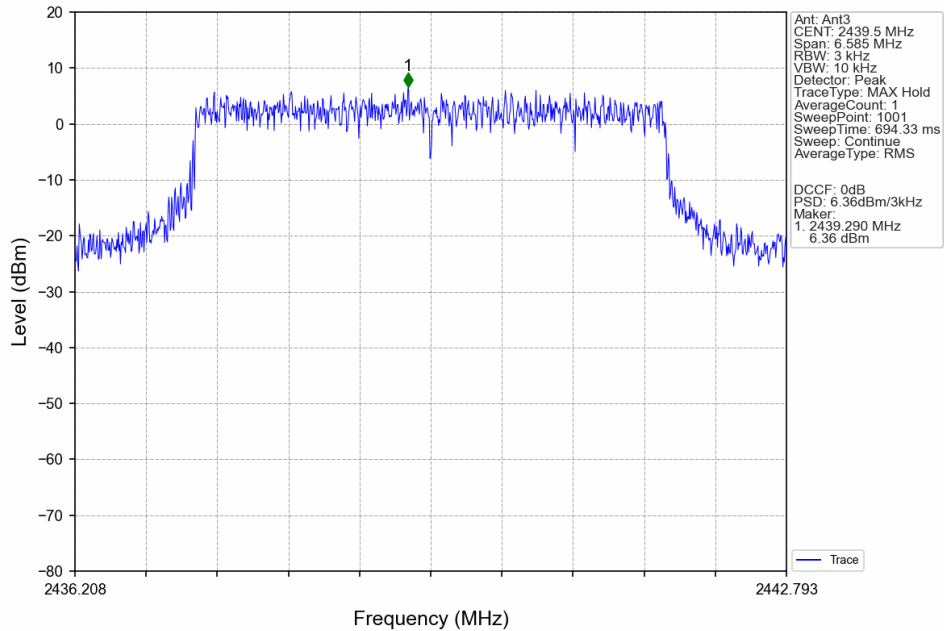
5M_MCH_2439.5MHz_MIMO_NTNV
