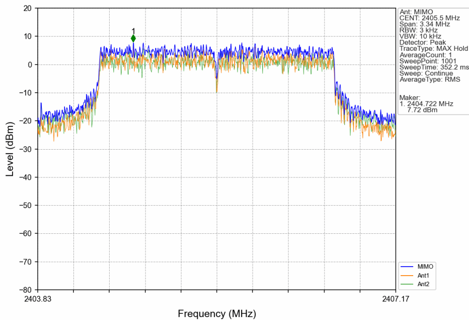
3M_LCH_2405.5MHz_MIMO_NTNV
