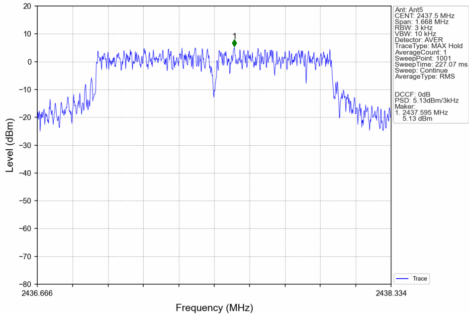
1.4M_MCH_2437.5MHz_MIMO_NTNV
