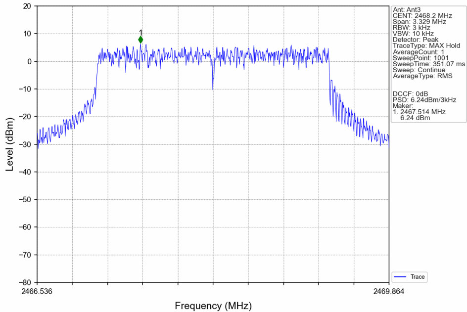
3M_HCH_2468.2MHz_MIMO_NTNV
