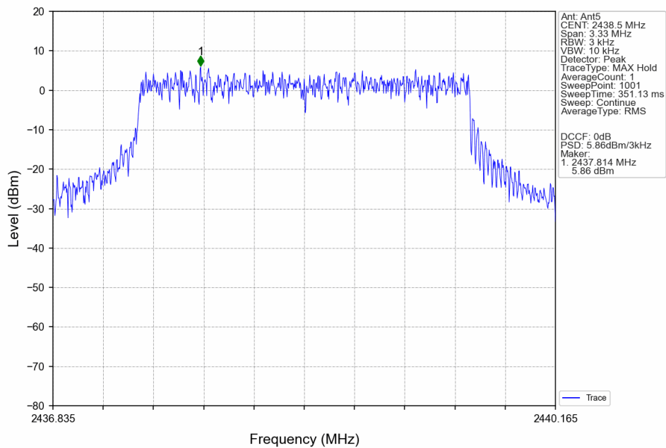
3M_MCH_2438.5MHz_Ant5_NTNV
