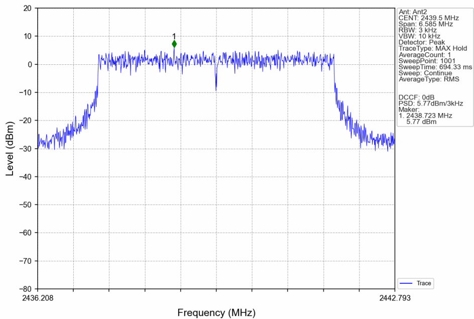
5M_MCH_2439.5MHz_Ant2_NTNV
