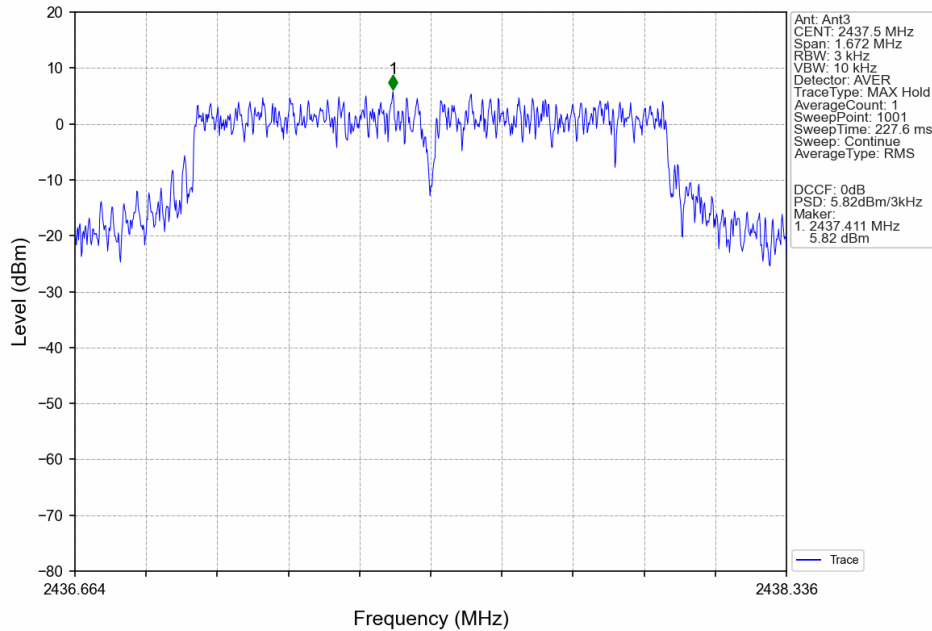
1.4M_MCH_2437.5MHz_MIMO_NTNV
