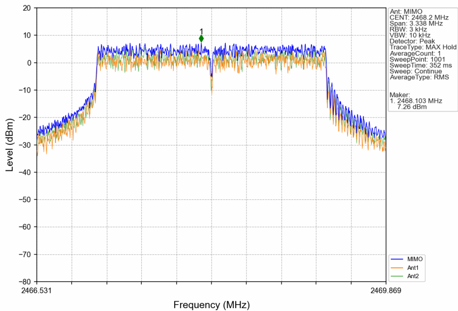
3M_HCH_2468.2MHz_MIMO_NTNV
