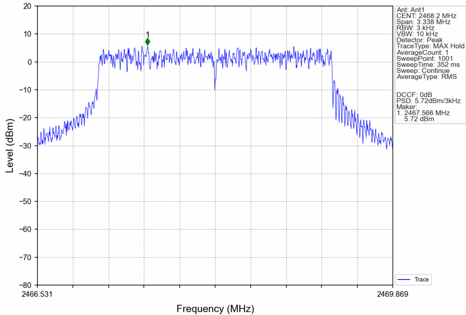
3M_HCH_2468.2MHz_MIMO_NTNV
