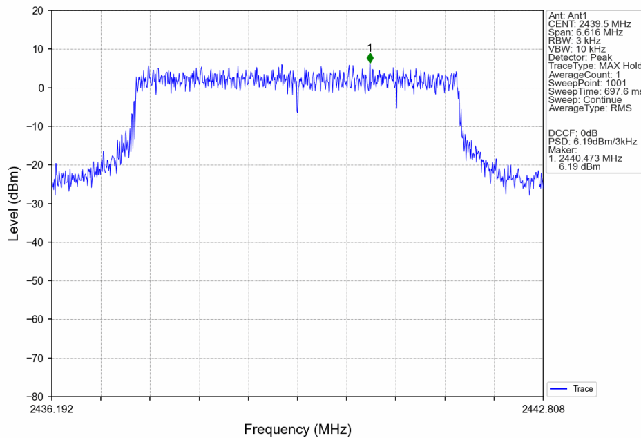
5M_MCH_2439.5MHz_MIMO_NTNV
