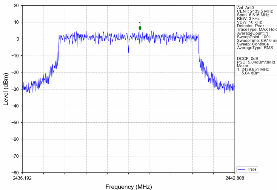
5M_MCH_2439.5MHz_Ant0_NTNV
