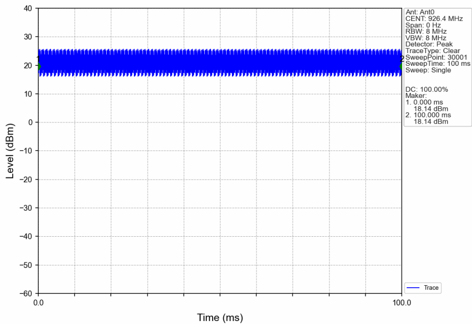
3M_HCH_926.4MHz_Ant0_NTNV
