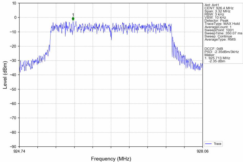
3M_HCH_926.4MHz_MIMO_NTNV
