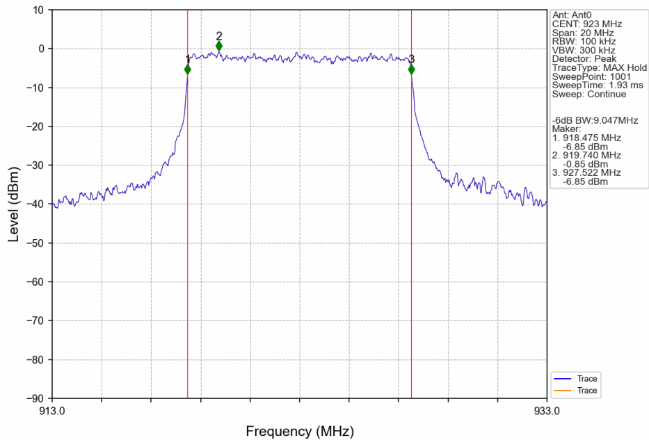
10M_HCH_923MHz_Ant0_NTNV
