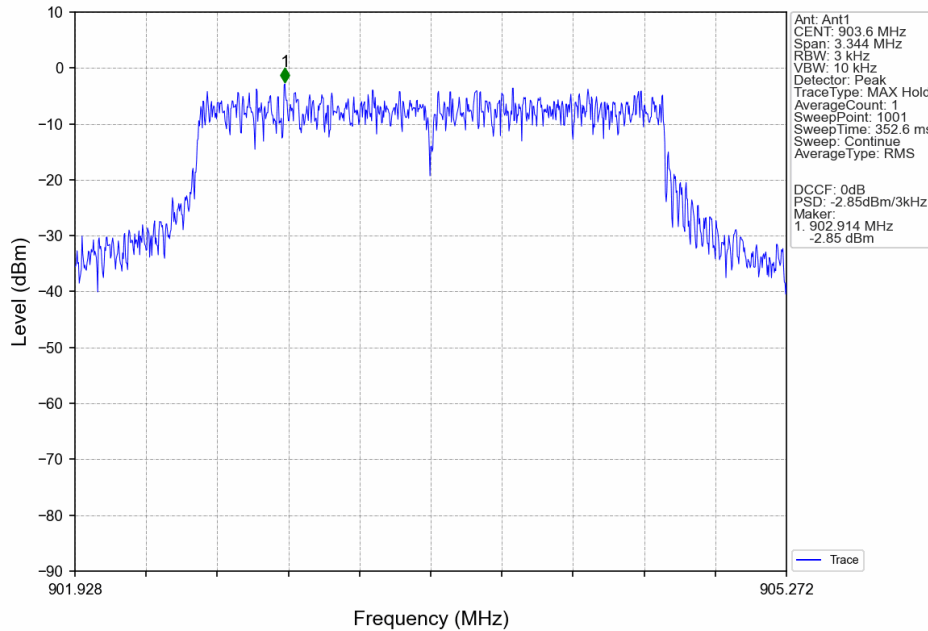
3M_LCH_903.6MHz_MIMO_NTNV
