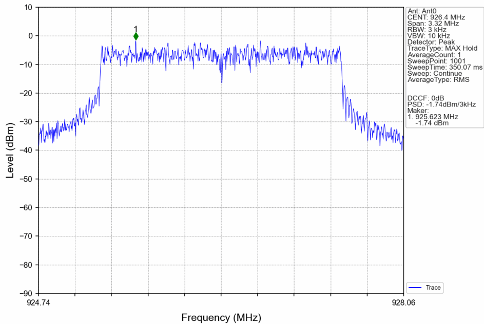
3M_HCH_926.4MHz_Ant0_NTNV
