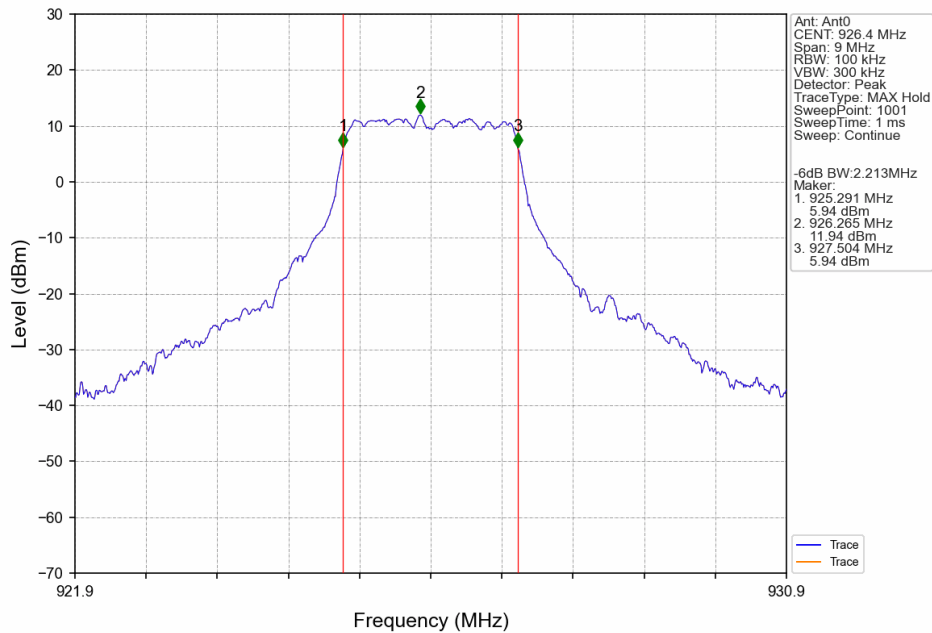
3M_HCH_926.4MHz_Ant0_NTNV
