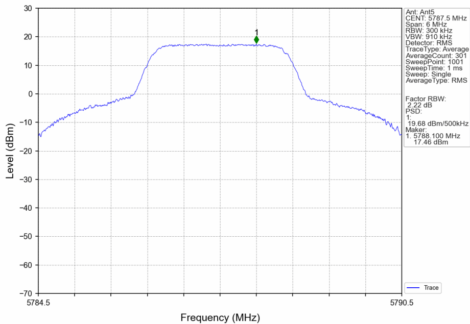
3M_MCH_5787.5MHz_Ant5_NTNV
