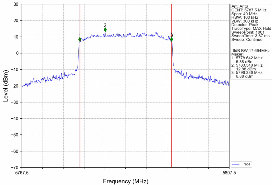
20M_MCH_5787.5MHz_Ant6_NTNV
