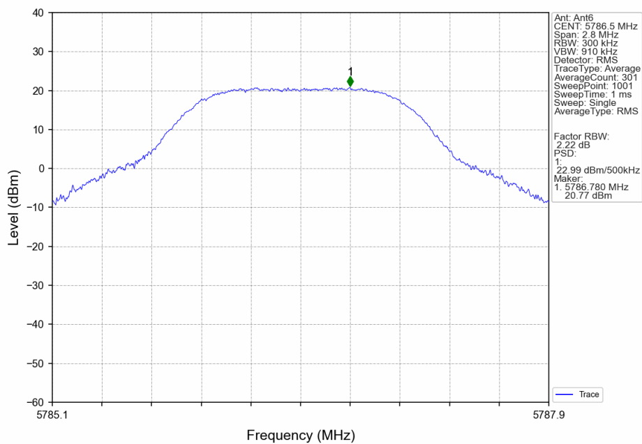
1.4M_MCH_5786.5MHz_Ant6_NTNV
