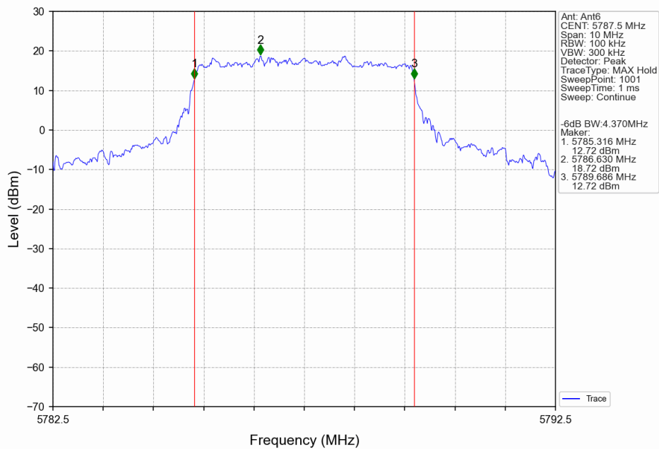
5M_MCH_5787.5MHz_Ant6_NTNV
