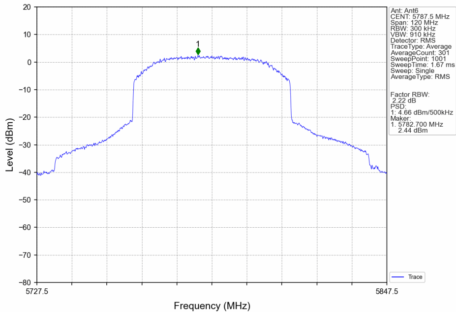
60M_MCH_5787.5MHz_Ant6_NTNV
