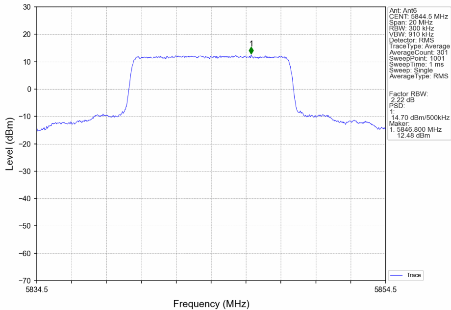
10M_HCH_5844.5MHz_Ant6_NTNV
