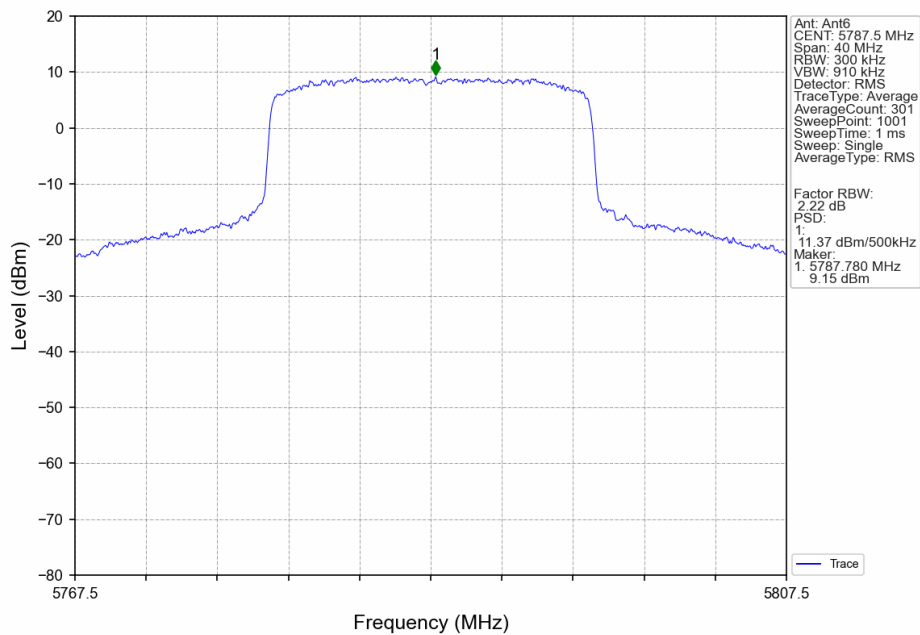
20M_MCH_5787.5MHz_Ant6_NTNV
