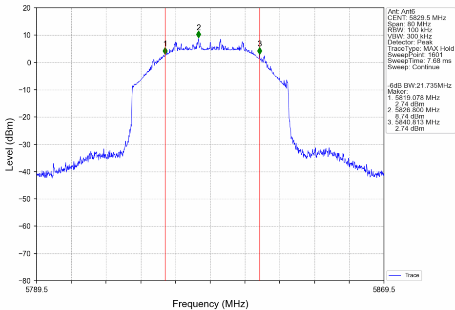
40M_HCH_5829.5MHz_Ant6_NTNV
