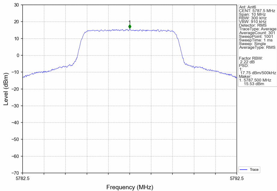
5M_MCH_5787.5MHz_Ant6_NTNV
