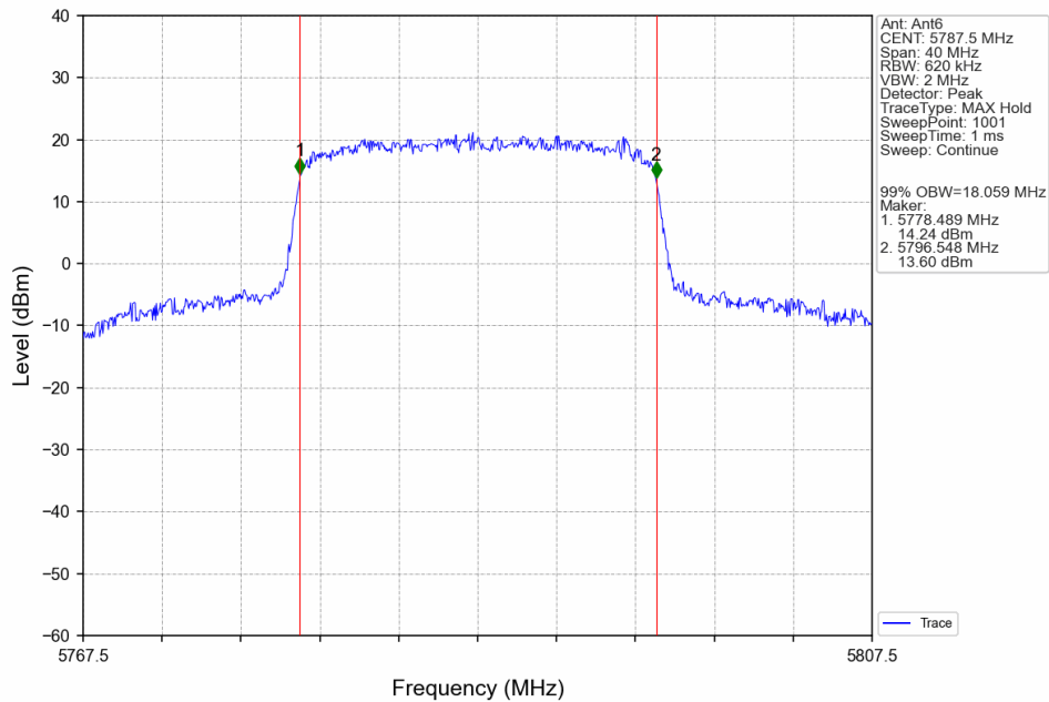
20M_MCH_5787.5MHz_Ant6_NTNV
