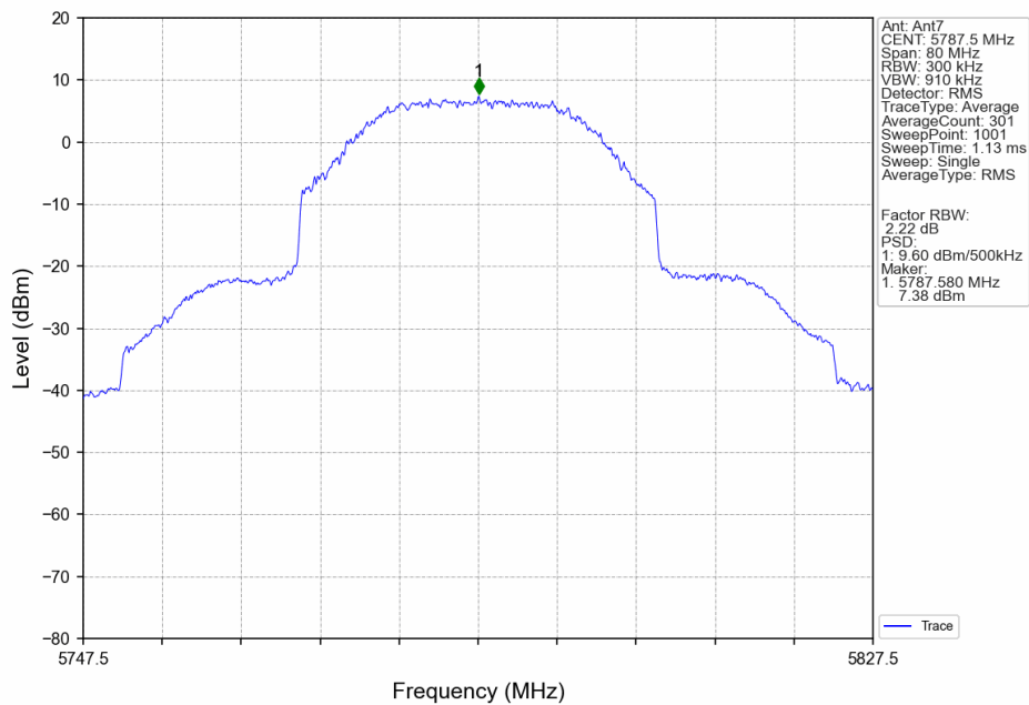
40M_MCH_5787.5MHz_Ant7_NTNV
