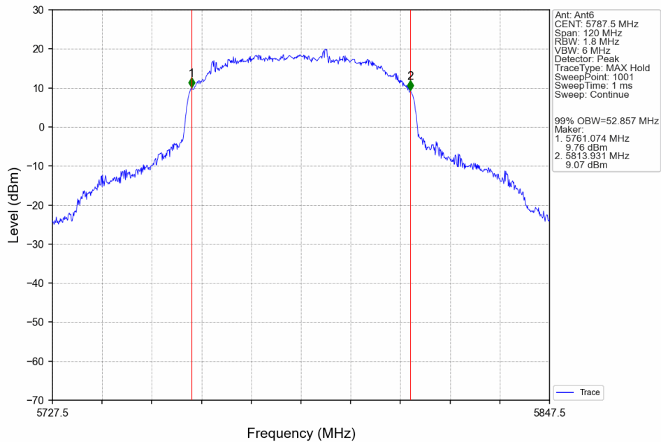
60M_MCH_5787.5MHz_Ant6_NTNV
