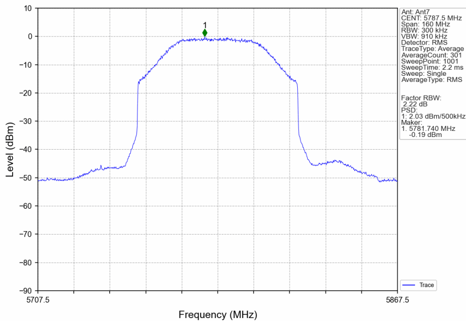
80M_MCH_5787.5MHz_Ant7_NTNV
