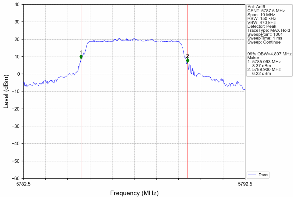
5M_MCH_5787.5MHz_Ant6_NTNV
