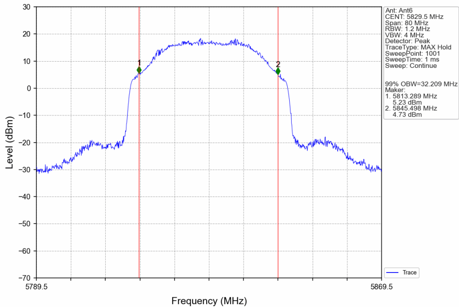
40M_HCH_5829.5MHz_Ant6_NTNV
