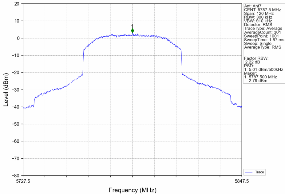
60M_MCH_5787.5MHz_MIMO_NTNV
