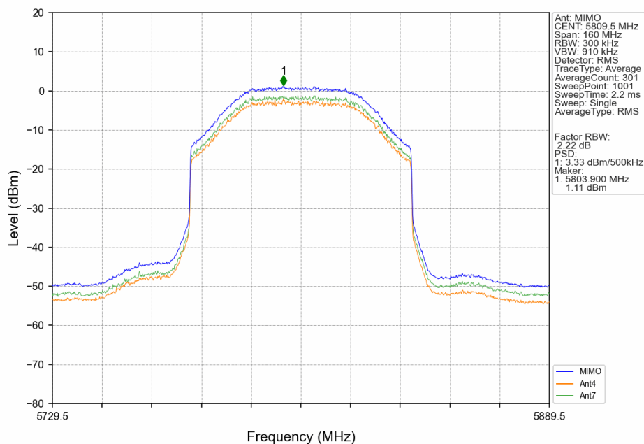
80M_HCH_5809.5MHz_MIMO_NTNV
