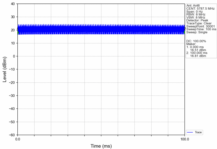
60M_MCH_5787.5MHz_Ant6_NTNV
