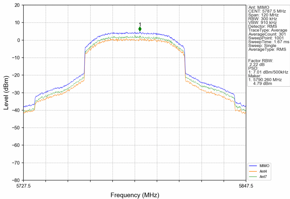
60M_MCH_5787.5MHz_MIMO_NTNV
