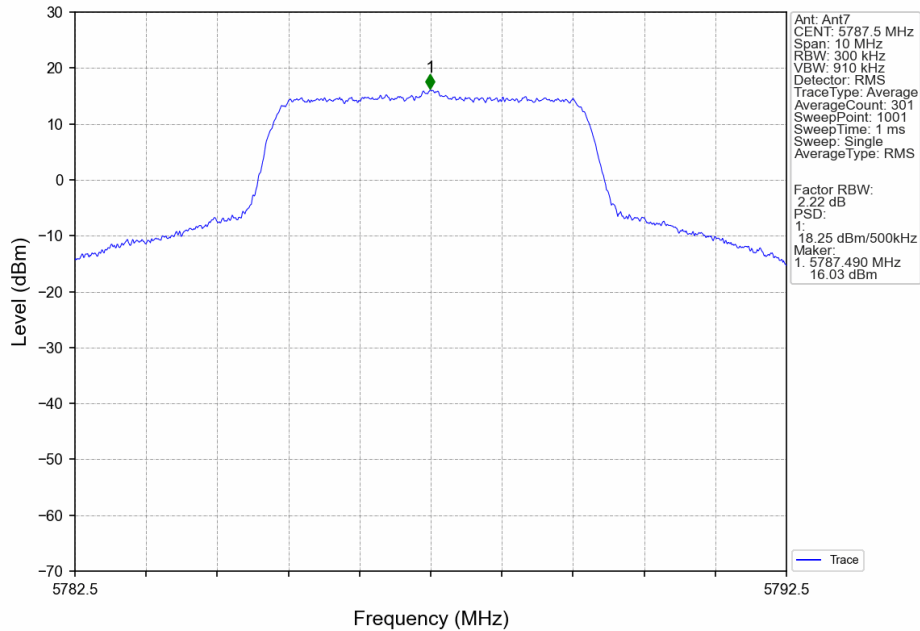
5M_MCH_5787.5MHz_MIMO_NTNV
