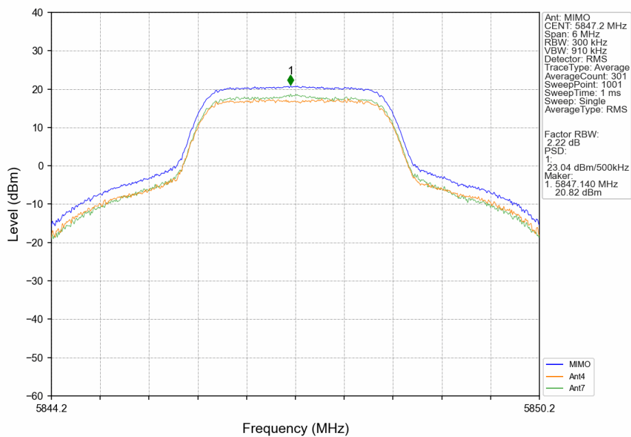
3M_HCH_5847.2MHz_MIMO_NTNV
