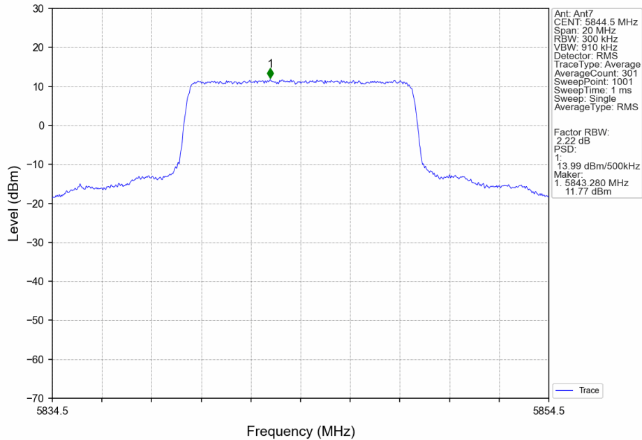
10M_HCH_5844.5MHz_MIMO_NTNV
