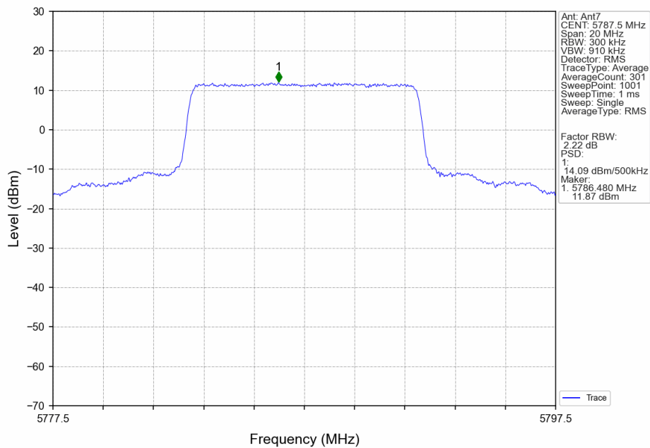
10M_MCH_5787.5MHz_Ant7_NTNV
