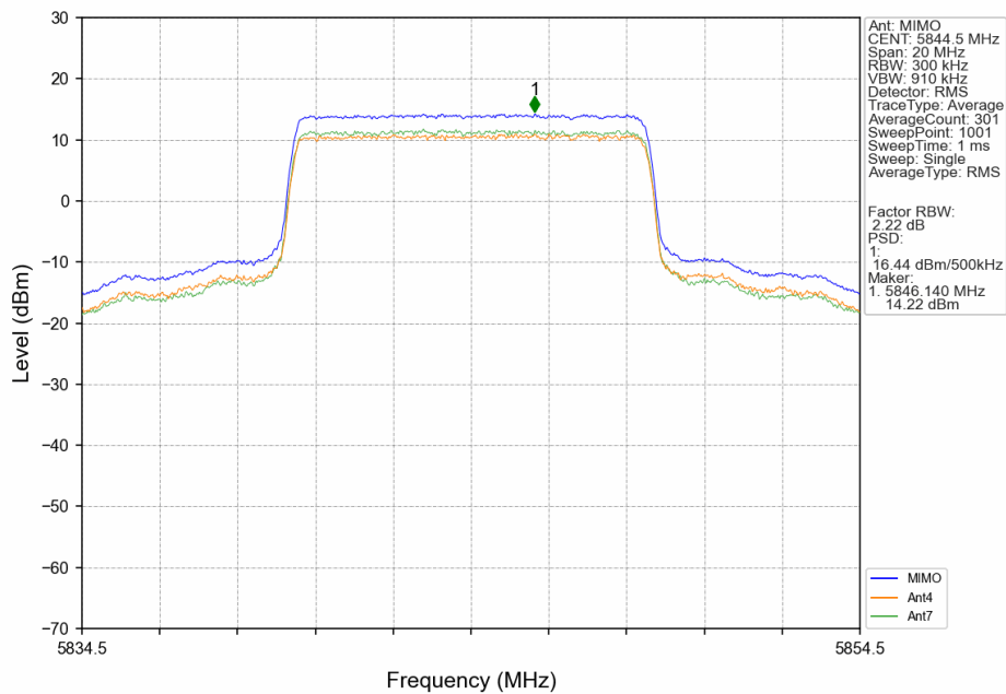
10M_HCH_5844.5MHz_MIMO_NTNV
