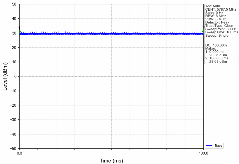
5M_MCH_5787.5MHz_Ant0_NTNV
