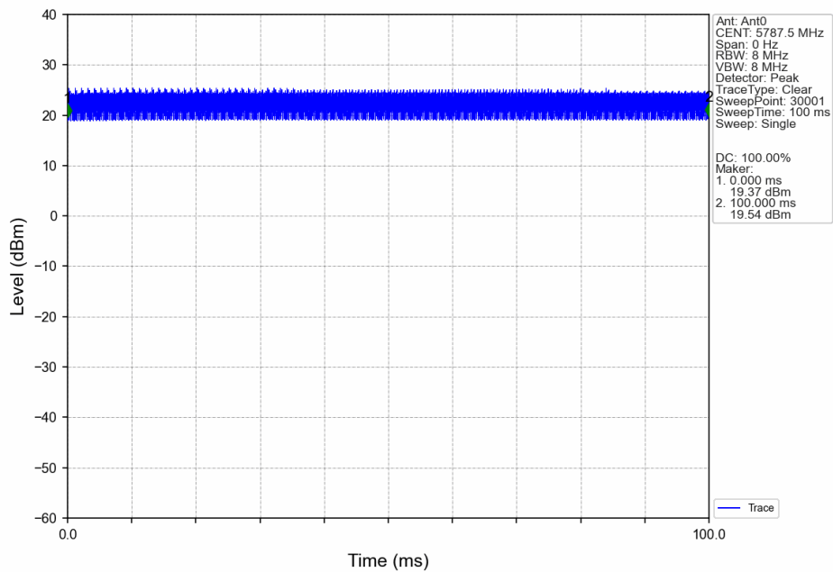
60M_MCH_5787.5MHz_Ant0_NTNV
