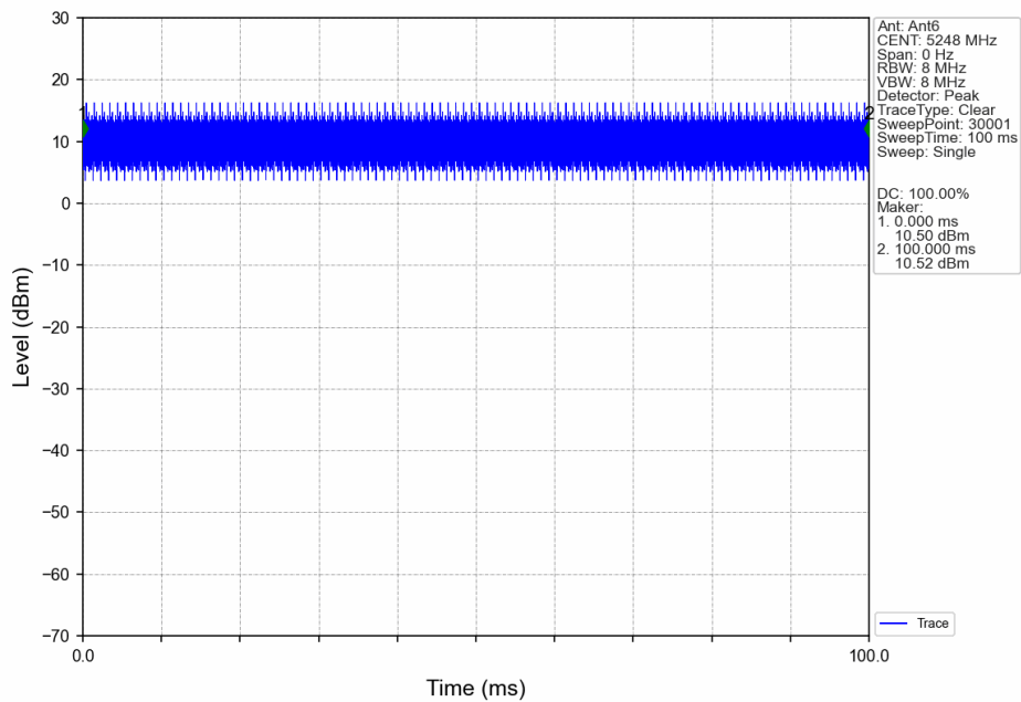
1.4M_HCH_5248MHz_Ant6_NTNV
