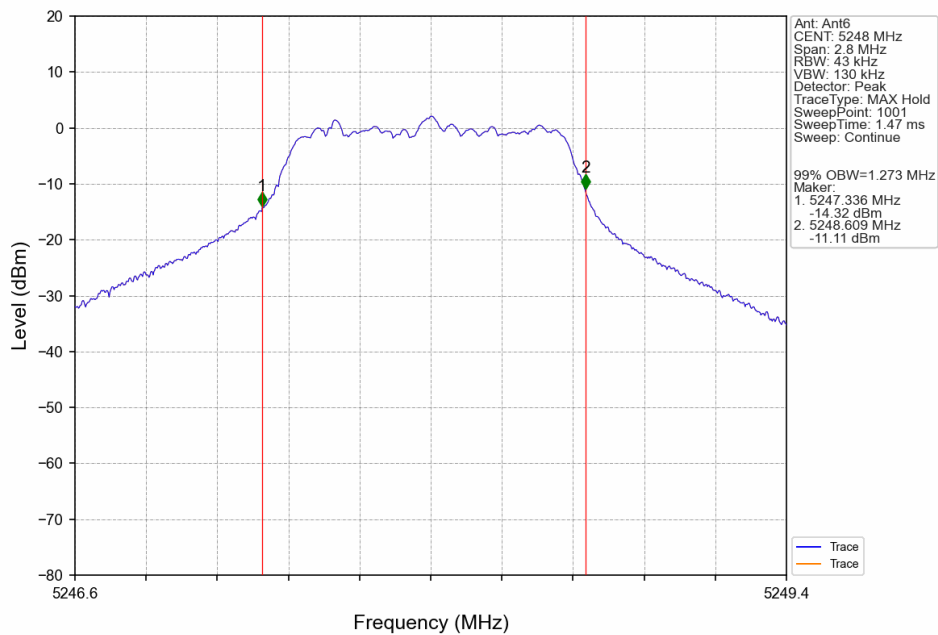
1.4M_HCH_5248MHz_Ant6_NTNV
