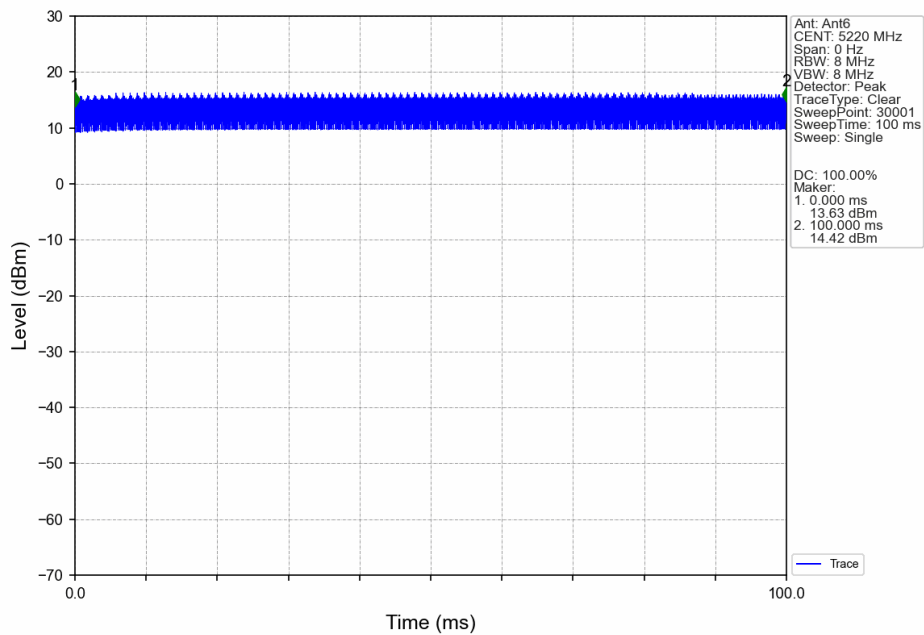
60M_HCH_5220MHz_Ant6_NTNV
