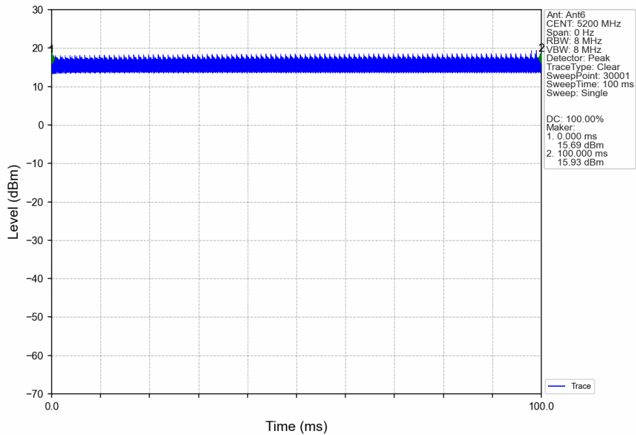
40M_MCH_5200MHz_Ant6_NTNV
