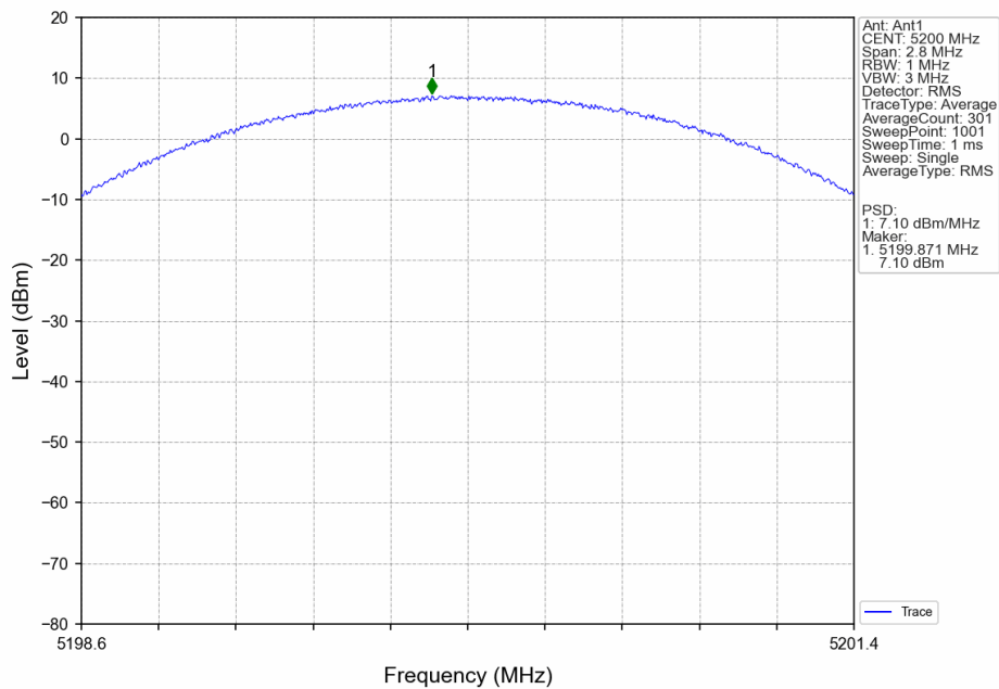
1.4M_MCH_5200MHz_Ant1_NTNV
