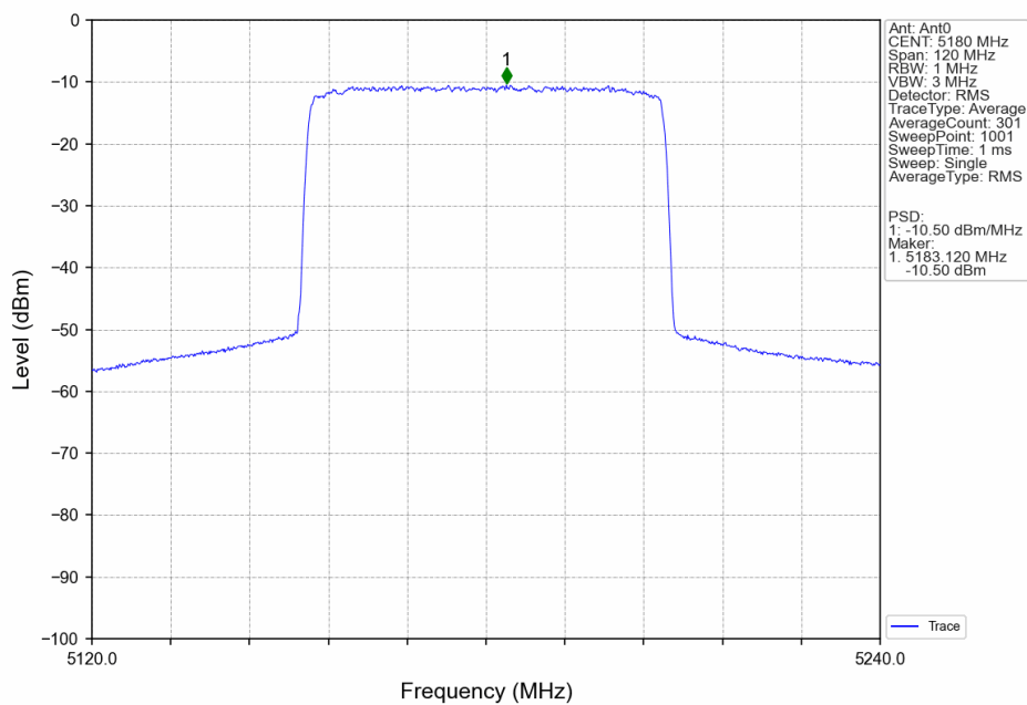
60M_LCH_5180MHz_Ant0_NTNV
