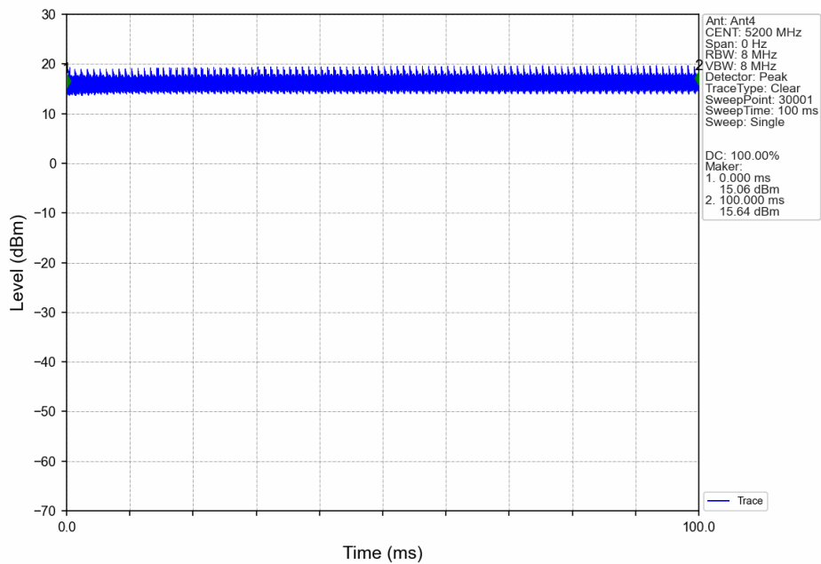
40M_MCH_5200MHz_Ant4_NTNV
