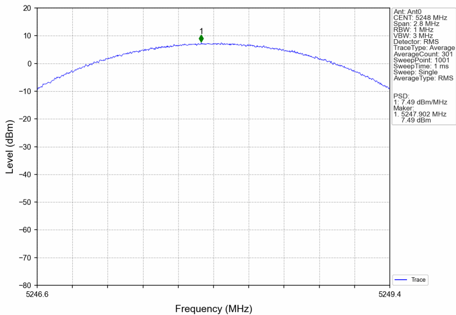
1.4M_HCH_5248MHz_Ant0_NTNV
