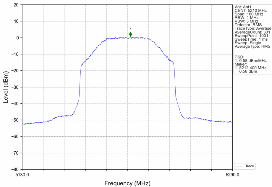
80M_HCH_5210MHz_Ant1_NTNV
