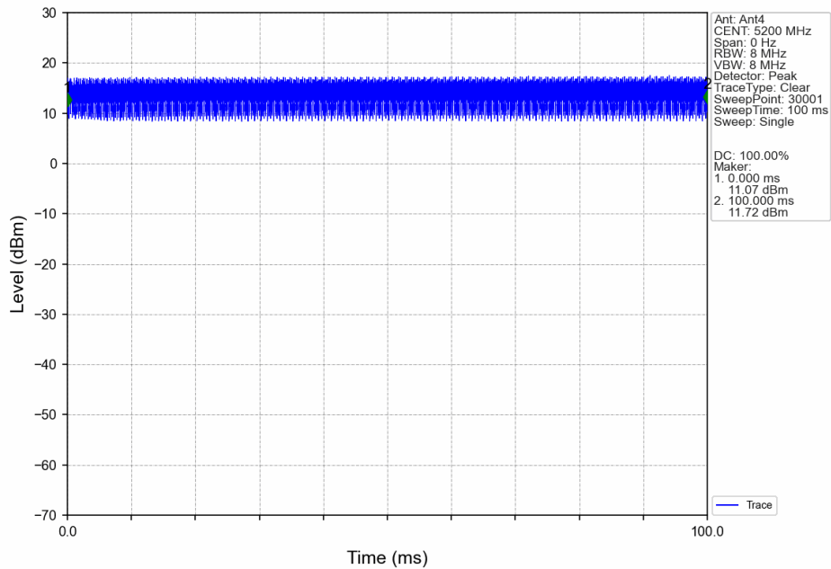
80M_MCH_5200MHz_Ant4_NTNV
