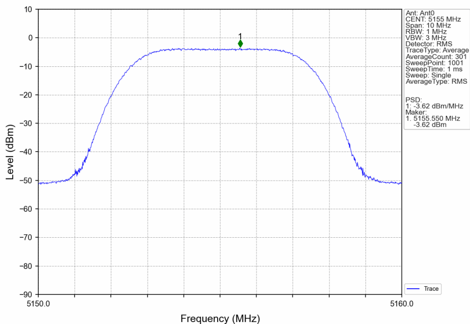
5M_LCH_5155MHz_Ant0_NTNV
