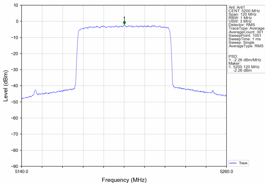
60M_MCH_5200MHz_Ant1_NTNV
