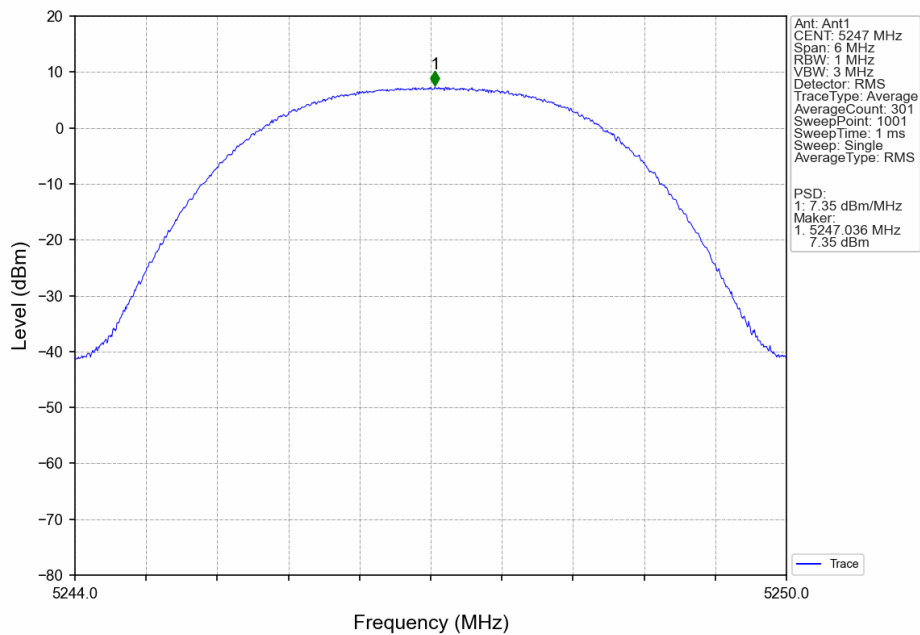
3M_HCH_5247MHz_Ant1_NTNV
