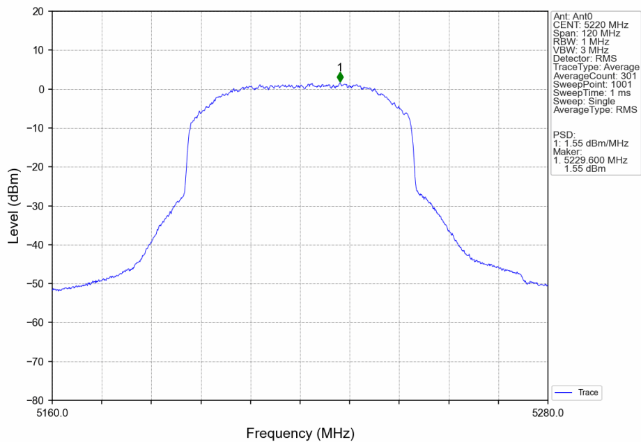
60M_HCH_5220MHz_Ant0_NTNV
