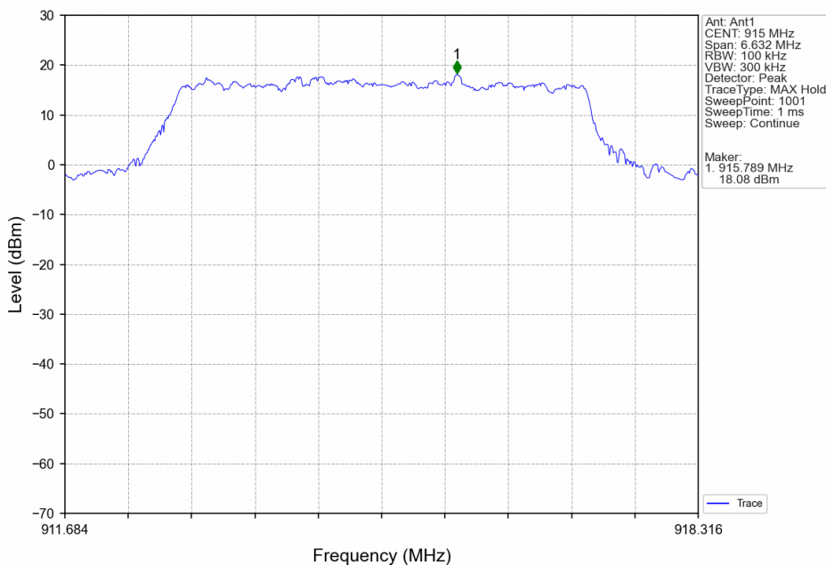
5M_MCH_915MHz_Ant1_NTNV
