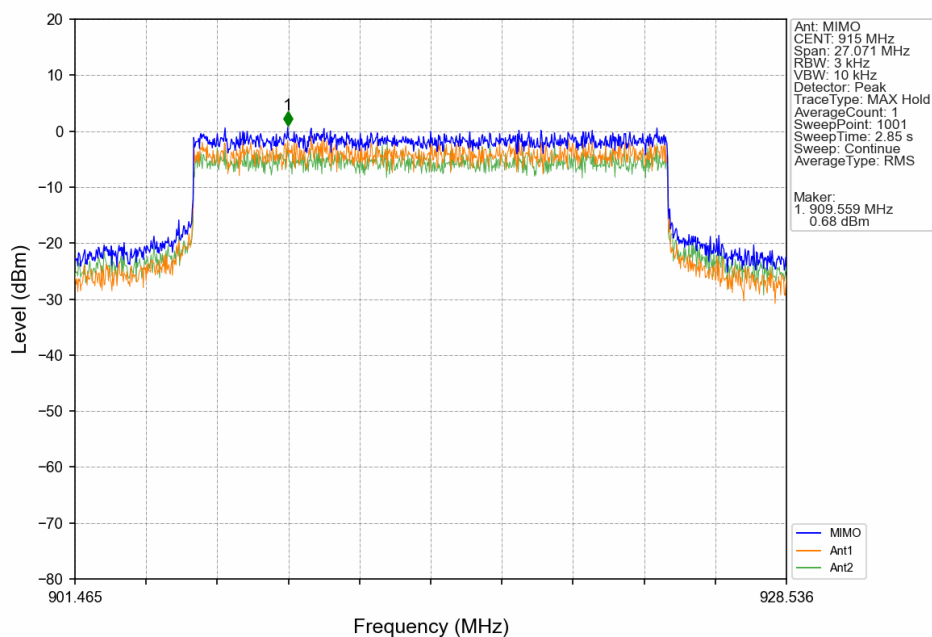
20M_MCH_915MHz_MIMO_NTNV
