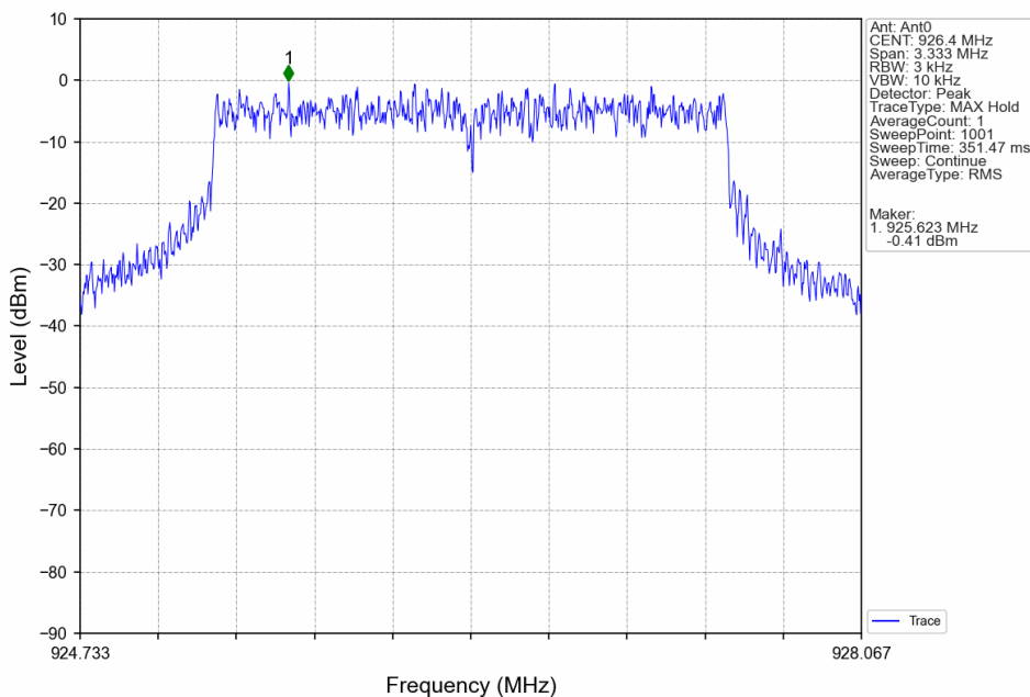
3M_HCH_926.4MHz_Ant0_NTNV
