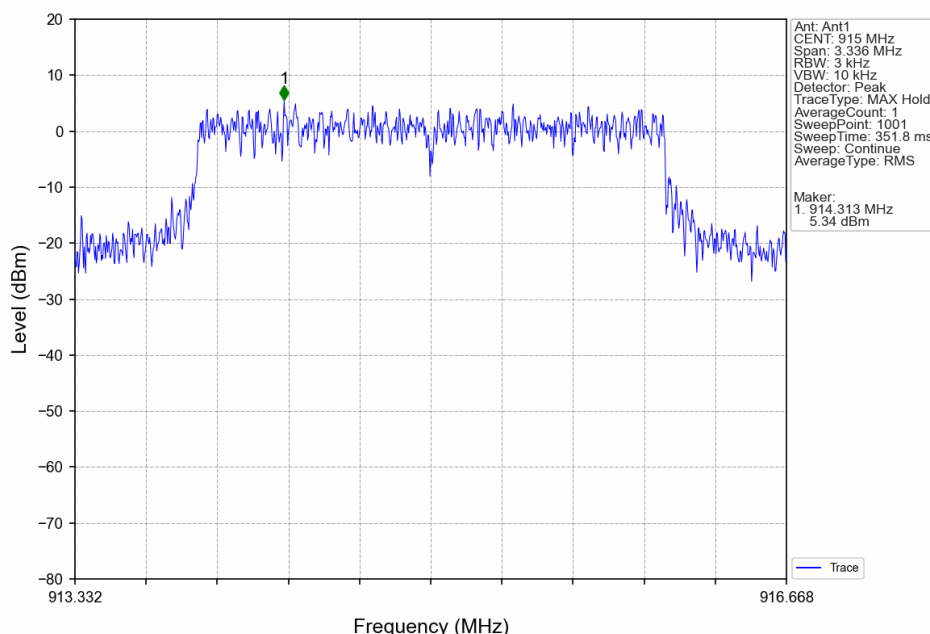
3M_MCH_915MHz_Ant1_NTNV
