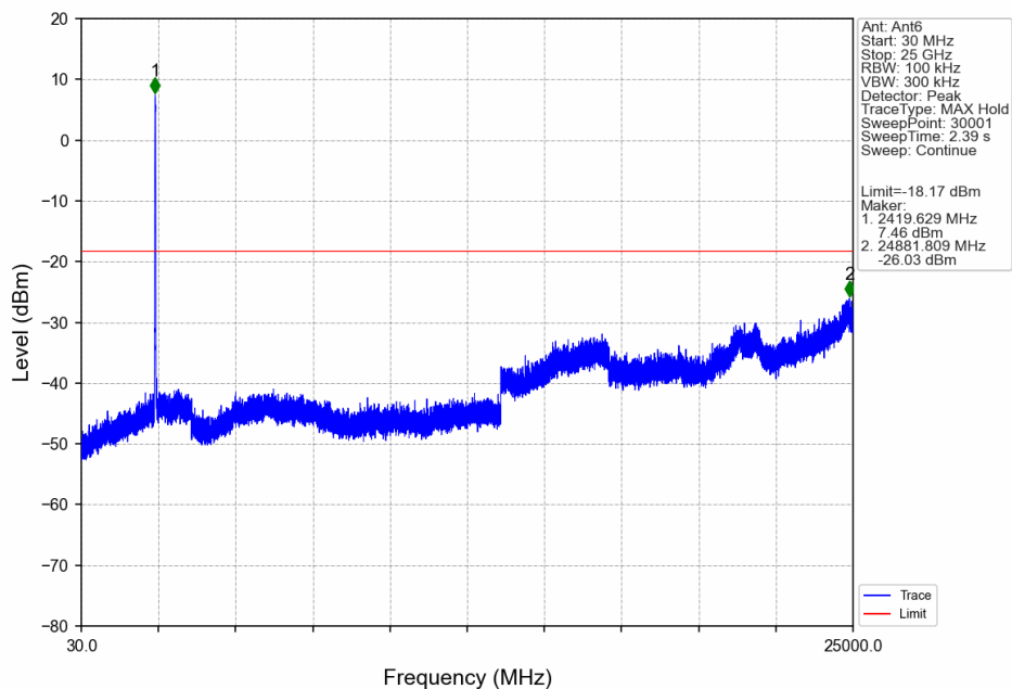
40M_LCH_2422.5MHz_Ant6_NTNV
