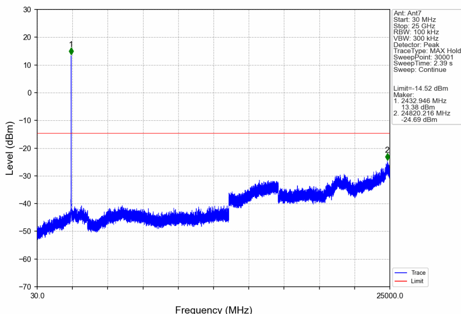
10M_MCH_2437.5MHz_Ant7_NTNV
