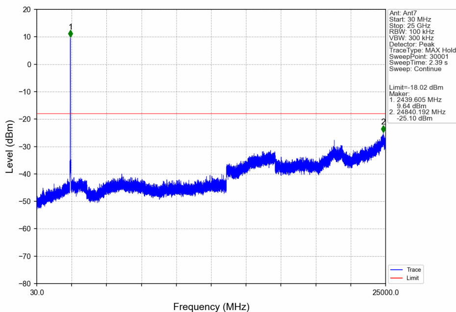
40M_MCH_2437.5MHz_Ant7_NTNV
