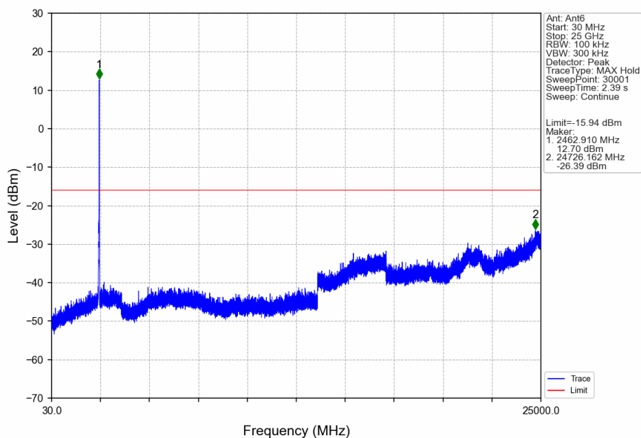
20M_HCH_2462.5MHz_Ant6_NTNV
