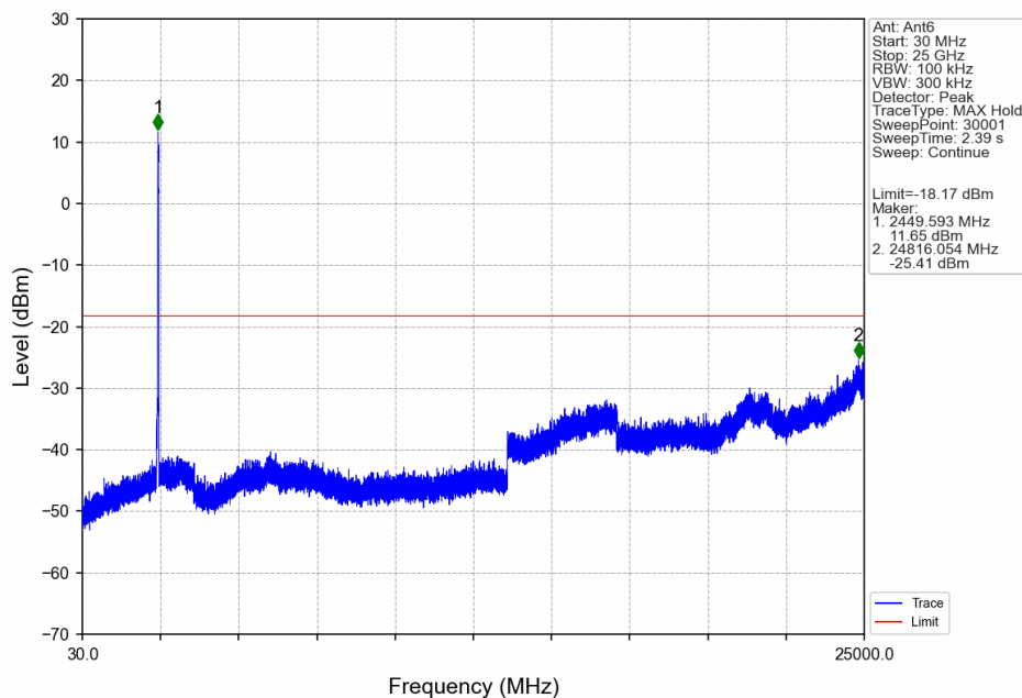
40M_HCH_2452.5MHz_Ant6_NTNV
