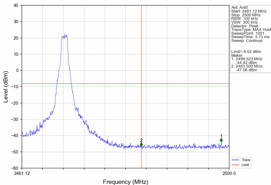
1.4M_HCH_2469.12MHz_Ant0_NTNV
