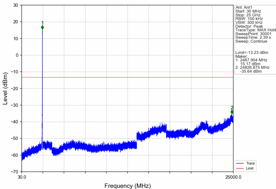
10M_HCH_2467.5MHz_Ant1_NTNV
