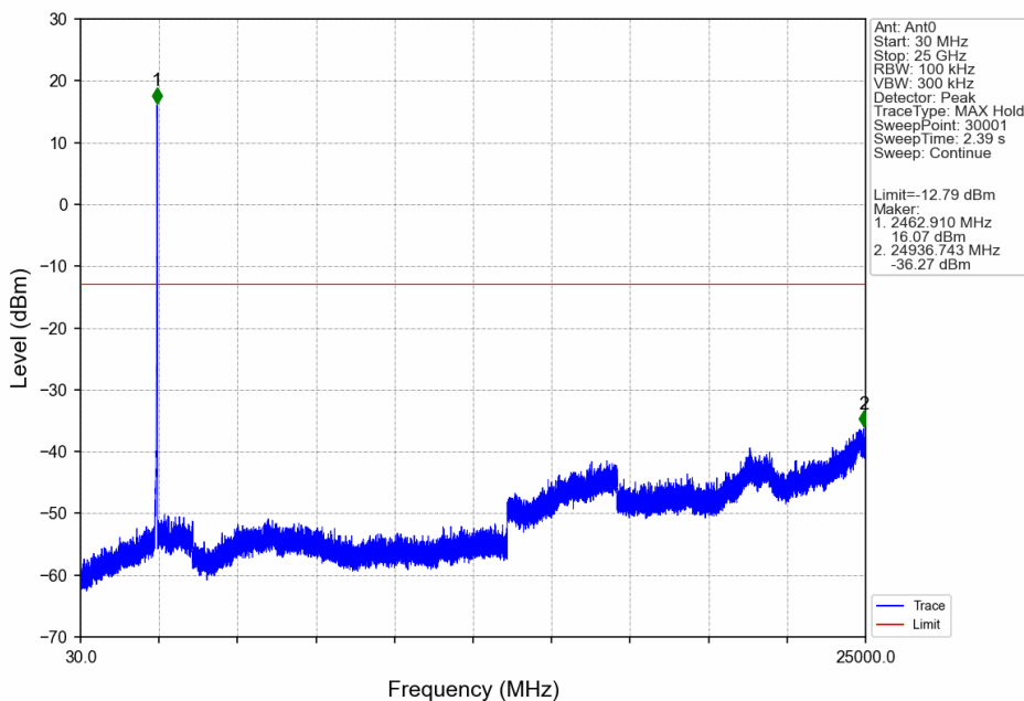
10M_HCH_2467.5MHz_Ant0_NTNV
