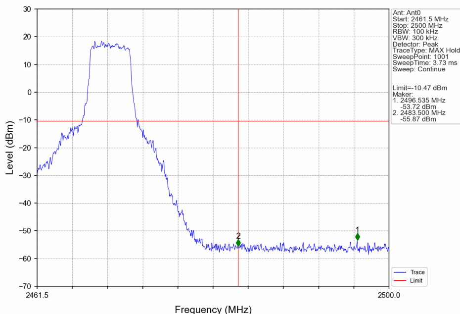
5M_HCH_2469.5MHz_Ant0_NTNV
