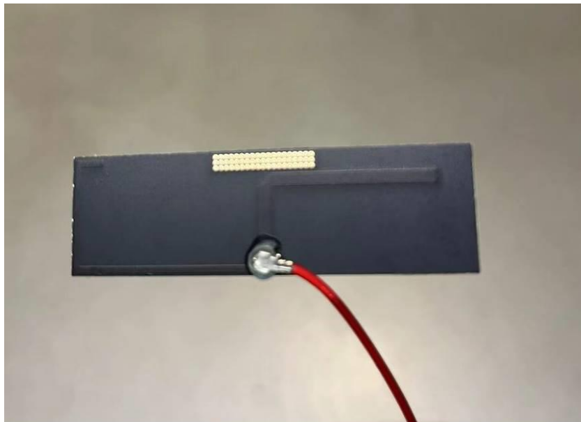
SDR ANT0
