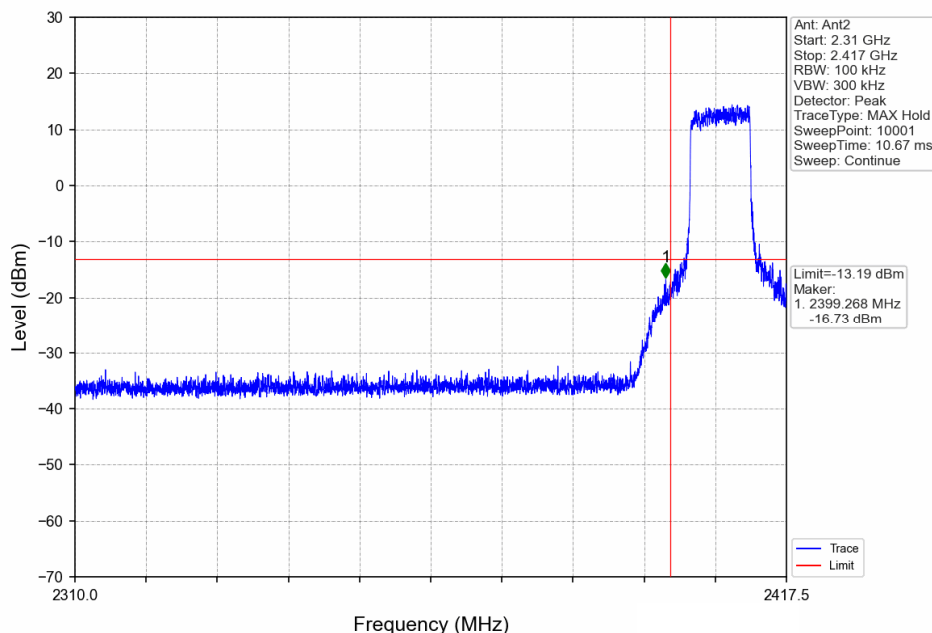
10MHz BW_LCH_2407.5MHz_Ant2_NTNV
