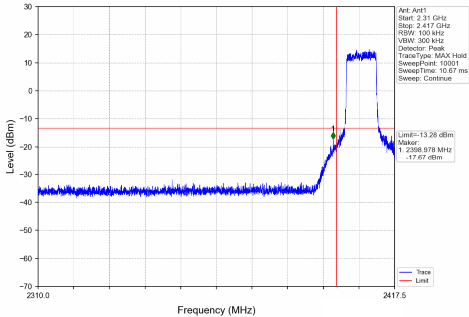
10MHz BW_LCH_2407.5MHz_Ant1_NTNV
