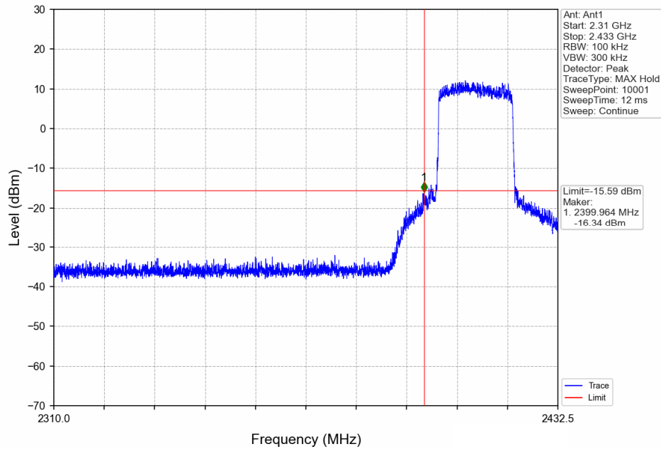
20MHz BW_LCH_2412.5MHz_Ant1_NTNV
