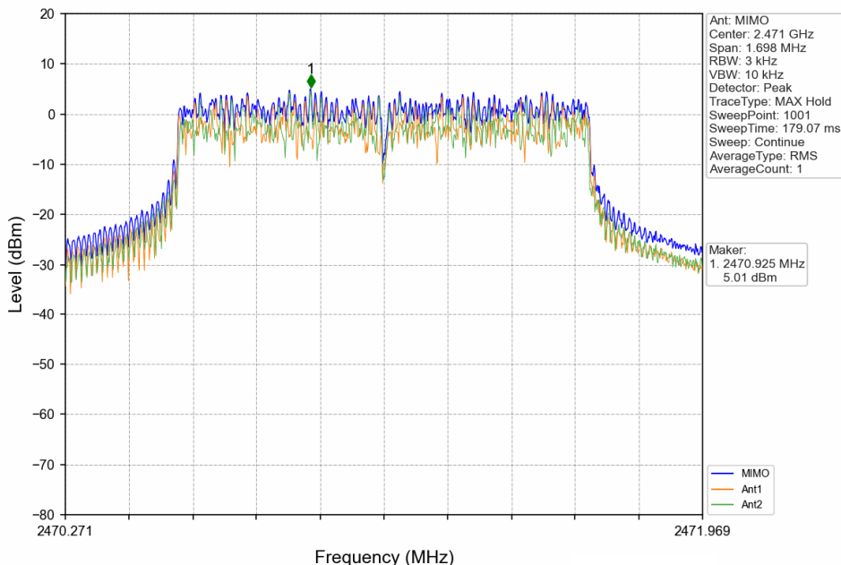
1.4MHz CA BW_HCH_2471.12MHz_MIMO_NTNV
