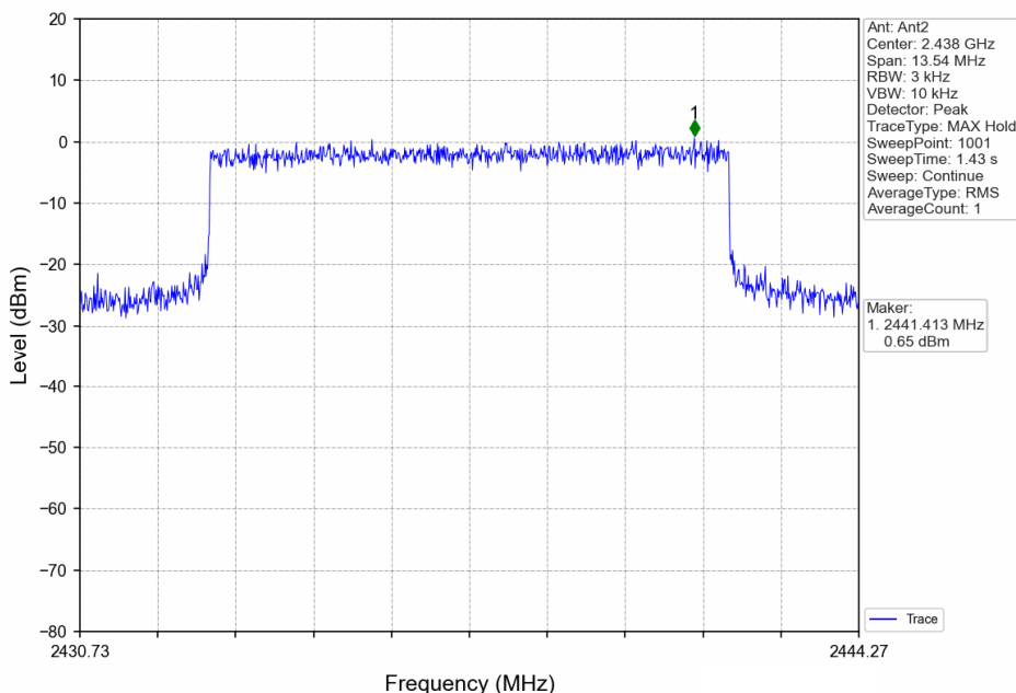
10MHz BW_MCH_2437.5MHz_MIMO_NTNV
