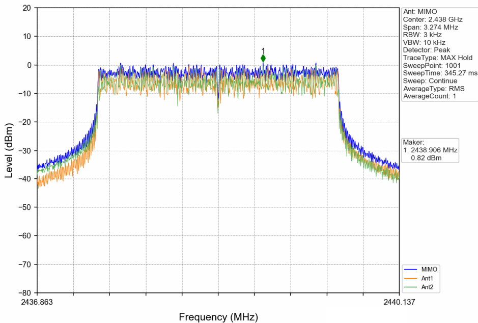
3MHz BW_MCH_2438.5MHz_MIMO_NTNV
