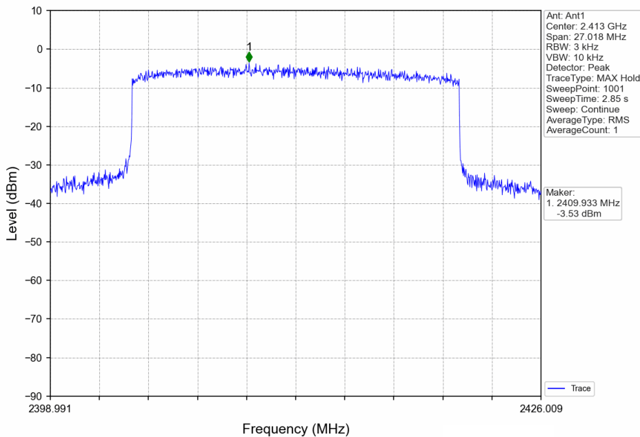
20MHz BW_LCH_2412.5MHz_Ant1_NTNV
