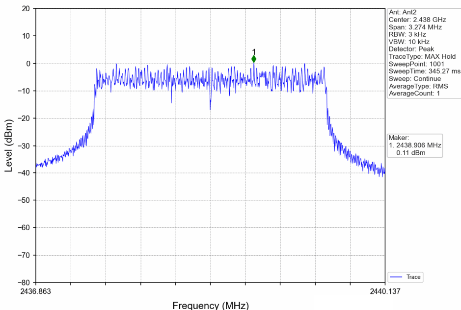
3MHz BW_MCH_2438.5MHz_MIMO_NTNV
