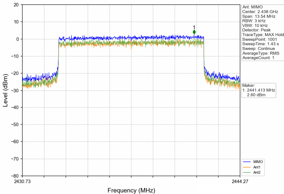
10MHz BW_MCH_2437.5MHz_MIMO_NTNV
