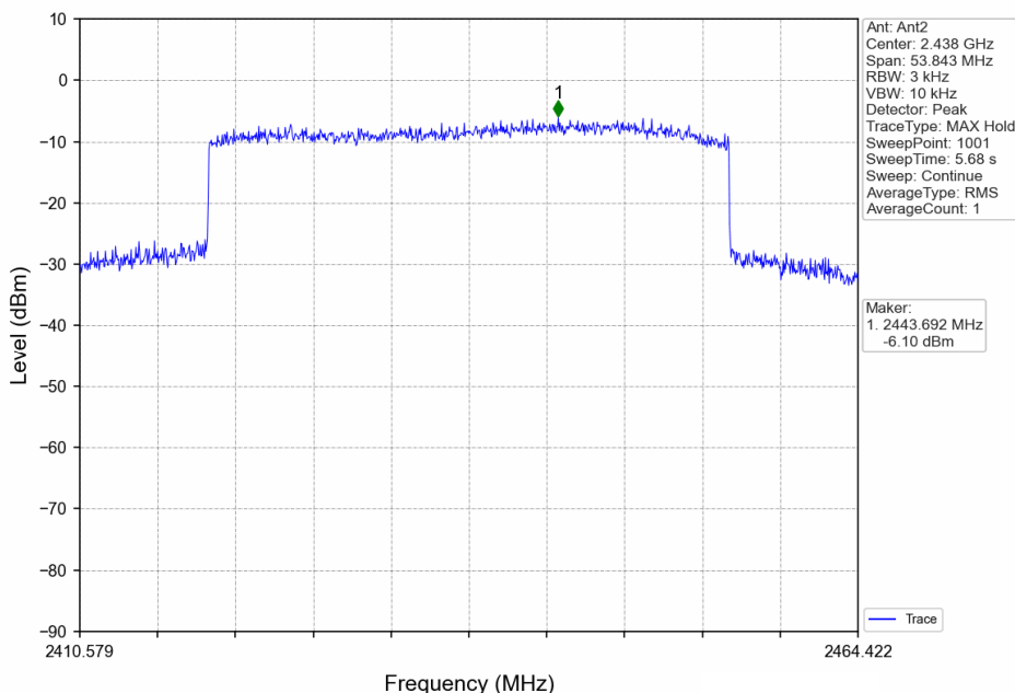
40MHz BW_MCH_2437.5MHz_MIMO_NTNV
