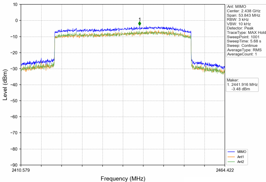
40MHz BW_MCH_2437.5MHz_MIMO_NTNV
